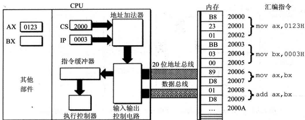
图 2.20 CS:2000H, IP:0003H(CPU 将从内存 2000H×16+0003H 处读取指令 BB 03 00)
