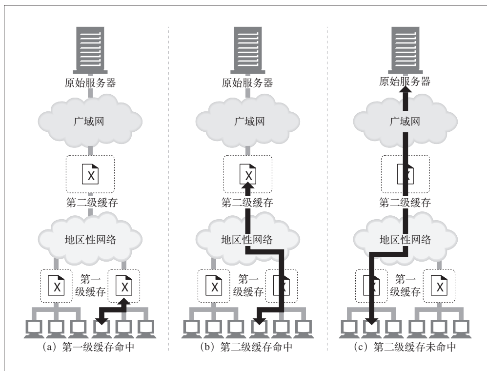
图 7-9 在两级的缓存层次结构中访问文档
