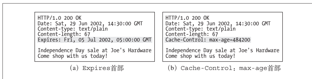
图 7-13 Expires 首部和 Cache-Control 首部
