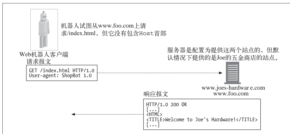
图 9-5 发送请求时没有携带 Host 首部，虚拟 docroot 会引发问题的例子
