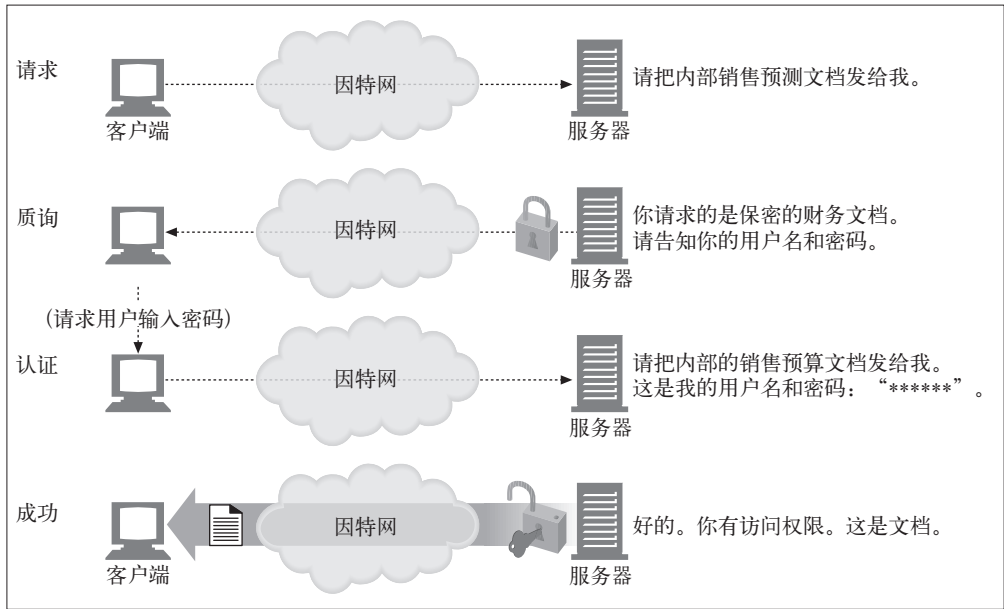
图 12-1 简化的质询 / 响应认证框架
