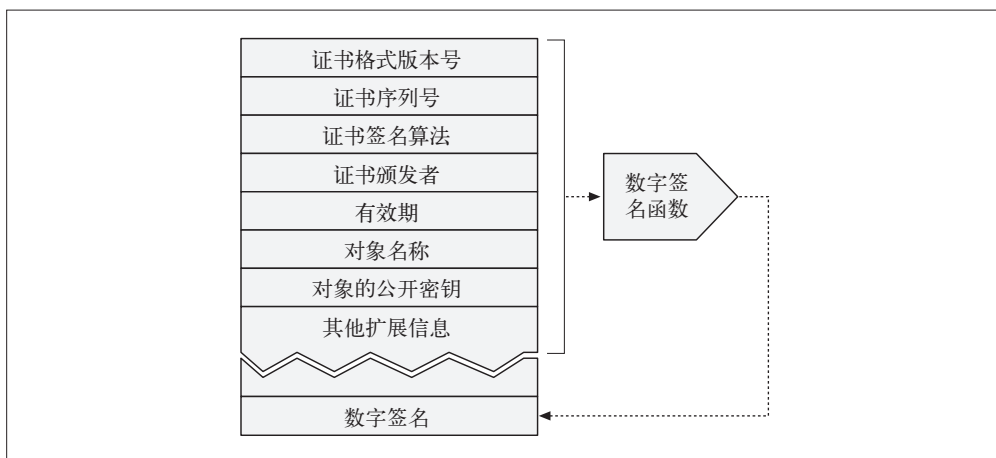
图 14-11 典型的数字签名格式
