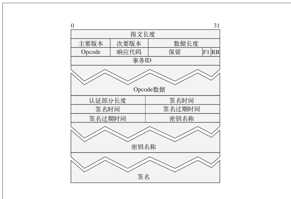
图 20-15 HTCP 报文格式
