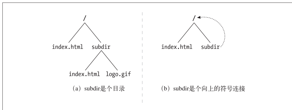
图 9-3 符号连接环路
