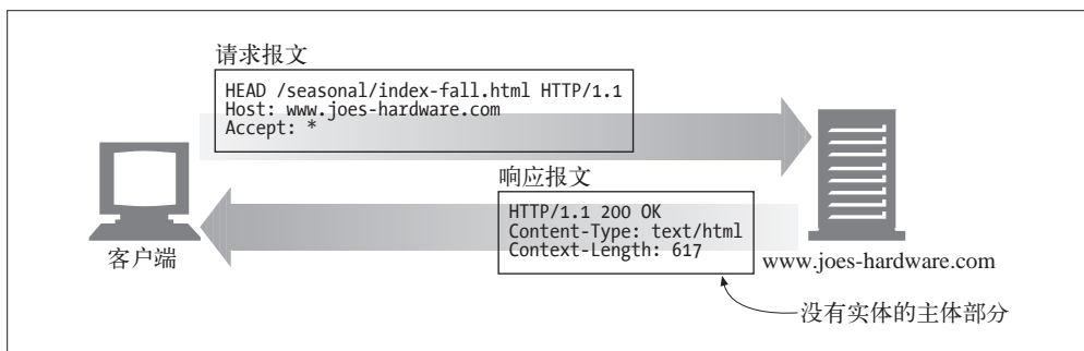
图 3-8 HEAD 示例
