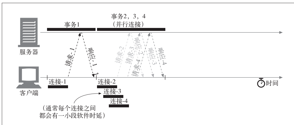
图 4-12 4 个事务（并行）
