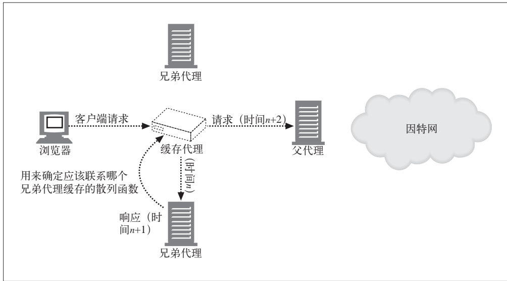
图 20-14 CARP 重定向
