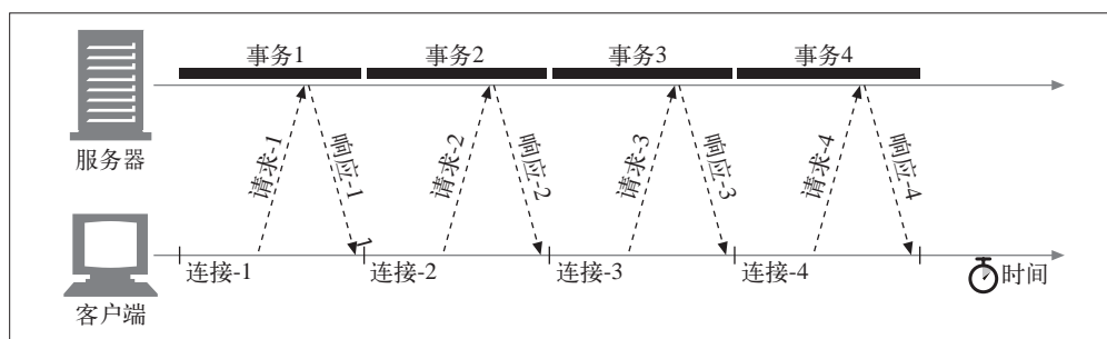
图 4-10 4 个事务（串行）
