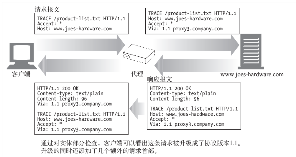
图 3-11 TRACE 示例
