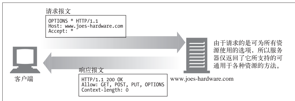
图 3-12 OPTIONS 示例
