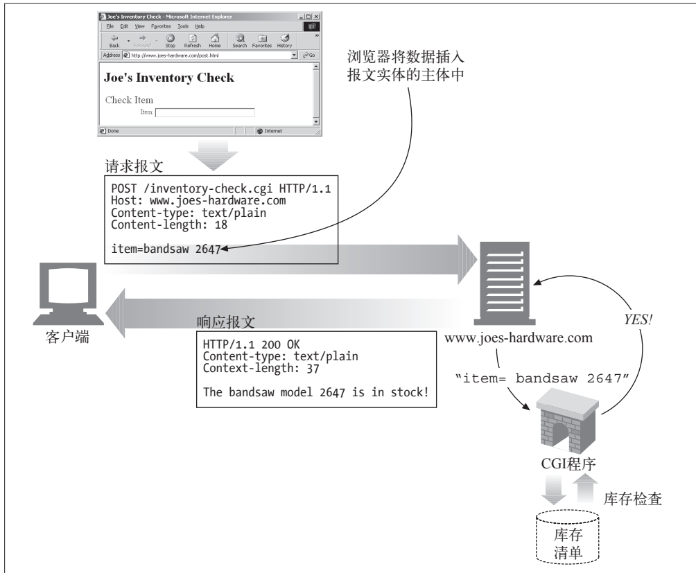
图 3-10 POST 示例
