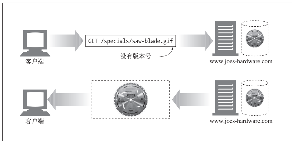
图 3-6 HTTP/0.9 事务
