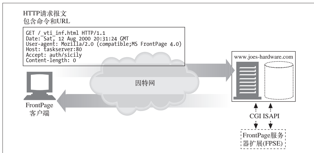
图 19-2 初始请求
