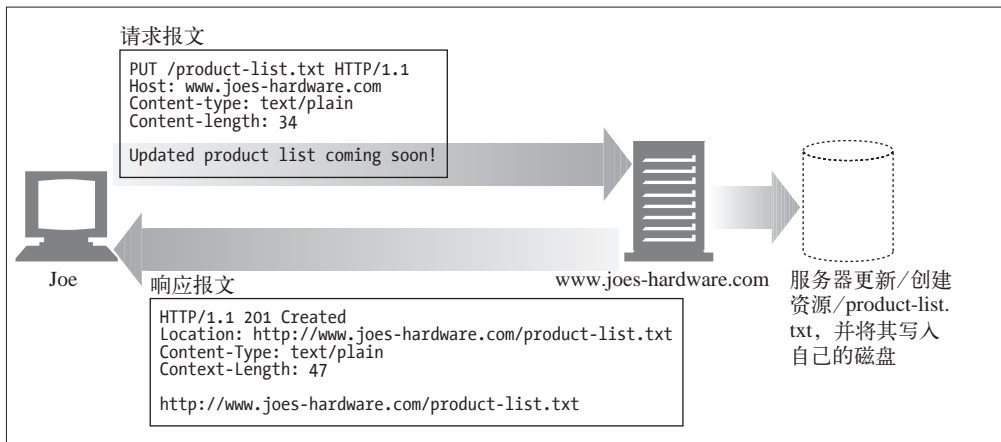
图 3-9 PUT 示例
