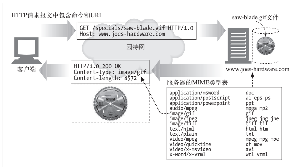
125 图 5-12 Web 服务器用 MIME 类型文件来设置资源输出的 Content-type 首部
