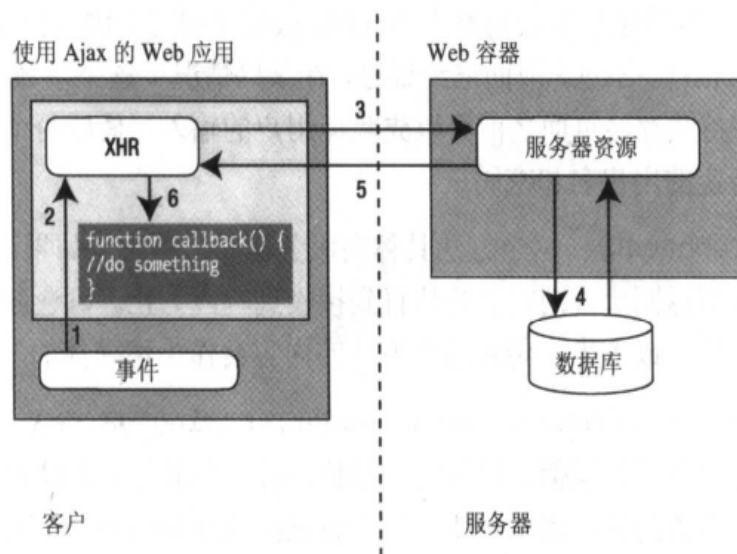
图 2-1 标准 Ajax 交互
