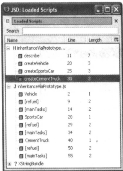
图 7-11 Loaded Scripts 窗口显示当前浏览器窗口中的所有可用脚本
