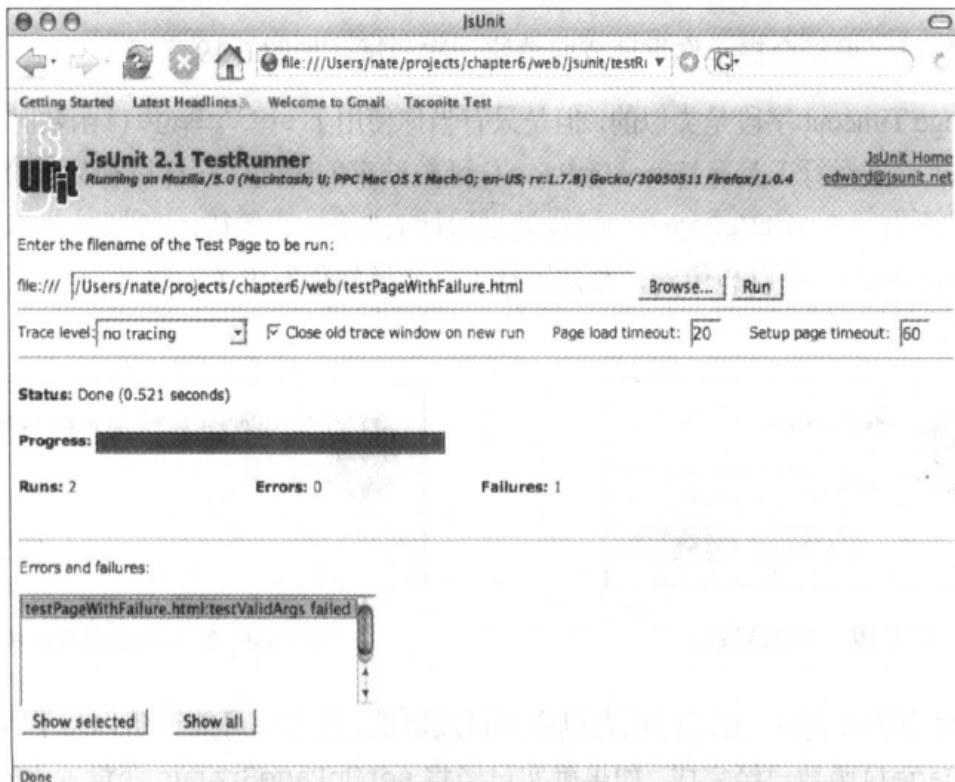
图 6-16 JsUnit 测试运行工具失败
