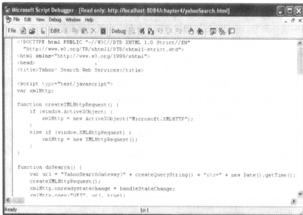
图 7-6 Microsoft Script Debugger 显示当前 HTML 页面
