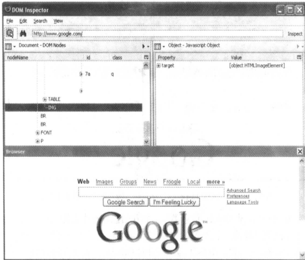
图 5-9 使用 DOM Inspector 移动 Google 搜索页面主图片的结果
