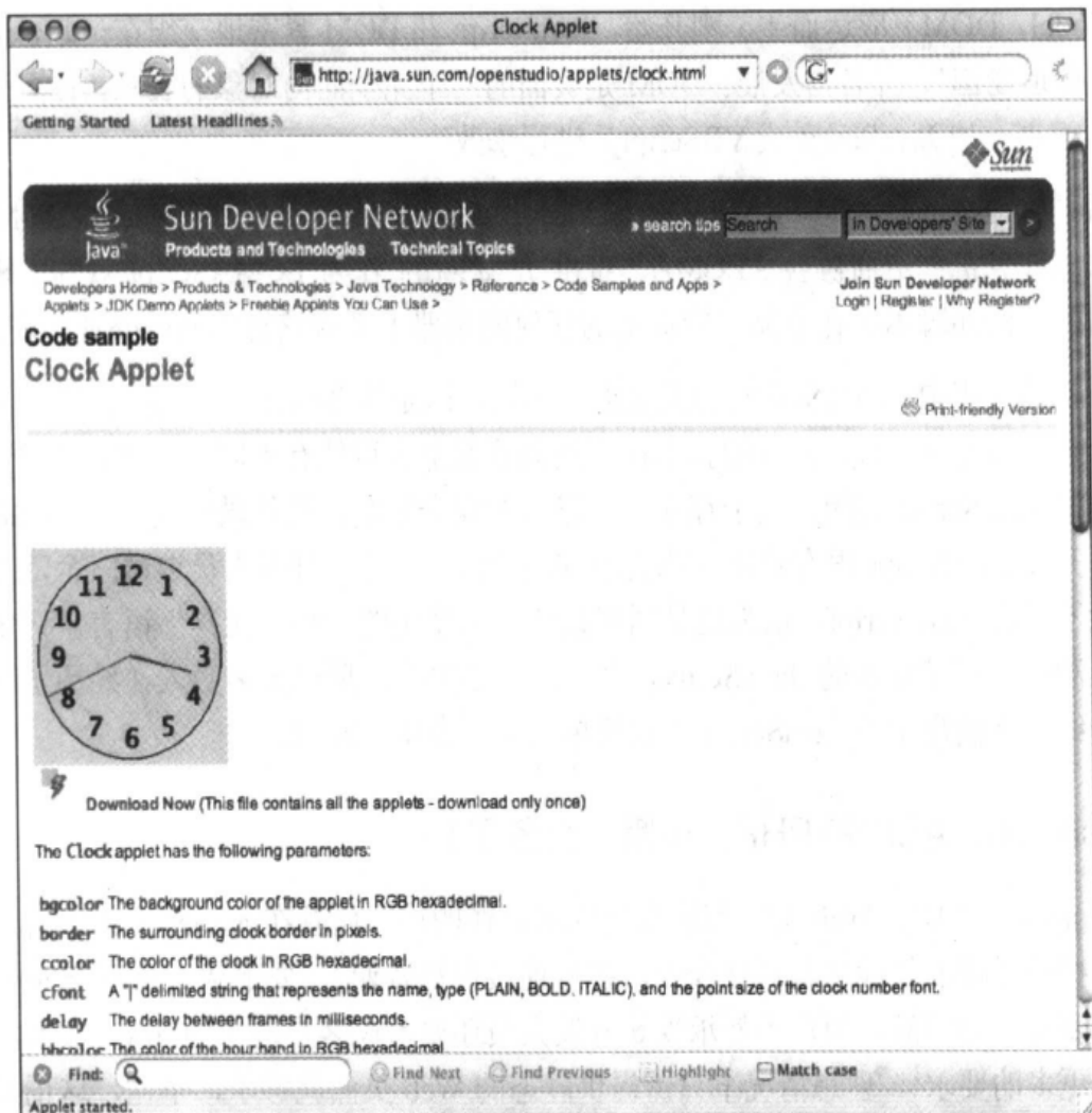
图 1-1 Sun 的时钟 applet
