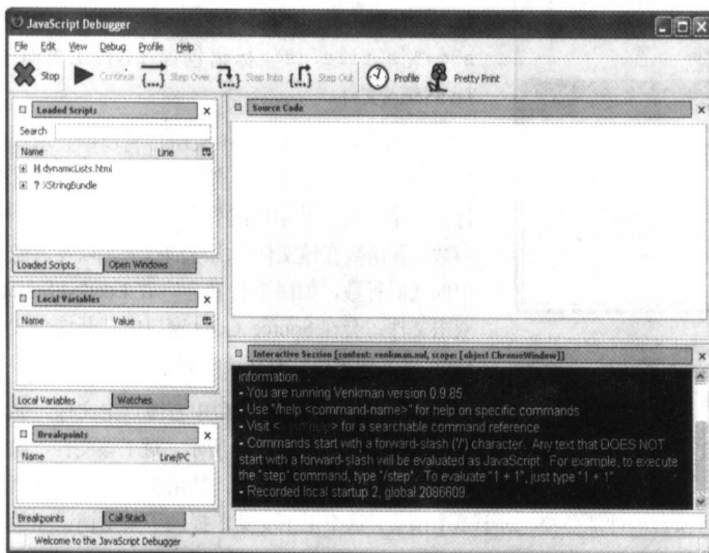
图 7-9 Venkman 的默认窗口布局
