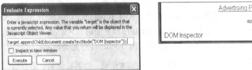
图 5-11 使用 JavaScript 计算窗口在页面的体中动态增加一个文本节点(左图), 以及浏览器窗格中的结果(右图)
