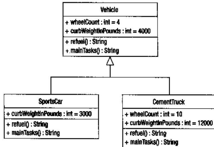
图 5-15 Vehicle、SportsCar 和 CementTruck 对象之间的关系
