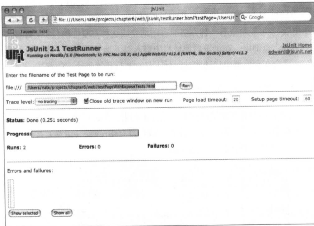
图 6-22 使用带 autoRun 的 testPage 的例子
