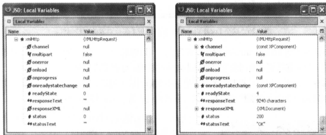
图 7-25 刚创建的 XMLHttpRequest 对象（左）和做出成功请求之后的 XMLHttpRequest 对象（右）
