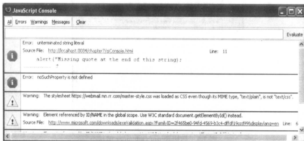
图 7-4 Firefox JavaScript Console 描述错误及错误在源文件中的位置
