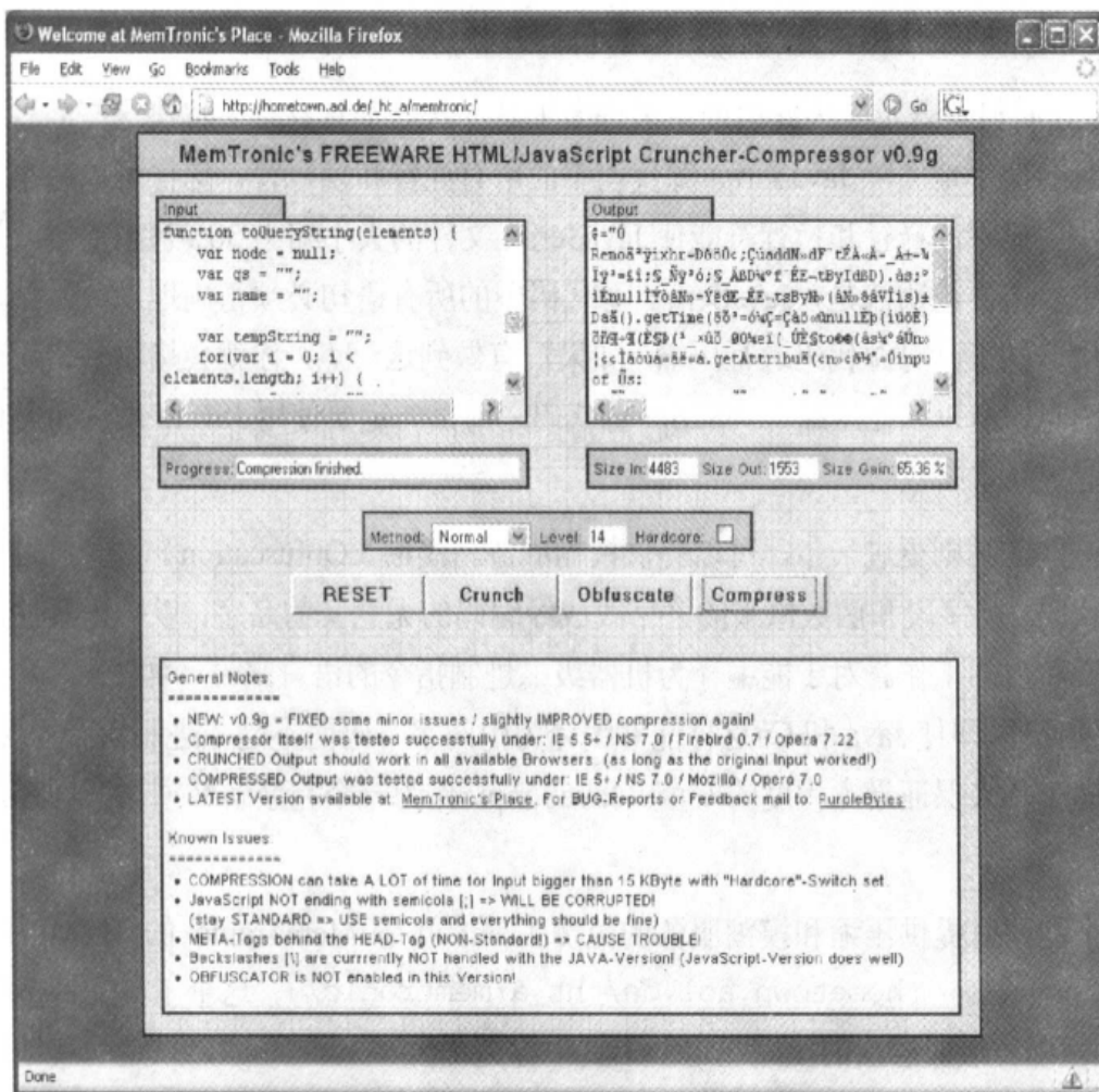
图 5-13 MemTronic 的 HTML/JavaScript Cruncher-Compressor 可以大大缩小 JavaScript 源代码的大小，并且难于读懂
