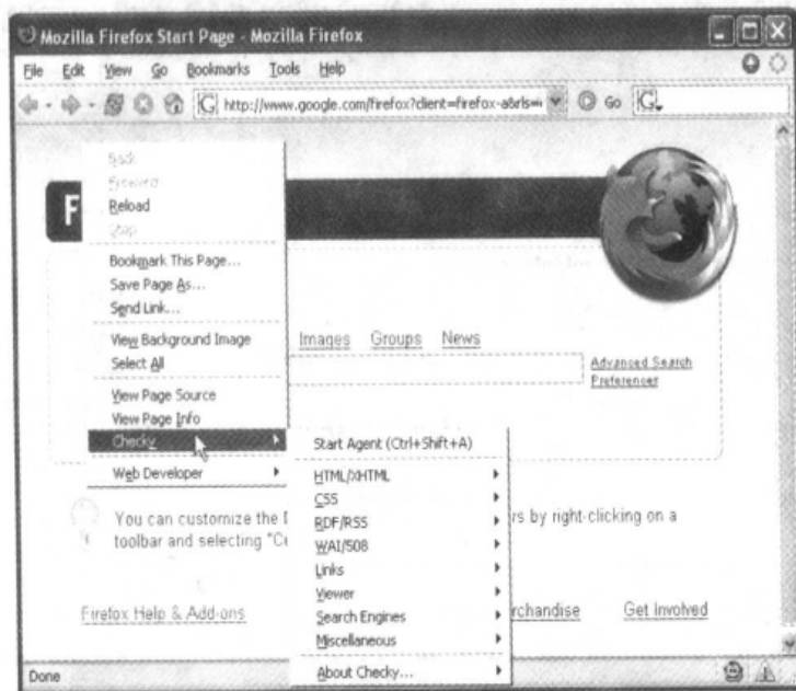
图 5-5 可以在 Firefox 中通过上下文菜单来访问 Checky
