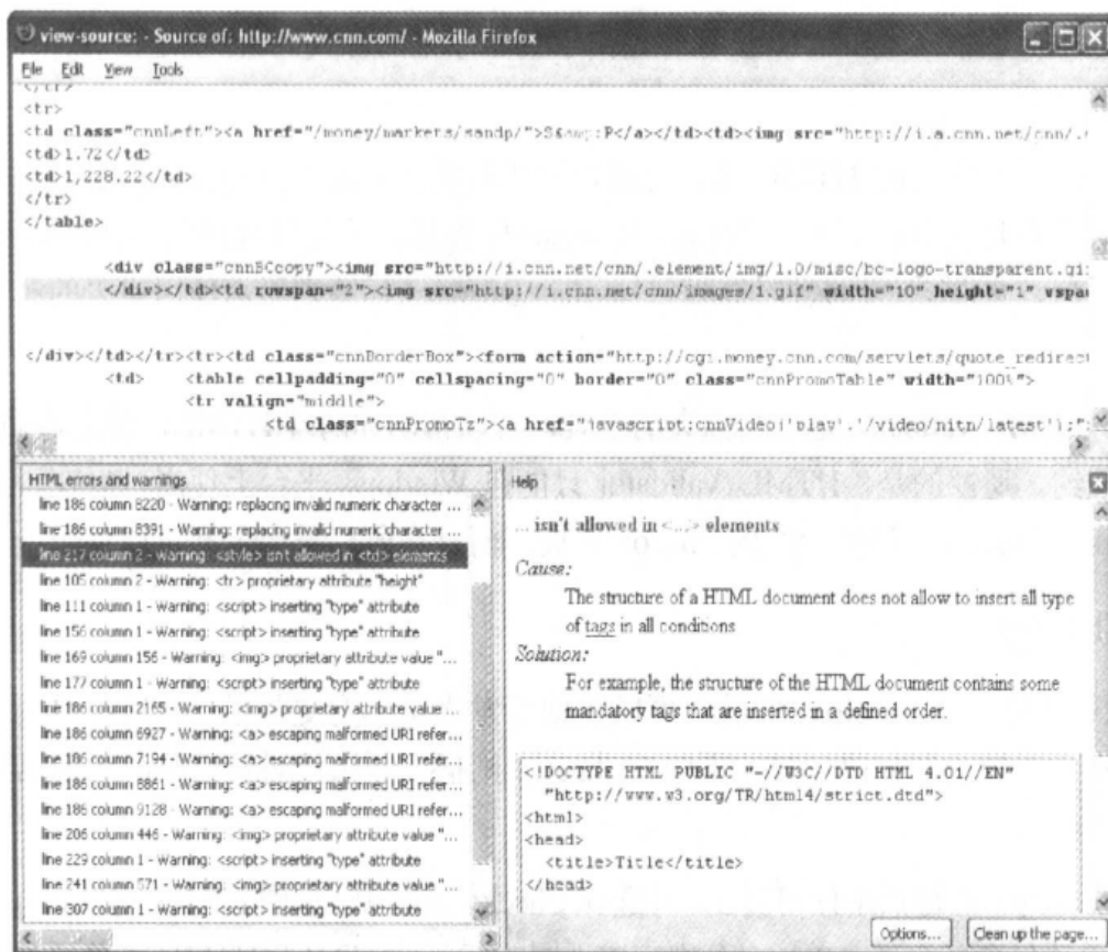
图 5-3 当查看页面的源代码时，HTML Validator 会列出 HTML 源代码中的错误，并提出修正问题的建议
