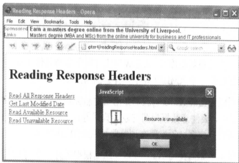
图 4-5 确定 Web 资源是否可用
