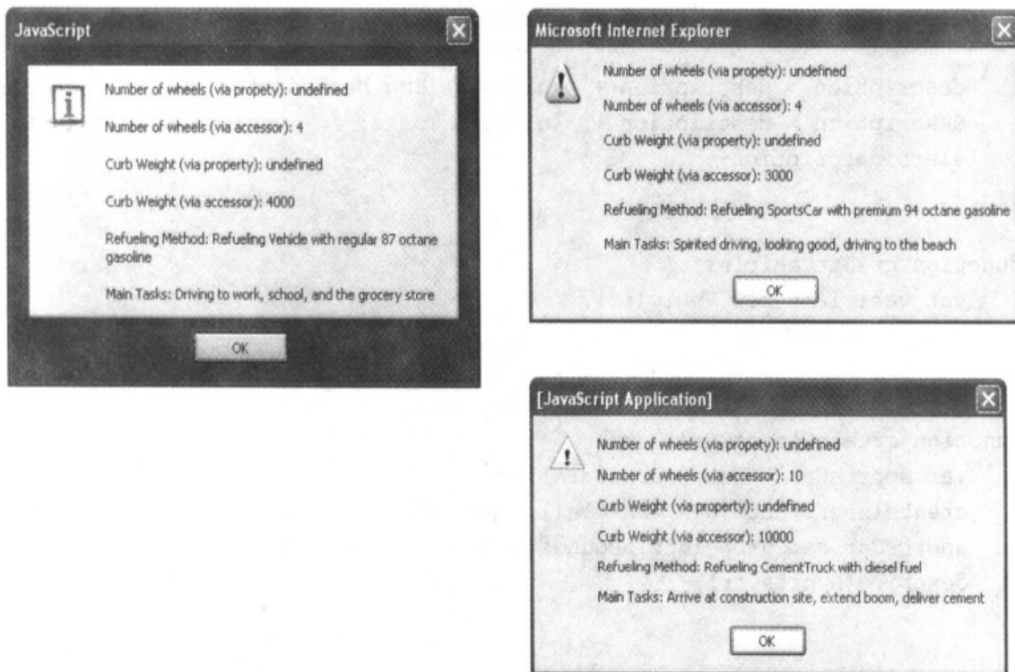
图 5-17 创建 Vehicle、SportsCar 和 CementTruck 对象, 并使用 describe 函数描述它们的结果。私有属性不能直接访问, 见警告框中的 undefined 值
