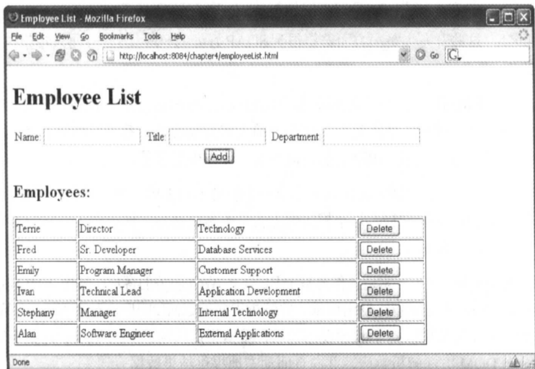
图 4-14 每次点击 Add 按钮时每个姓名动态增加到列表中，而不必每次都刷新页面
