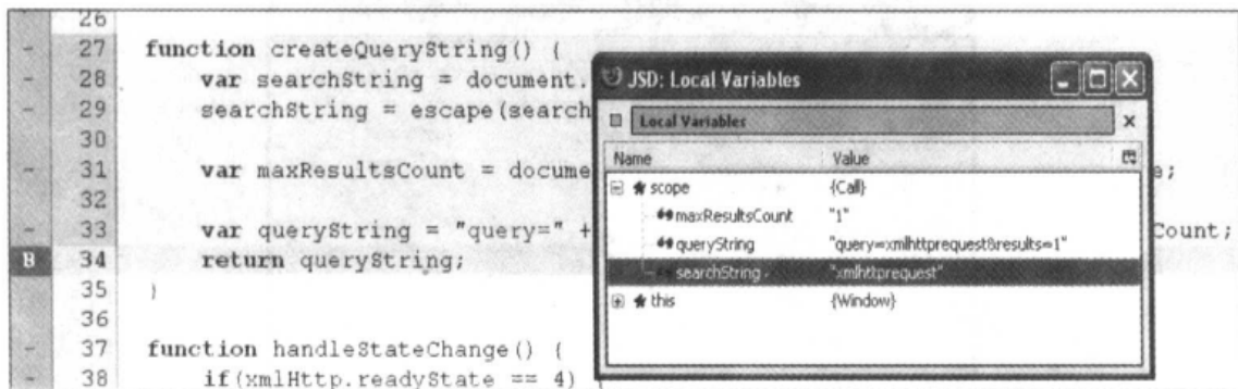
图 7-22 当前作用域中的所有变量
