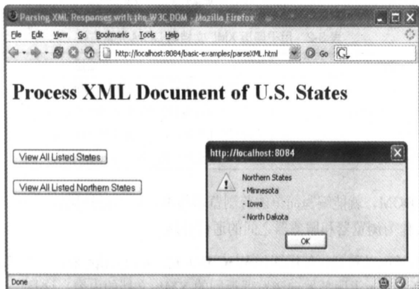
图 3-2 点击页面上的任何一个按钮都会从服务器加载 XML 文档，并在警告框中显示适当的结果
