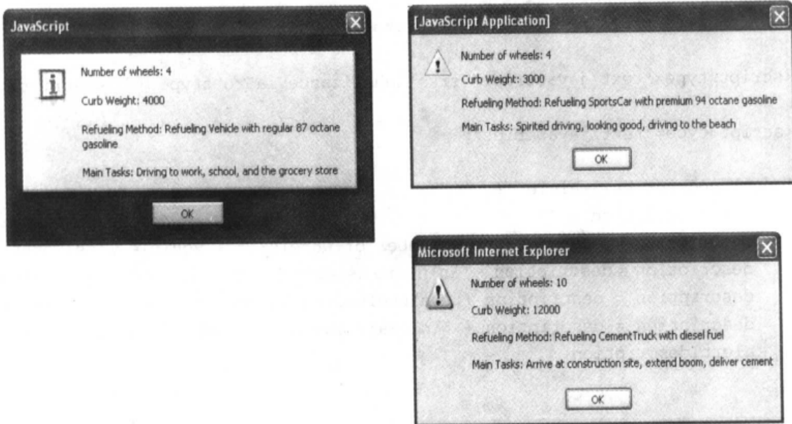
图 5-16 创建 Vehicle、SportsCar 和 CementTruck 对象并使用 describe 函数分别描述的结果
