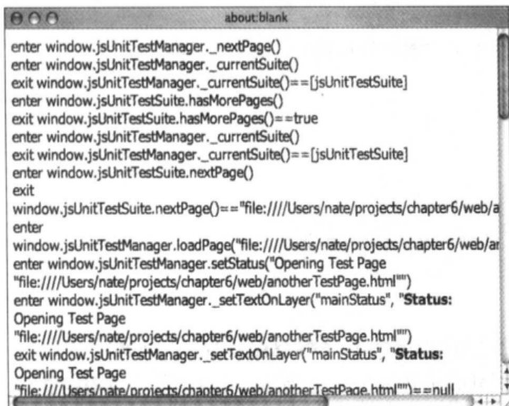
图 6-24 debug 查询的输出
