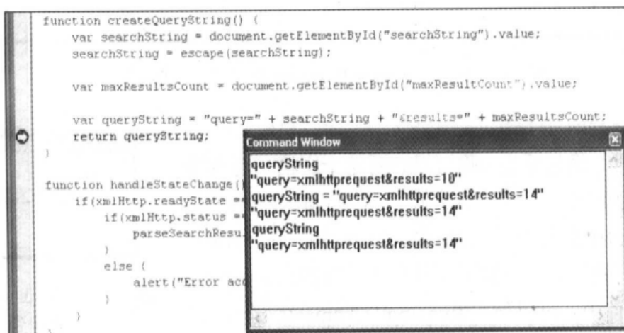
图 7-8 使用命令窗口检查和修改变量值
