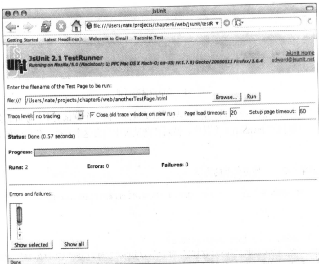
图 6-2 采用典型方法的结果
