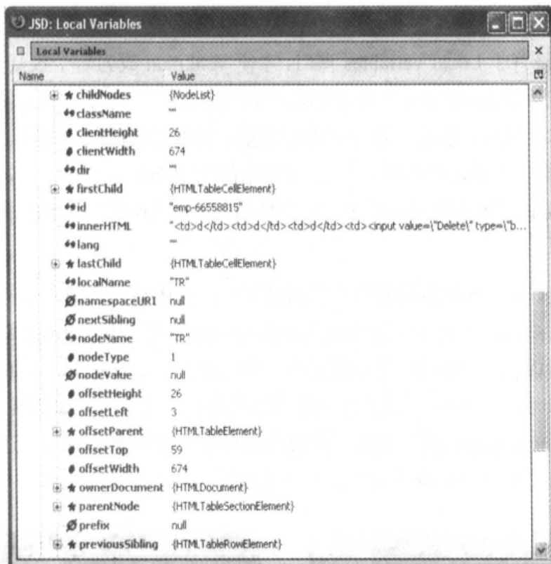
图 7-26 这个 Local Variables 窗口显示了表行对象的一些属性
