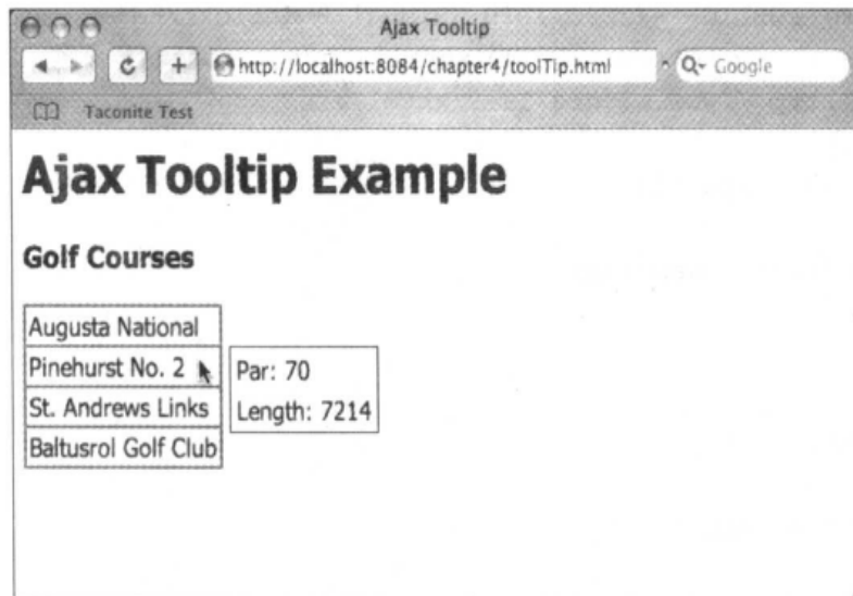
图 4-13 Ajax 工具提示示例
