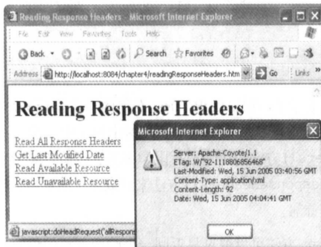
图 4-3 显示所有响应首部
