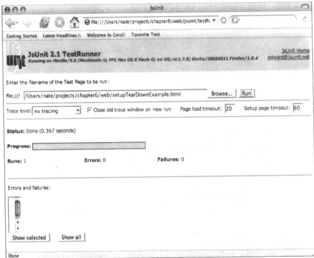
图 6-6 运行 setUp() / tearDown() 的例子
