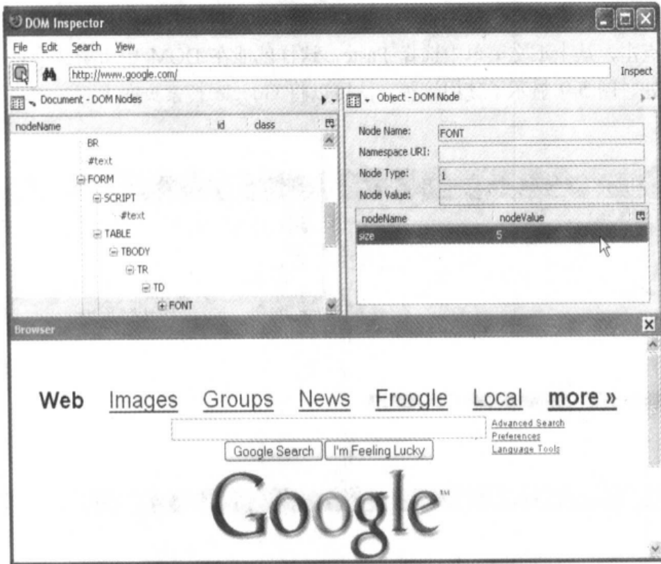
图 5-10 使用 DOM Inspector, 动态修改输入框上方的字体大小
