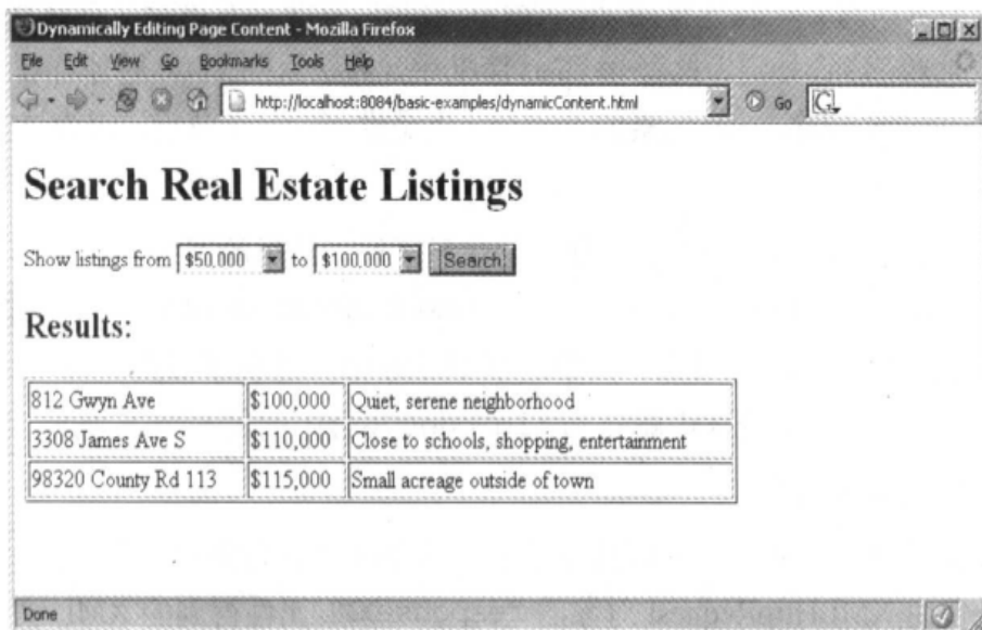
图 3-3 使用 W3C DOM 方法和 JavaScript 动态创建搜索结果
