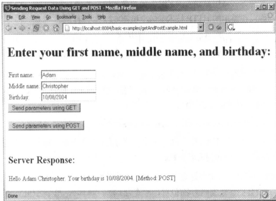
图 3-4 浏览器使用 GET 或 POST 方法发送输入数据，服务器回显输入数据作为响应
