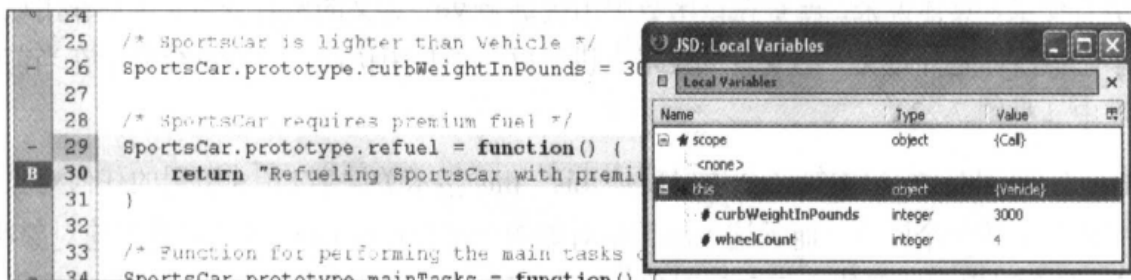
图 7-24 在对象的成员函数中暂停执行, Local Variable 窗口显示了对应的属性
