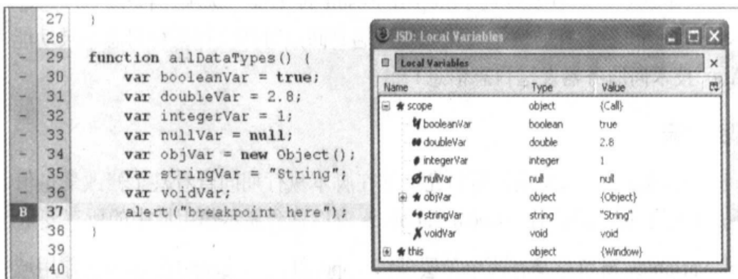
图 7-23 Local Variables 窗口显示了每种可用的数据类型
