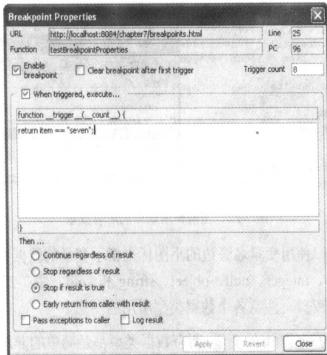
图 7-21 配置一个断点，从而只基于一个条件暂停执行
