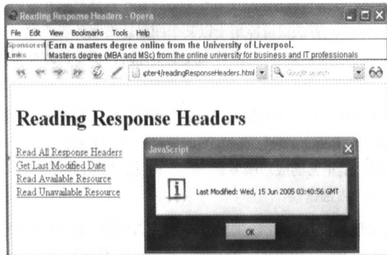
图 4-4 读取一个响应首部, 在这里是 Last-Modified 首部
