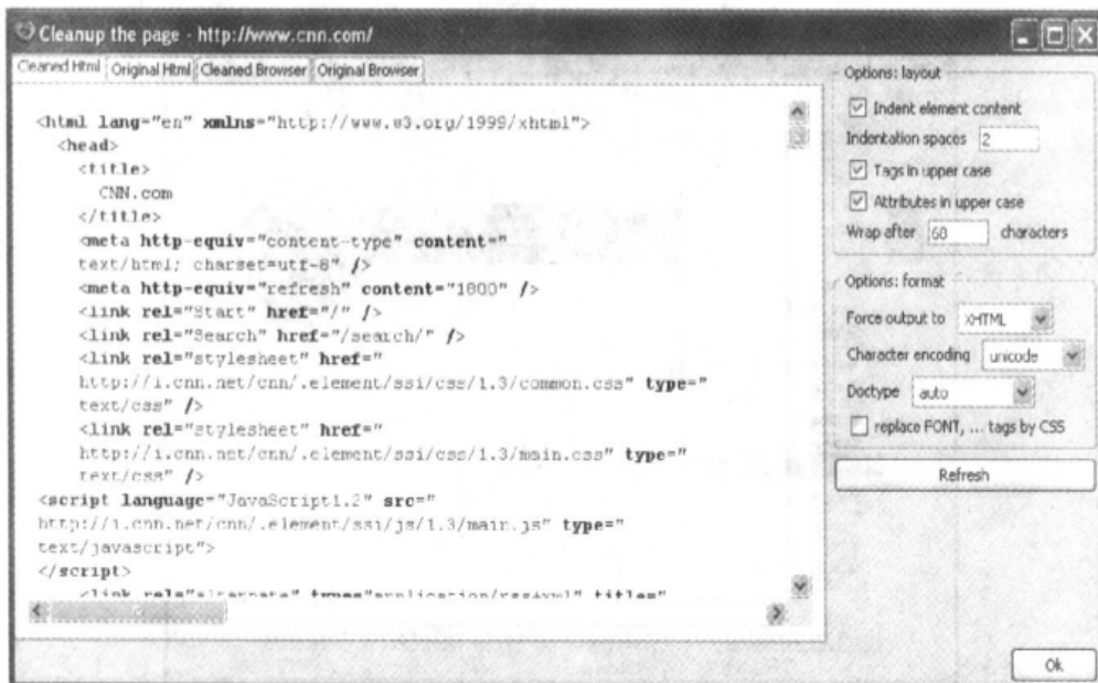
图 5-4 HTML Validator 的 Cleanup the Page 对话框给出了新的源代码，这个源代码已经修正了在原来的源 HTML 代码中发现的错误
