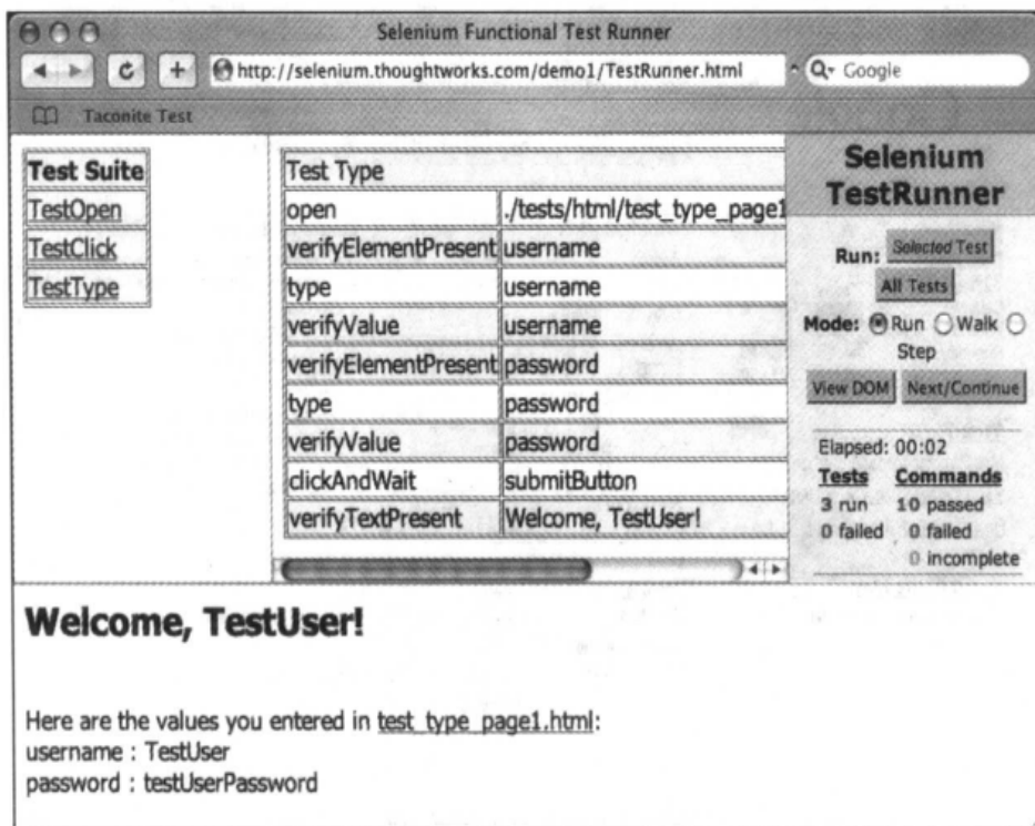
图 1-8 Selenium
