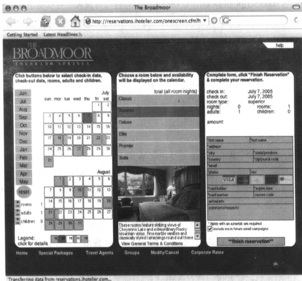
图 1-4 Flash 应用
