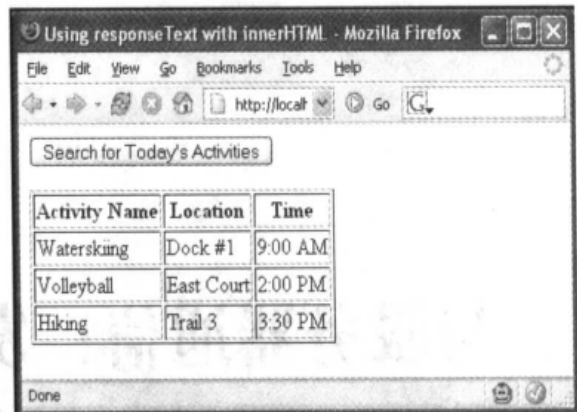
图 3-1 浏览器窗口显示了使用 XMLHttpRequest 获取并使用 innerHTML 处理的搜索结果
