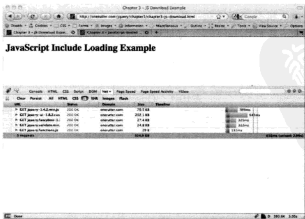
图10-2 Firebug显示一个页面中包含多个jQuery插件
