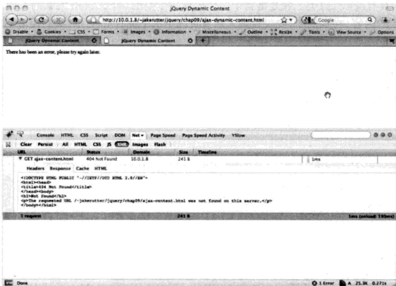
图9-4 当被请求内容不可用时，一条404错误信息显示出来
