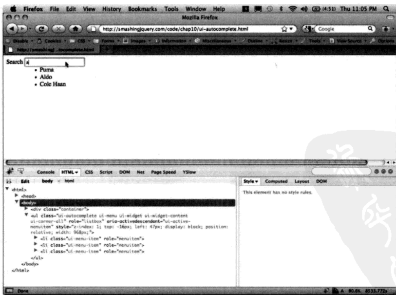
图 10-13 一个 jQuery UI 自动完成组件示例
