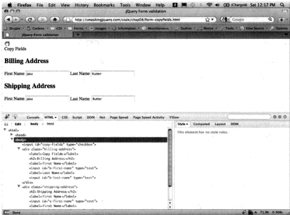
图8-15 工作中的复制功能复选框
