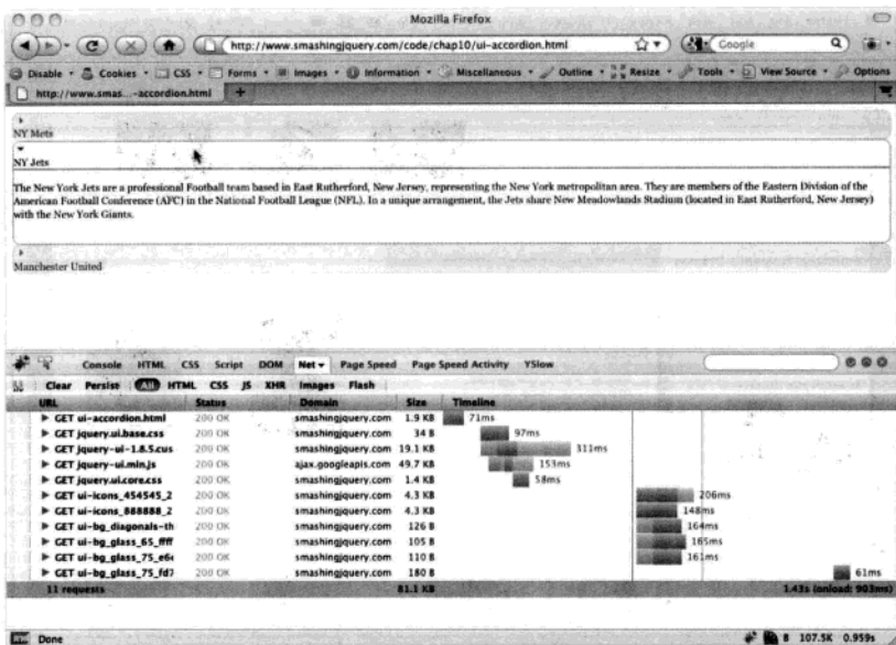
图 10-11 jQuery UI 折叠组件示例
