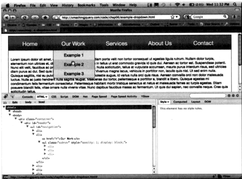
图 6-6 Firefox 浏览器中 Firebug 插件已开启，可观察到 DOM 中下拉菜单代码的变化
