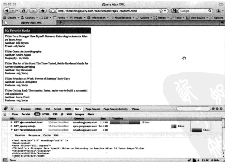
图9-12 得到XML并生成My Favorite Books（我最喜欢的书）组件
