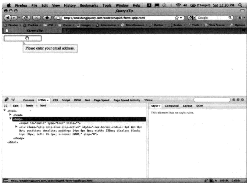
图8-17 使用qTip显示表单提示信息
