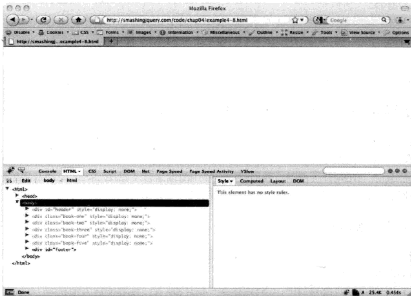
图3-8 选取多种类型元素并设置样式之后的浏览器输出
