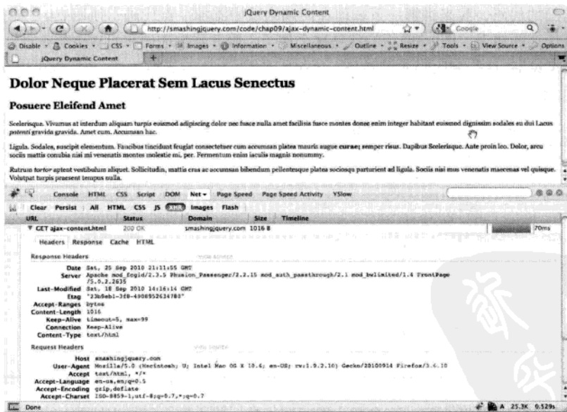
图9-3 使用.load()方法动态载入内容
