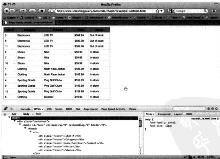
图7-13 tablesorter插件已经应用到前面HTML代码对应的表格上
