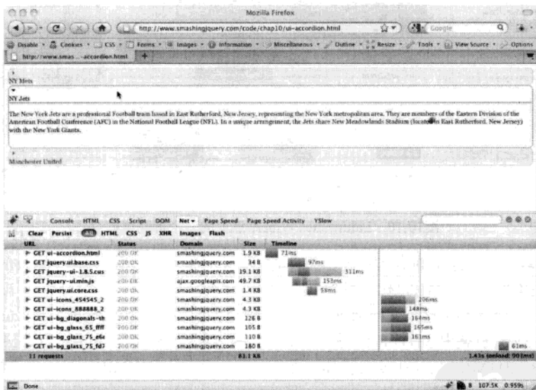
图10-11 jQuery UI 折叠组件示例 (另见插图10-11)
