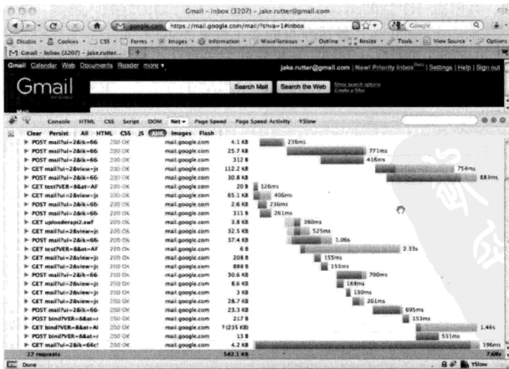
图9-2 Firebug呈现的由Gmail发起的XHR请求
