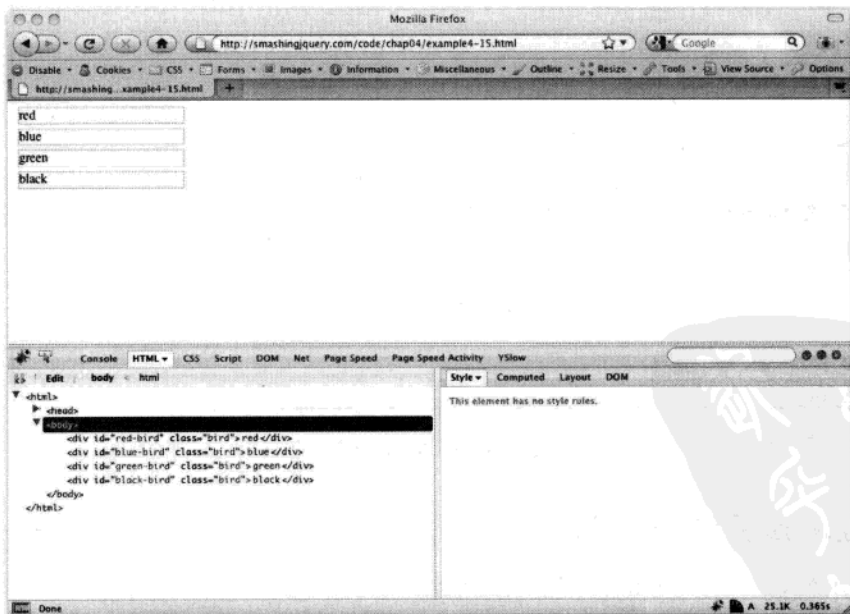
图3-15 匹配bird成功并设置样式之后的浏览器输出
