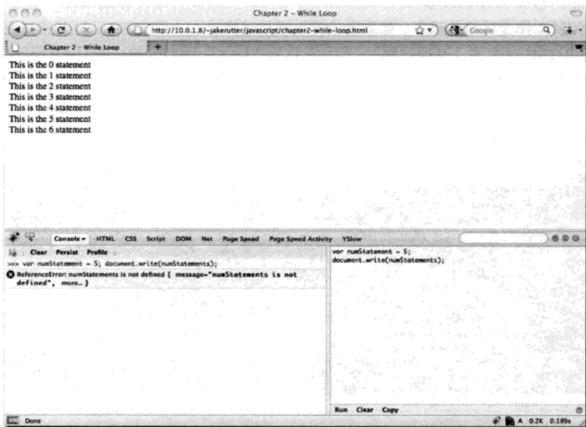
图2-10 Firebug控制台及其中显示的错误信息
