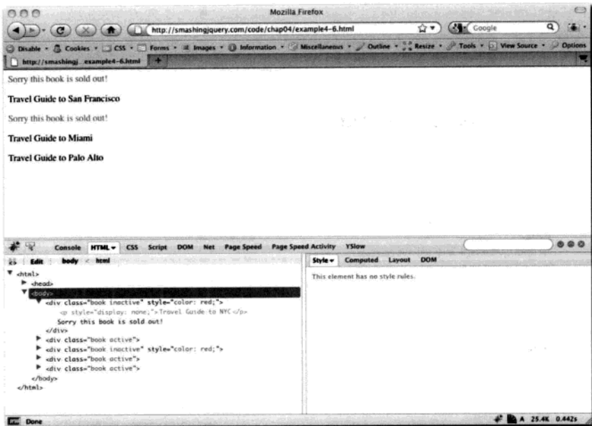
图 3-6 选取元素并设置样式之后的浏览器输出
