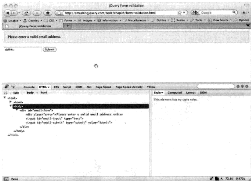
图8-13 若用户输入的电子邮件地址格式不正确，在单击Submit（提交）按钮时会显示一条提示信息
