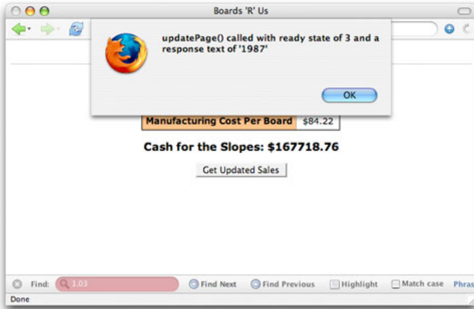
图 4. 就绪状态为 3 的响应文本
