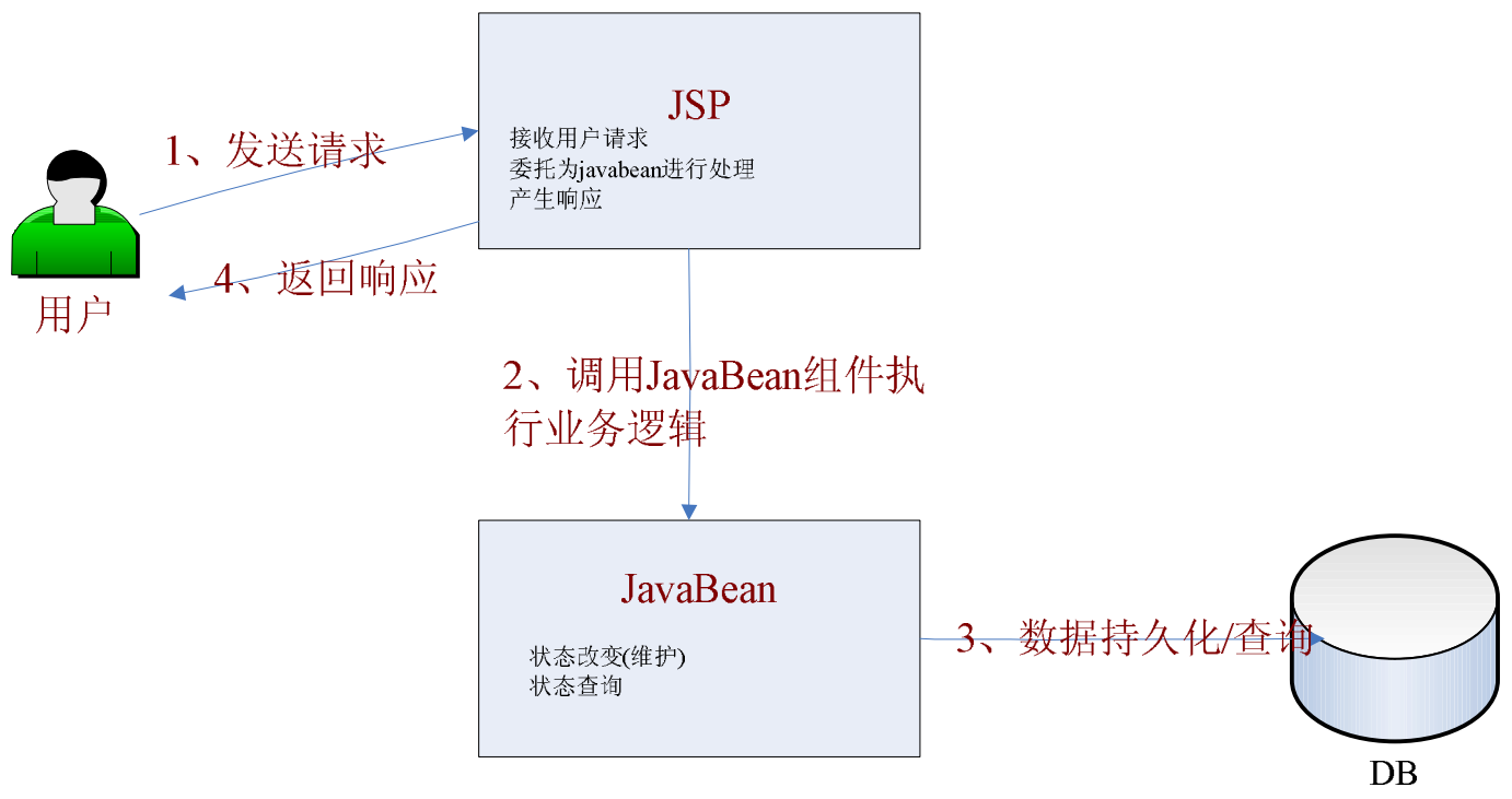
图 1-8 Model1 架构
