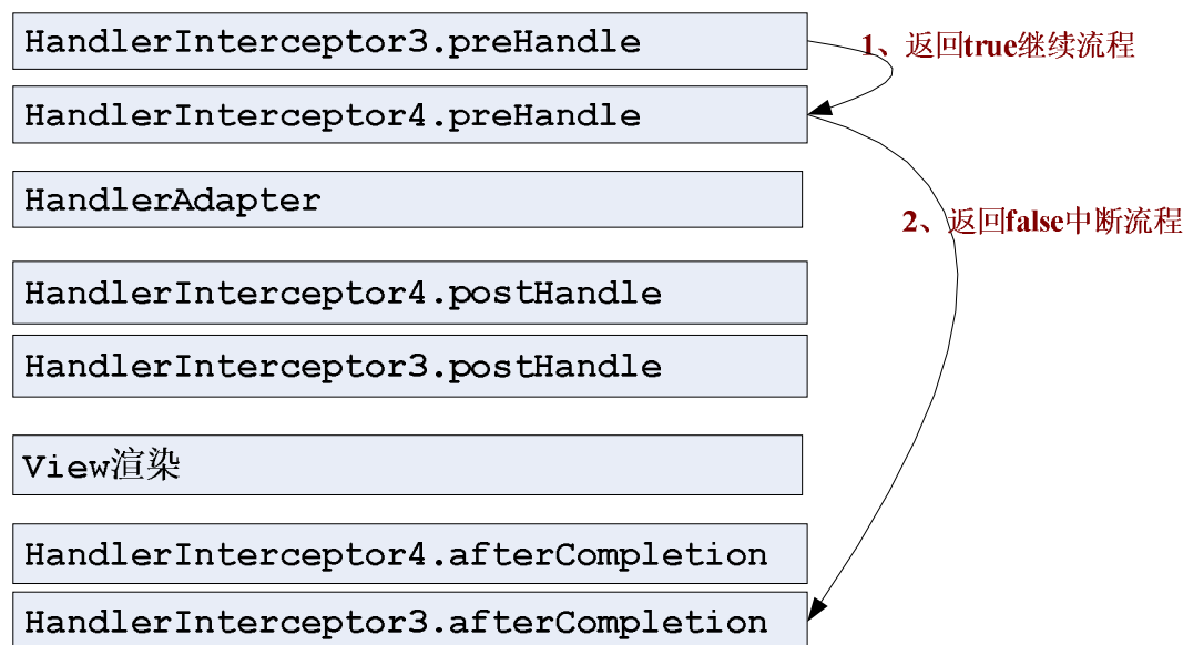
图 5-2 中断流程
