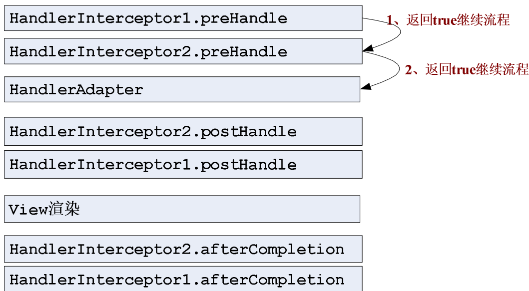
图 5-1 正常流程
