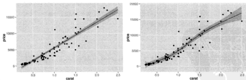
图 2.7 在运用线性模型作为平滑器时 formula 参数的作用。左图是 \text{formula} = y \sim x 的默认值, 右图是 \text{formula} = y \sim \text{ns}(x, 5) 。
