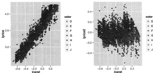
图 5.14 进行数据变换以移除显而易见的效应。左图对 x 轴和 y 轴的数据均取以 10 为底的对数以剔除非线性性。右图剔除了主要的线性趋势。
