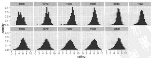
图 7.3 每十年电影平均评分的分布。
