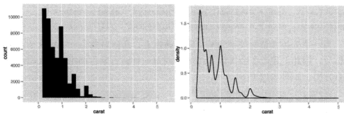
图 2.10 展示钻石重量的分布。左图使用的是 geom = "histogram" 右图使用的是 geom = "density" 。
