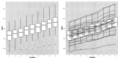
图 4.5 如果想用箱线图来查看每个时期的高度分布，默认的分组是正确的 (左图)。如果想用 geom_line() 添加每个男孩的轨迹，就需要在新图层里设定 aes(group = Subject) (右图)。
