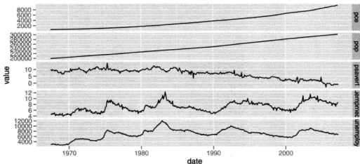
图 7.5 自由度在展示不同量纲的时间序列时非常有用。
