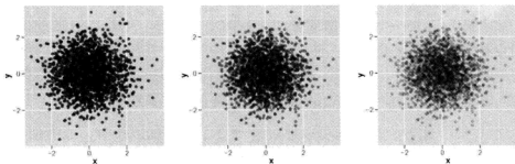
图 5.8 以从一个二元正态数据中抽样所得的数据为例，使用 \alpha 混合来减轻遮盖绘制问题。 \alpha 值从左至右分别为：1/3, 1/5, 1/10。
