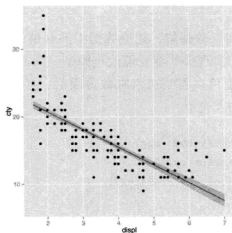
图 9.10 一个拟合得不好的简单线性模型。
