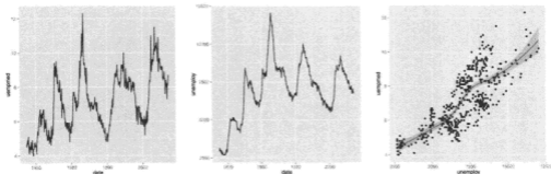
图 9.3 如果 economics 数据是“宽”的格式时，很容易分别画出两个变量的时间序列图（左图和中图），也很容易画出散点图（右图）。
