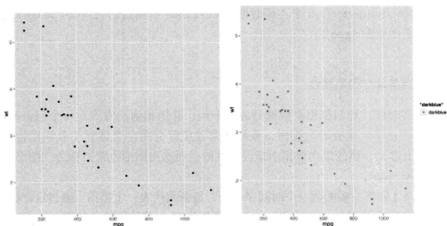
图 4.2 (参见彩图 9) 将颜色设定为 "darkblue" (左) 与将颜色映射到 "darkblue" (右) 的区别。当颜色映射到 "darkblue" 时, "darkblue" 将被看作一个普通的字符串, 使用默认的颜色标度进行标度转换, 结果得到了粉红色的点和图例。
