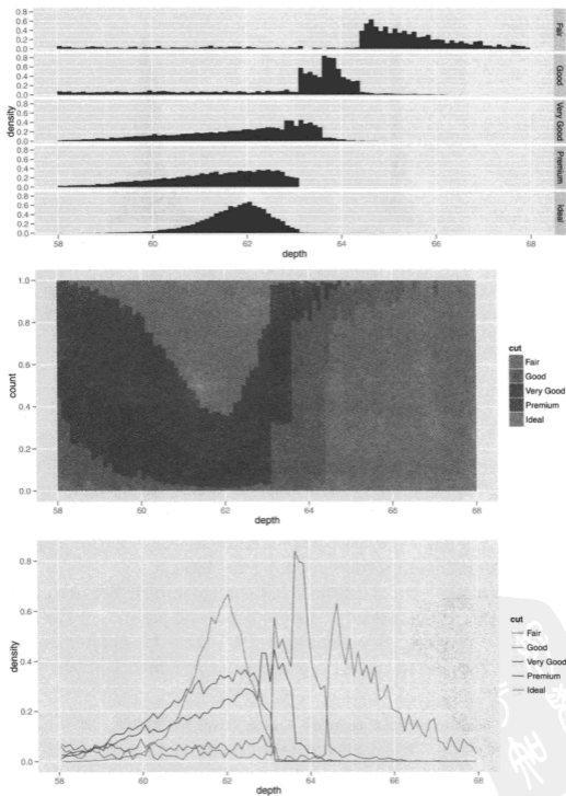
图 5.3 (参见彩图 14) 钻石数据切割和深度分布的三种视图。从上至下分别是分面直方图、条件密度图和频率多边形图。它们都显示出了一个有趣的模式：随着钻石质量的提高，分布逐渐向左偏移且愈发对称。
