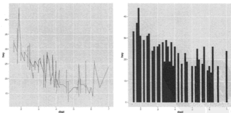
图 3.2 除了用点来表示数据，我们还可以用其他的几何对象，如直线（左）或条形（右）。对于这个数据，用这两种几何对象所作的图形都没有什么意义，但在语法上是有效的。
