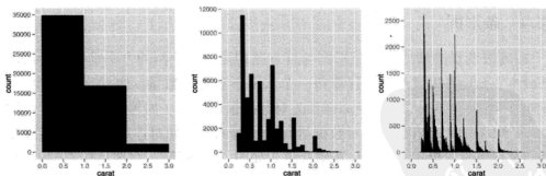
图 2.11 变动直方图的组距可以显示出有意思的模式。从左到右，组距分别为 1, 0.1 和 0.01。只有重量在 0 到 3 克拉之间的钻石显示在图中。
