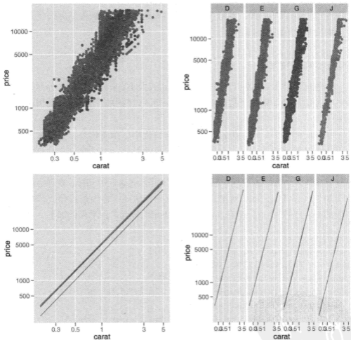
图 7.7 (参见彩图 28) 分面与分组的差异：克拉与价格的双对数图，四种颜色标注。
