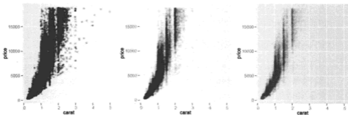
图 2.3 将 alpha 值从 1/10(左) 变动到 1/100(中) 再到 1/200(右), 来看大部分的点在哪里进行重叠。
