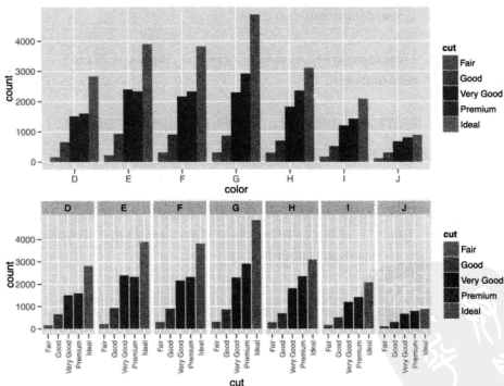
图 7.8 (参见彩图 29) 并列 (上) vs 分面 (下) 对于水平完全交叉的变量对。
