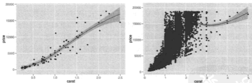
图 2.4 重量与价格的散点图中加入了平滑曲线。左图为 dsmall 数据集，右图为完整数据集。
