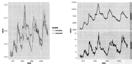
图 9.5 (参见彩图 36) 当序列数据大小差异很大时, 可以使用两种方法: 左图, 把数据调整到相同的尺度上; 右图, 把数据画在不同的分面图形上。
