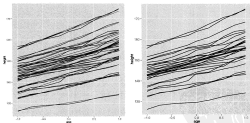
图 4.4 给 Oxboys 数据添加光滑曲线。左图用了和折线图同样的分组变量, 得到了每个男孩的拟合直线。右图在平滑层里用了 aes(group = 1) , 得到了所有男孩的拟合直线。
