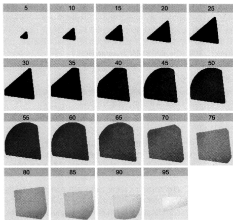
图 6.6 (参见彩图 20)hcl 色彩空间的形状。色相被映射为角度, 彩度被映射为半径, 每个分面各自表示一种明度。hcl 色彩空间的形状比较奇异, 但我们也能够看出每个分面的中心为灰色, 随着向边缘移动, 颜色变得愈加浓烈。明度为 0 和 100 的切片已被省略, 因为它们分别是一个黑点和一个白点。
