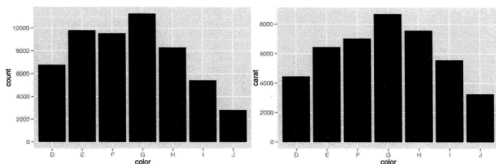
图 2.13 钻石颜色的条形图。左图显示的是分组的计数，右图是按 weight = carat 进行加权，展示了每种颜色的钻石的总重量。
