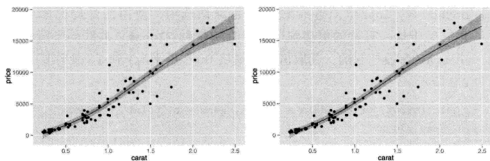
图 2.6 在运用广义可加模型作为平滑器时 formula 参数的作用。左图是 \text{formula} = y \sim s(x) ，右图是 \text{formula} = y \sim s(x, \text{bs} = \text{"cs"}) 。
