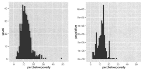
图 5.20 不含权重信息 (左侧) 以及含权重信息 (右侧) 的直方图。不含权重信息的直方图展示了郡的数量, 而含权重信息的直方图展示了人口数量。权重的加入的确极大地改变了对图形的解读!
