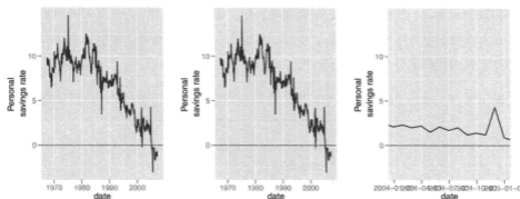
图 6.5 个人储蓄率的时间序列图。 (左图) 默认外观, (中图) 每隔 10 年为一断点, 以及 (右图) 使用年月日的格式仅显示在 2004 年内的图形。测量值是在每月月末记录的。
