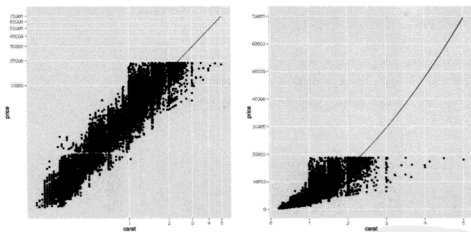
图 7.16 (左) 克拉与价格对数变换后的散点图。直线为回归曲线： \log(y) = a + b \times \log(x) 。(右) 将前面的图变换回去 ( coord_trans(x = "pow10", y = "pow10") )，标度还原，因此线性趋势变成指数形式， y = k \times c^x 。图形很明显地揭示了克拉值大、价格贵的钻石是很稀少的。
