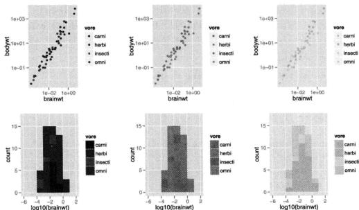
图 6.9 (参见彩图 23) 三种 ColorBrewer 调色板, Set1(左图), Set2(中图) 和 Pastell(右图), 分别应用于点(首行)和条形(次行)。更明亮的颜色对点效果良好,但对于条形来说过于刺眼。淡色对条形效果良好,但会让点看不清楚。
