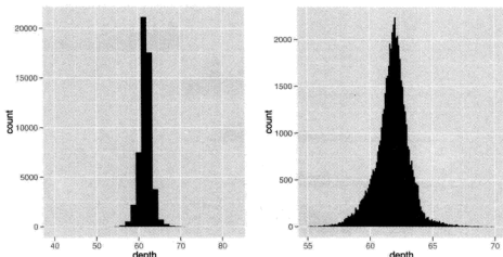
图 5.2 永远不要指望依靠默认的参数就能对某个具体的分布获得一个表现力强的图形(左图)。(右图)对 x 轴进行了放大, xlim = c(55, 70) , 并选取了一个更小的组距宽度, binwidth = 0.1 , 较左图揭示出了更多细节。我们可以发现这个分布是轻度右偏的。同时别忘了在标题中写上重要参数(如组距宽度)的信息。
