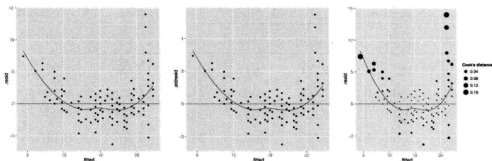
图 9.11 (左) 基本的拟合值 - 残差图。(中) 标准化的残差。(右) 点大小与 Cook 距离成比例。只要有全部的数据就可以很容易地修改基本图形。
