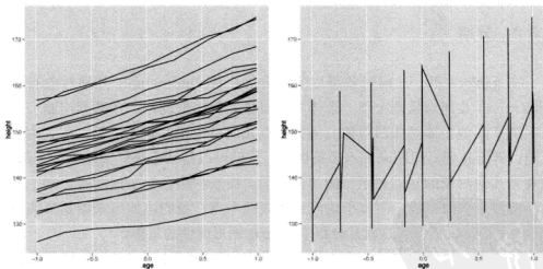
图 4.3 正确分组时 (分组变量 group = Subject ) 每个个体的折线图 (左)。错误分组时连接所有观测点的折线图 (右)。此处省略了分组图形属性，效果等同于 group = 1 。
