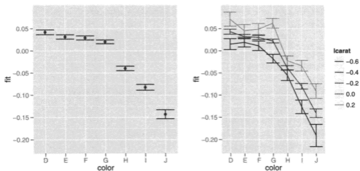
图 5.15 (参见彩图 17) 展示模型估计结果中变量 color 的不确定性。左图为 color 的边际效应。右图则是针对变量 carat 的不同水平 (level), 变量 color 的条件效应。误差棒显示了 95% 的逐点置信区间。
