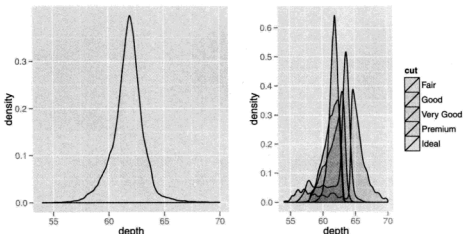
图 5.6 (参见彩图 15) 密度图实际上就是直方图的平滑化版本。它的理论性质比较理想，但难以由图回溯到数据本身。左图为变量 depth 的密度图。右图为按照变量 cut 的不同取值上色的版本。
