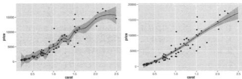
图 2.5 span 参数的作用。左图是 span = 0.2 , 右图是 span = 1 。
