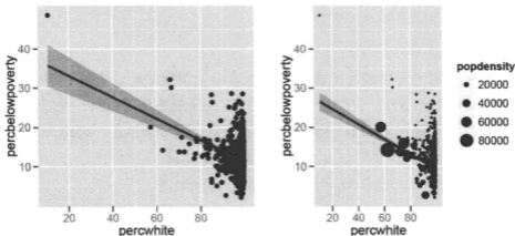
图 5.19 未考虑权重的最优拟合曲线 (左图) 和以人口数量作为权重的最优拟合曲线 (右图)。
