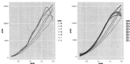
图 9.2 (参见彩图 34) 手动计算图 9.1 中的统计量。左图为预测值，右图加上标准差。
