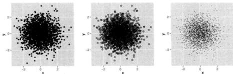
图 5.7 修改使用的符号可以帮助我们处理轻微到中等程度的遮盖绘制问题。从左至右分别为：默认的 shape 、 shape = 1 (中空点)，以及 shape = "." (像素大小的点)。
