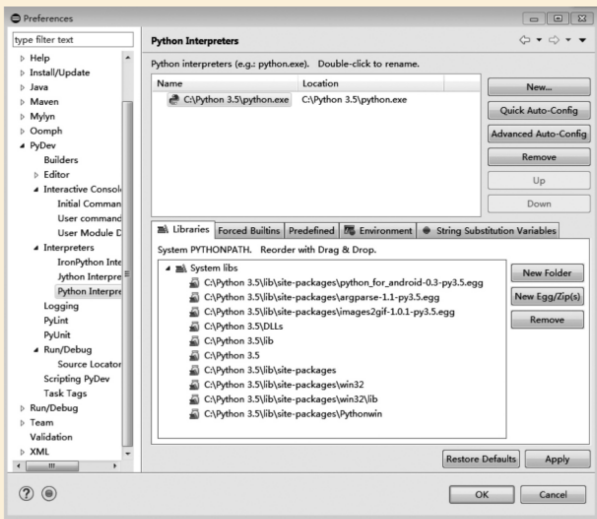
图1-3 配置Eclipse+PyDev环境
