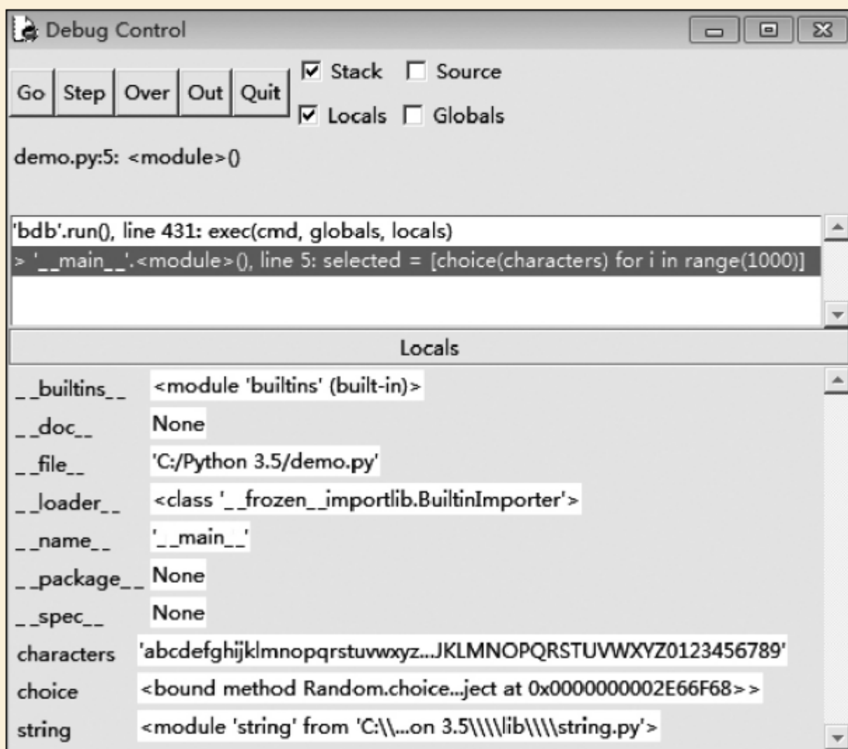
图 11-3 程序调试截图（一）
