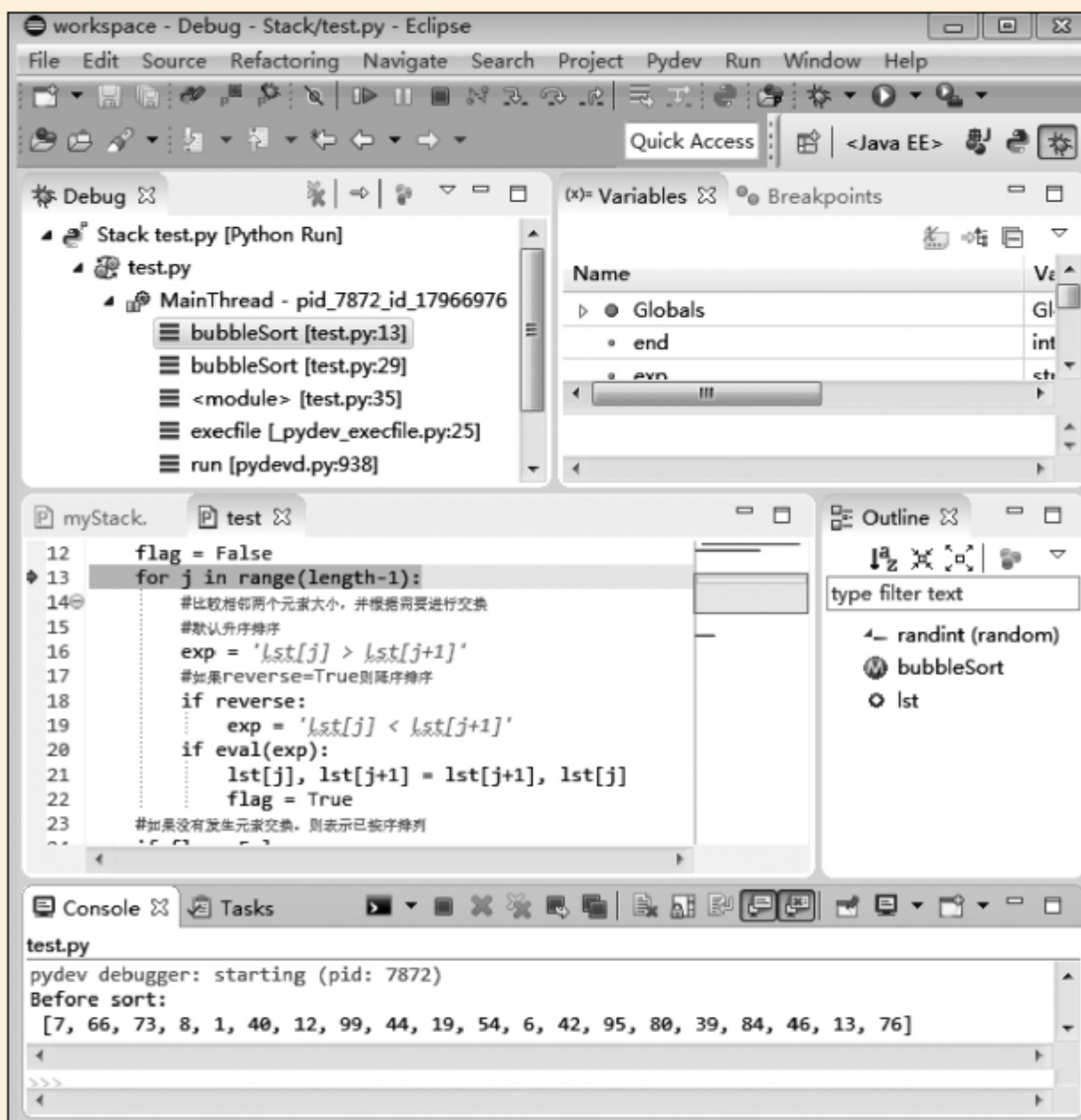
图 11-5 Eclipse+PyDev调试界面
