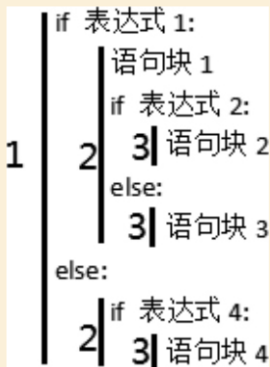
图4-4 代码层次与隶属关系
