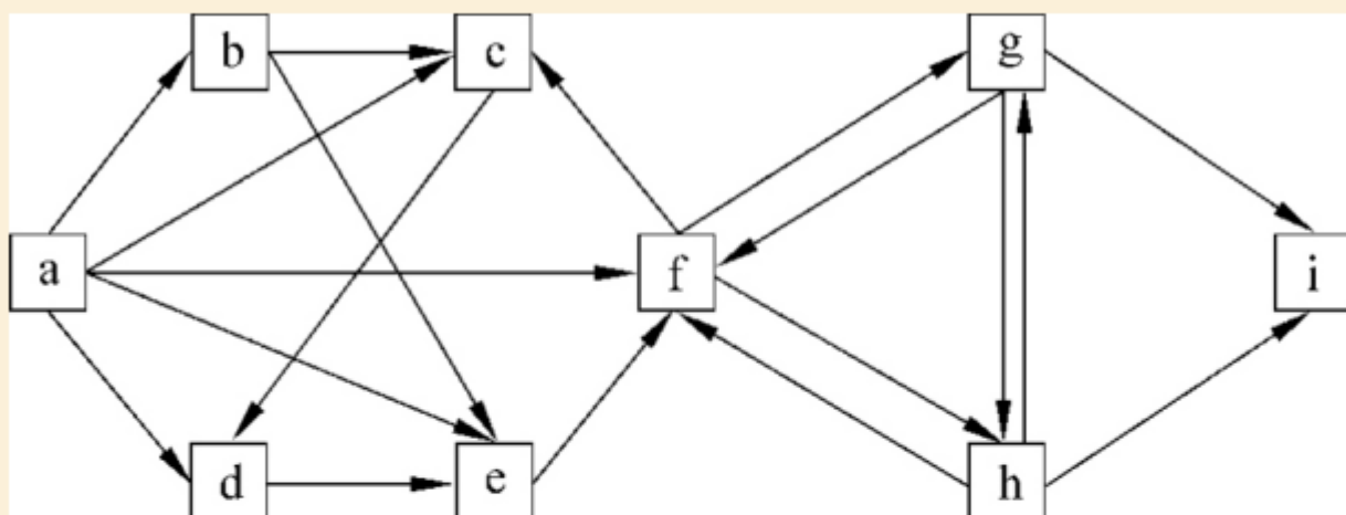
图3-3 有向图结构
