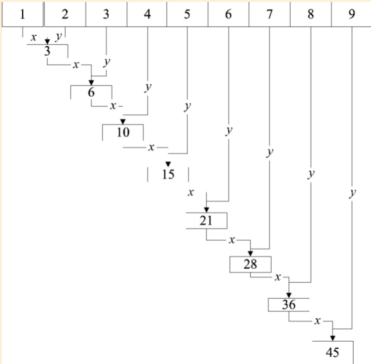
图2-1 reduce()函数执行过程示意图
