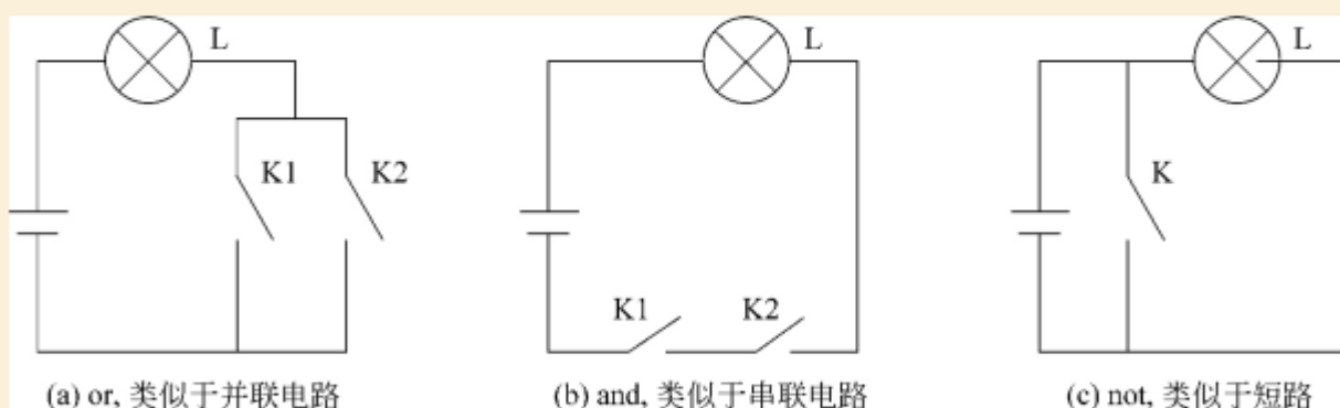
图4-1 逻辑运算符与几种电路的类比关系
