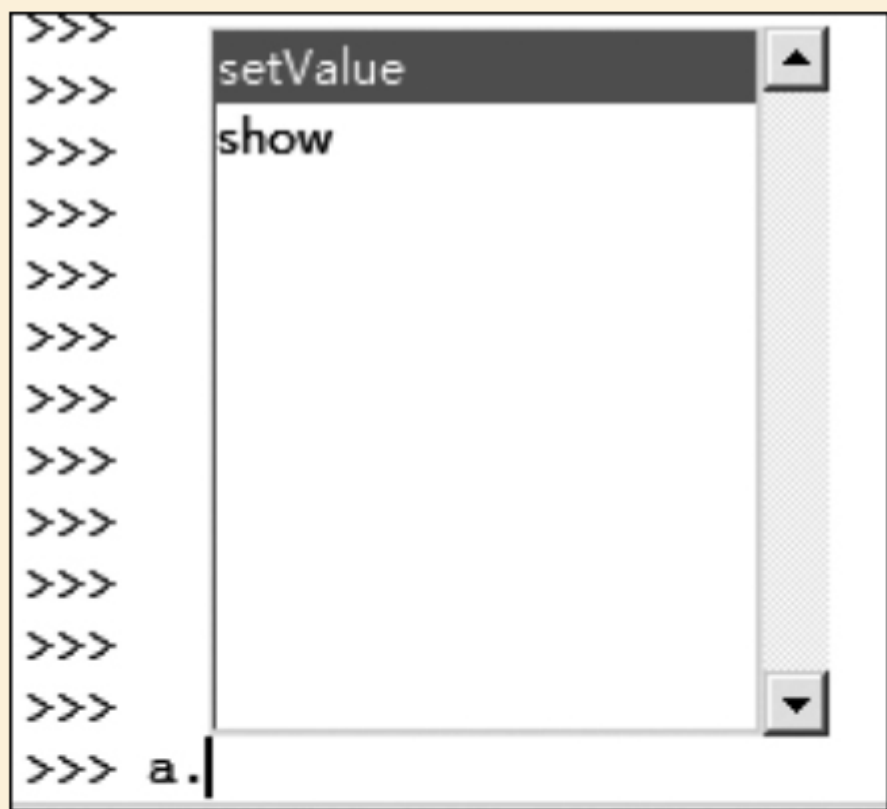
图6-1 列出对象公开成员
