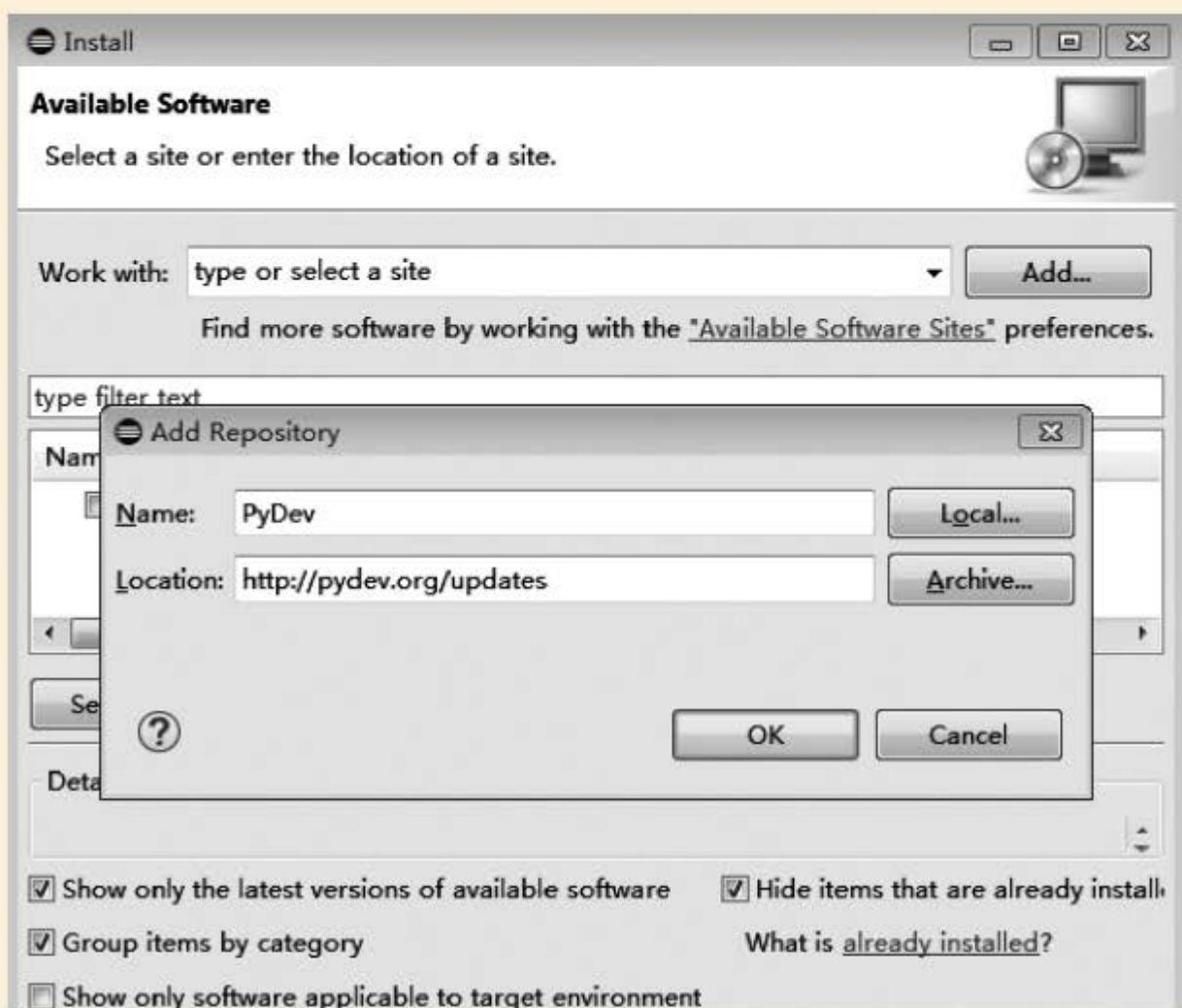
图1-2 安装PyDev
