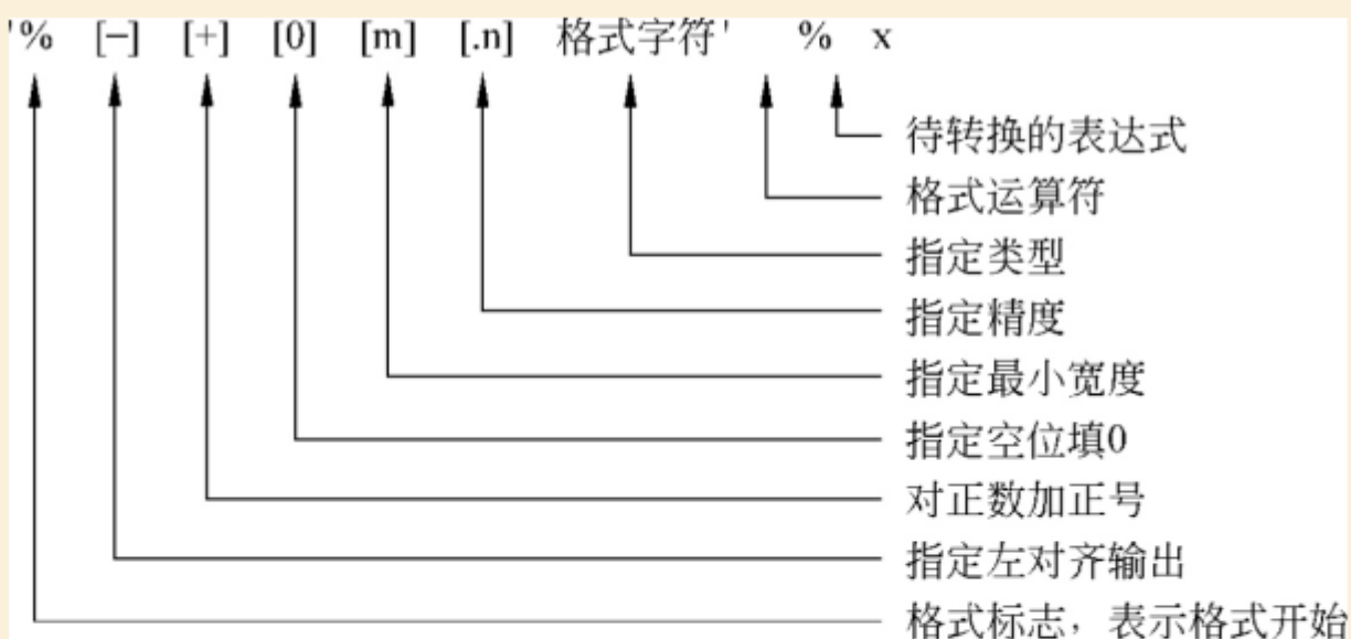
图7-1 字符串格式化
