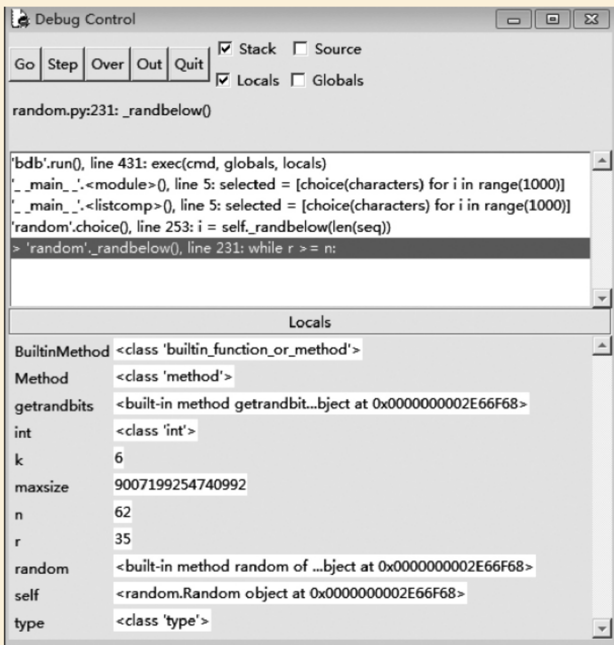
图11-4 程序调试截图（二）
