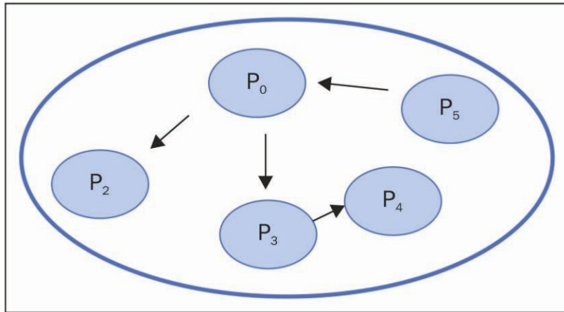
MPI.COMM_WORLD中进程间的通信示例
