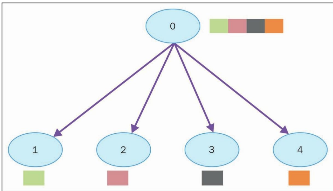
将数据从进程0散播给进程1、2、3与4
