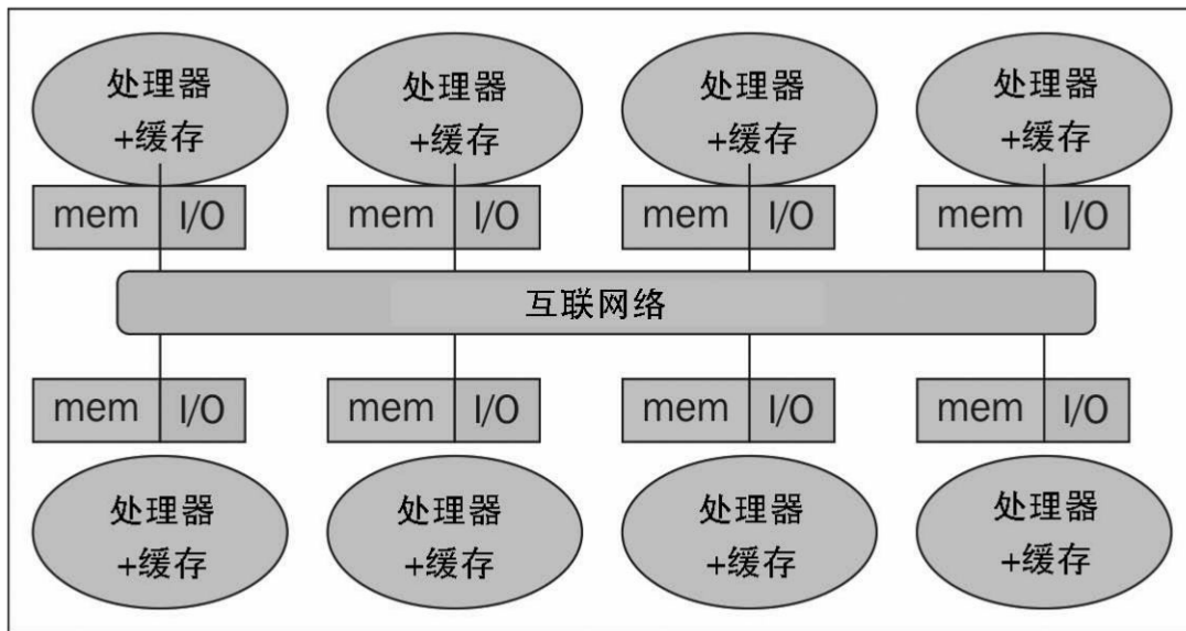
分布式内存架构模式
