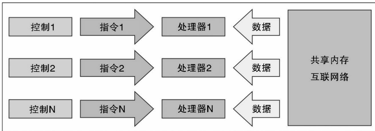
MIMD架构模式
