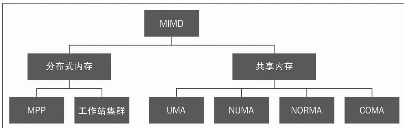
MIMD架构中的内存组织
