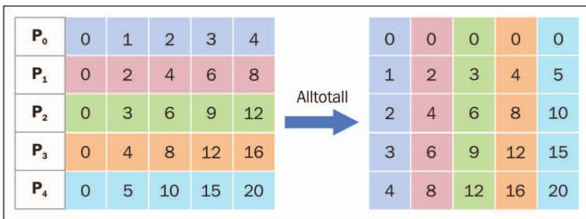
Alltoall聚合通信
