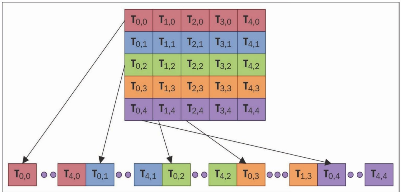
线程区块划分: T(x, y) , 其中 x = \text{threadIdx.x} , y = \text{threadIdx.y}
