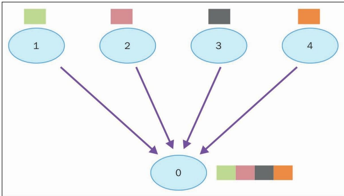
从进程1、2、3与4收集数据
