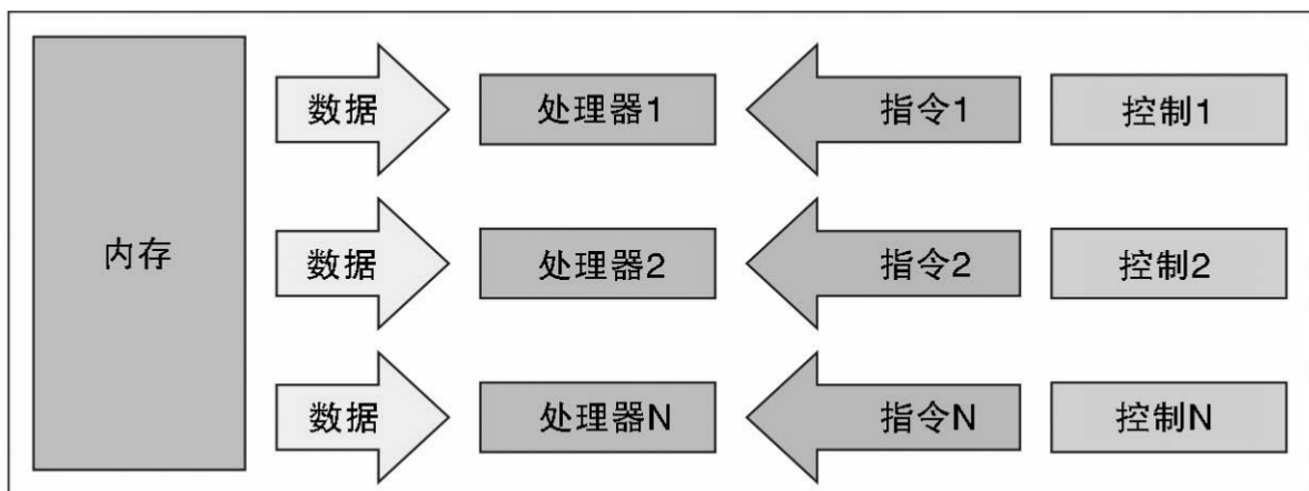
MISD架构模式
