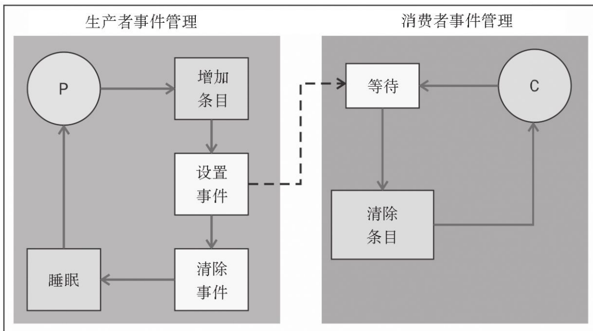
使用事件对象实现的线程同步
