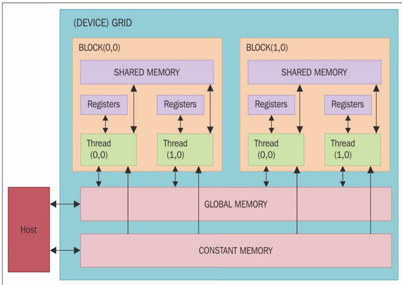
GPU内存模型
