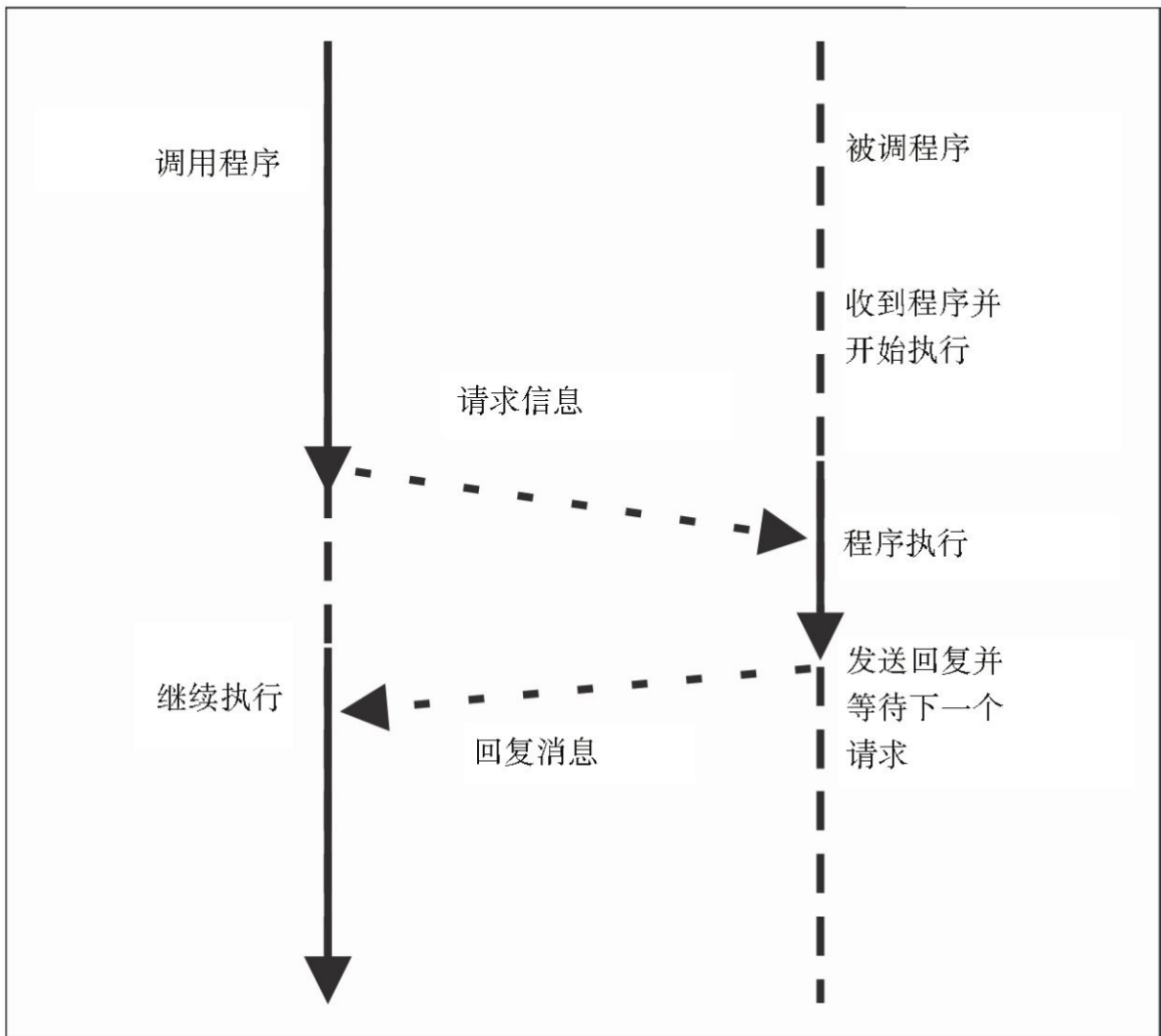
远程过程调用模式
