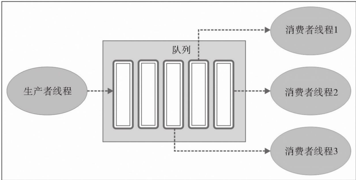
使用队列模块实现的线程同步
