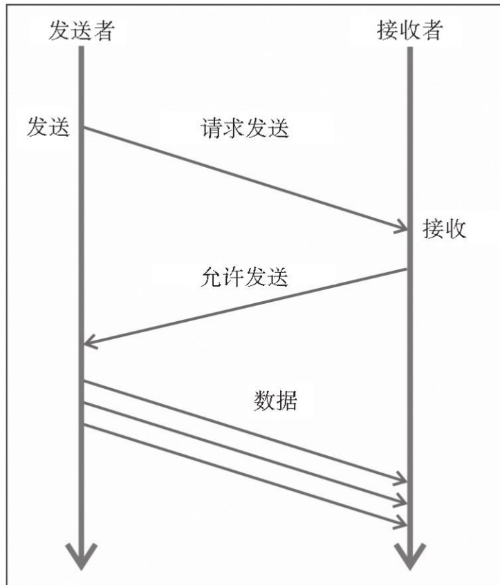
发送/接收传输协议
