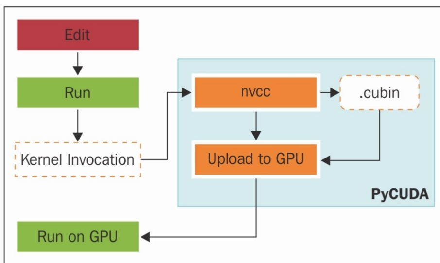
PyCUDA执行模式
