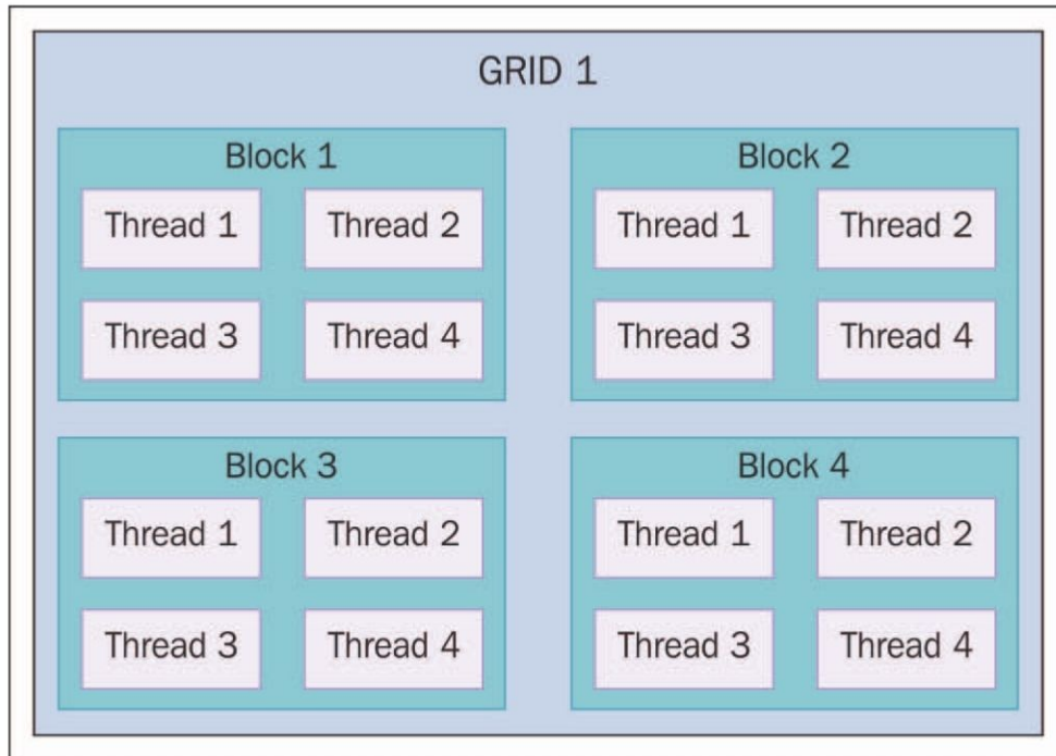
PyCUDA二层结构中（三维）线程的分布
