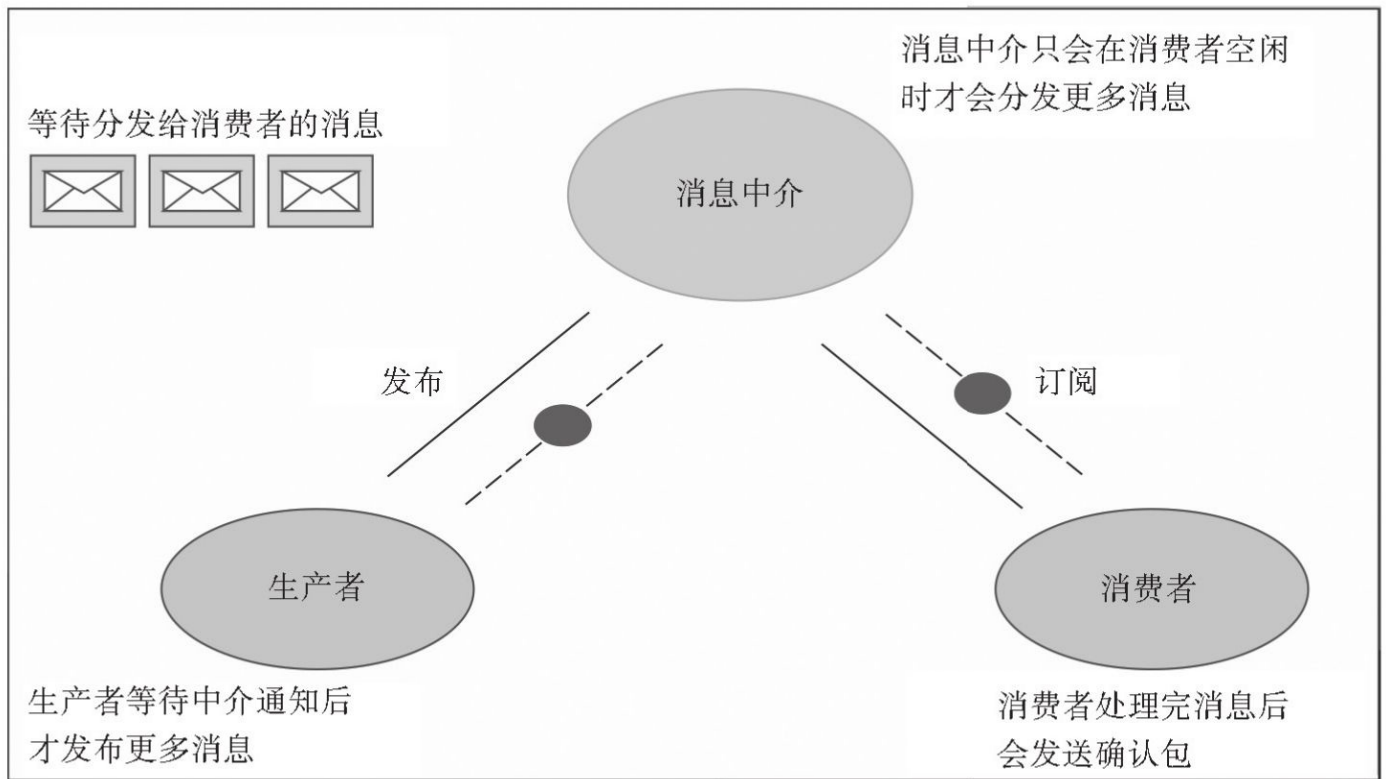
消息中介架构
