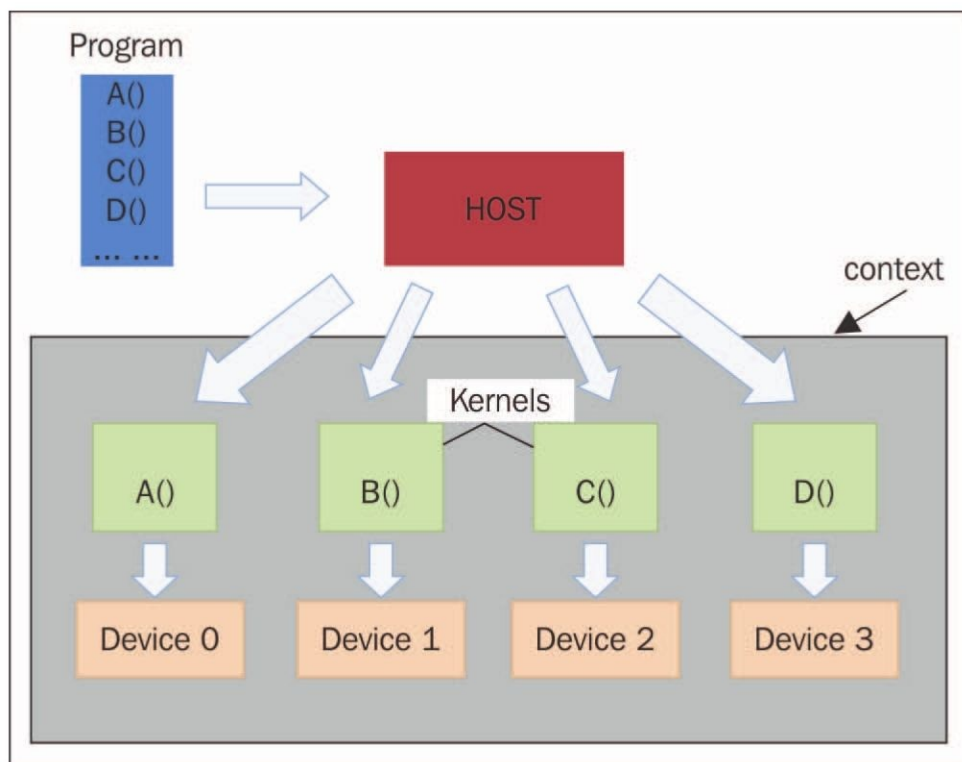
PyOpenCL编程
