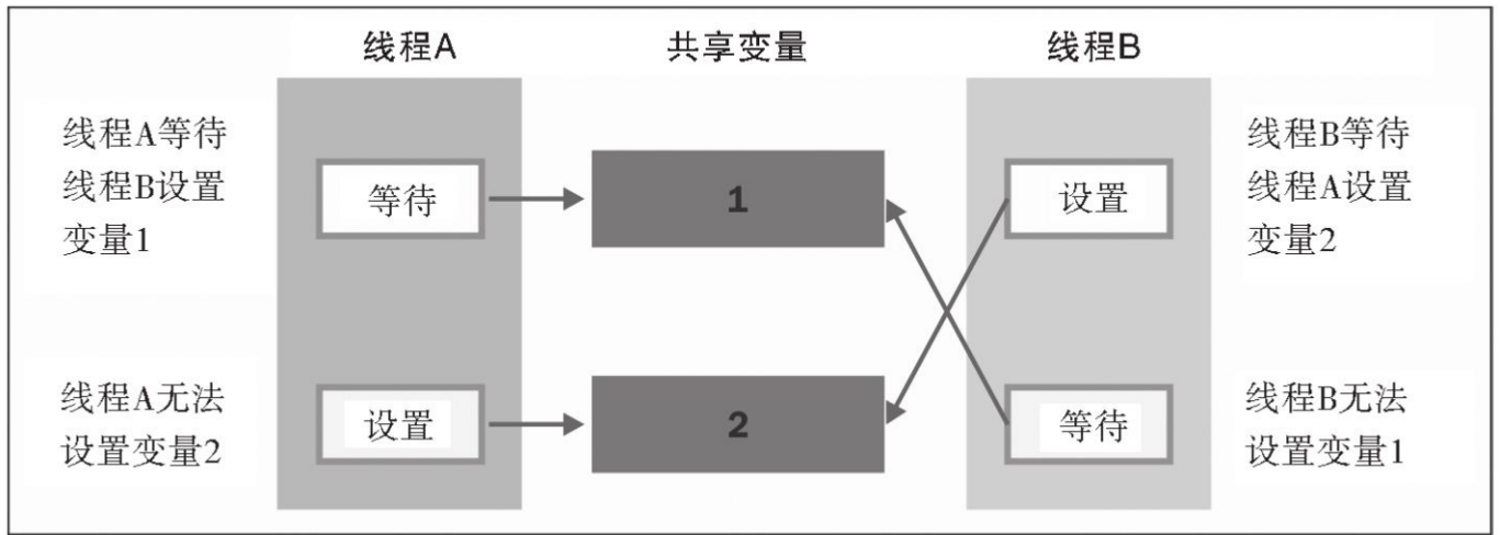
死锁
