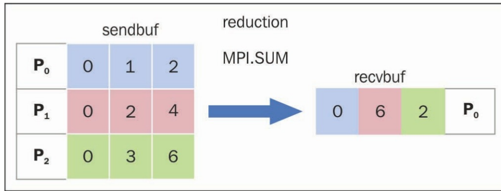
汇聚聚合通信
