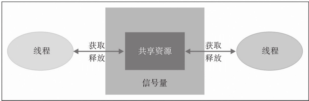
使用信号量实现线程同步
