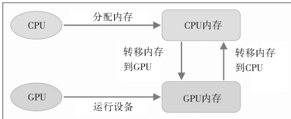
PyCUDA编程模式
