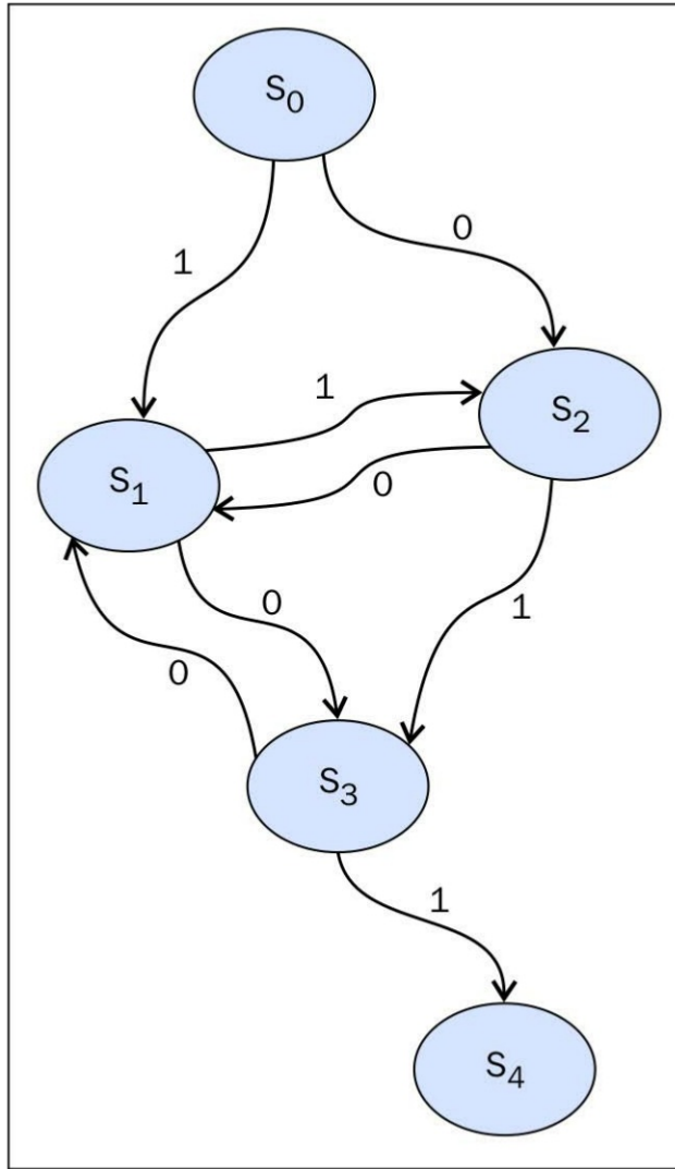
有限状态机
