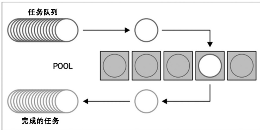
池化管理
