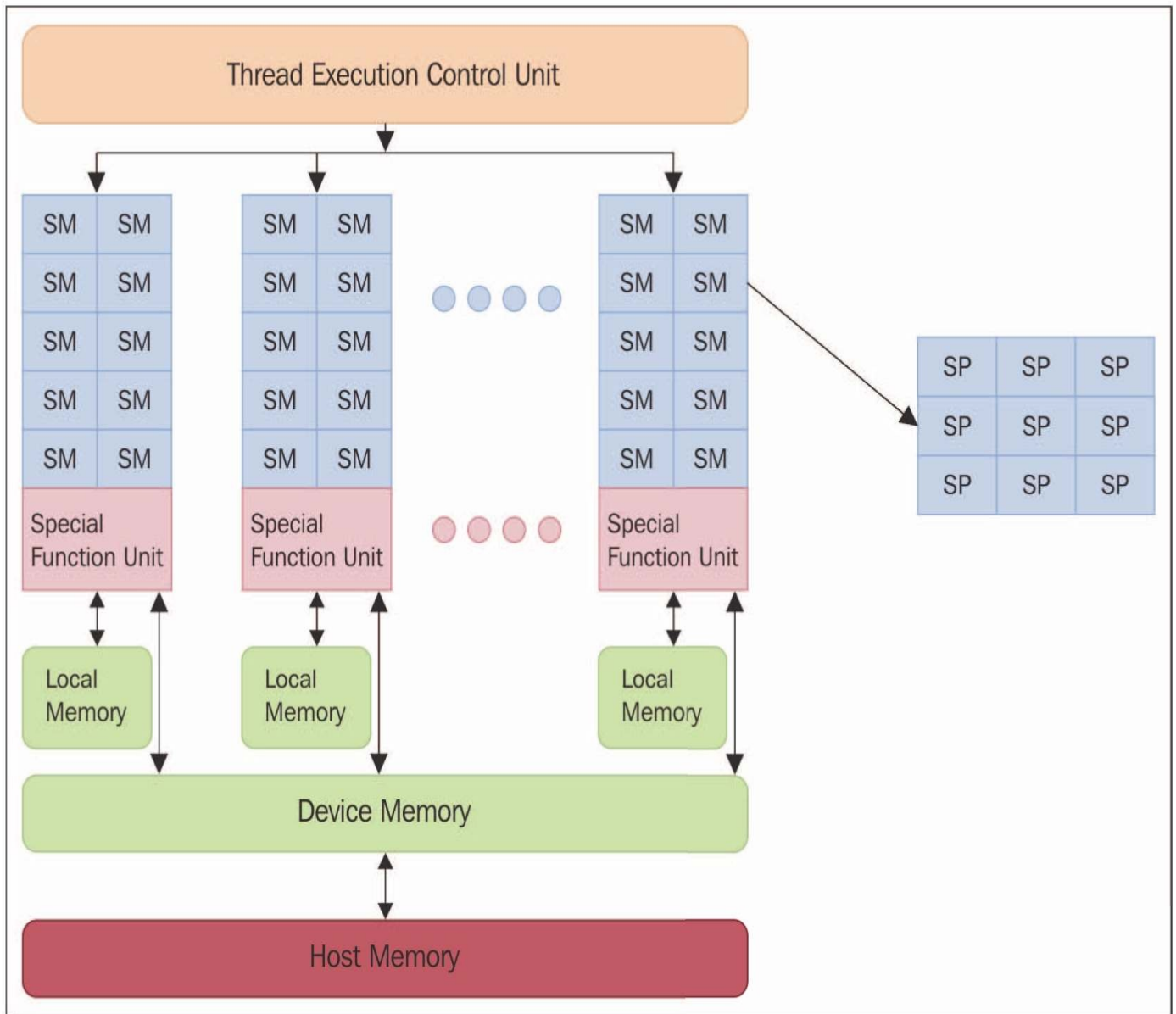
GPU架构
