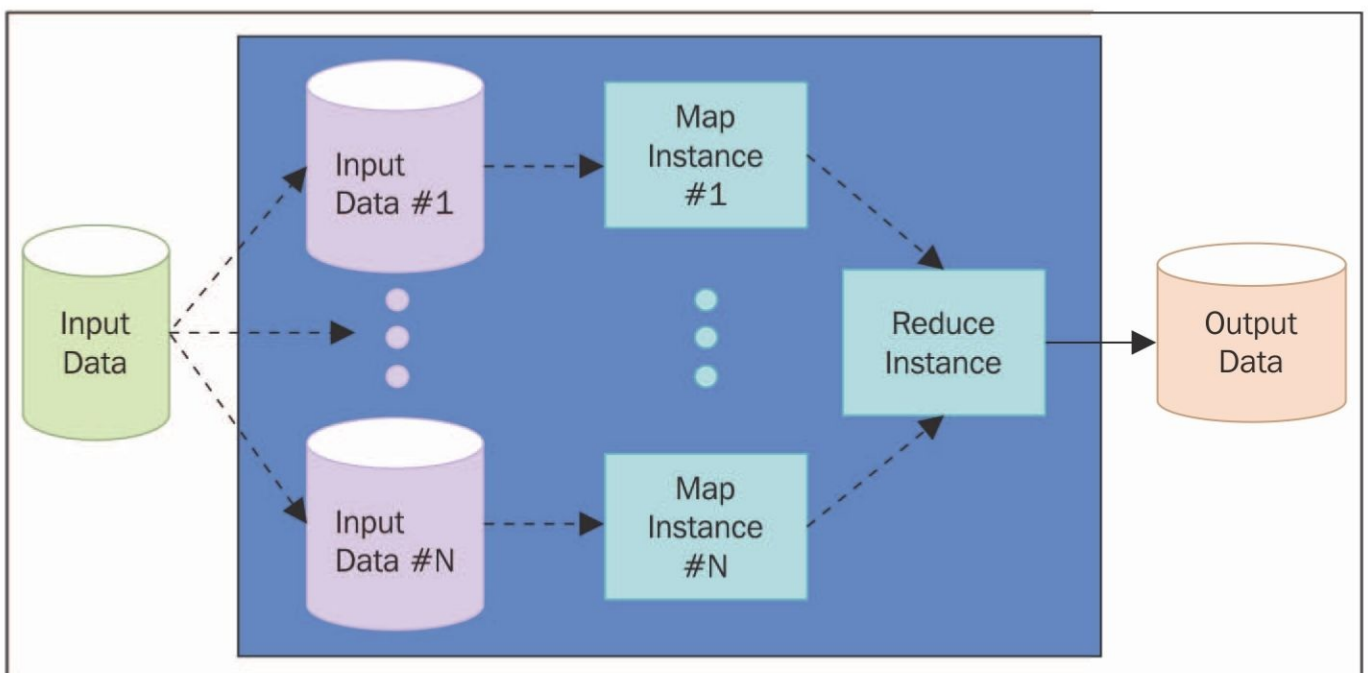
MapReduce方案
