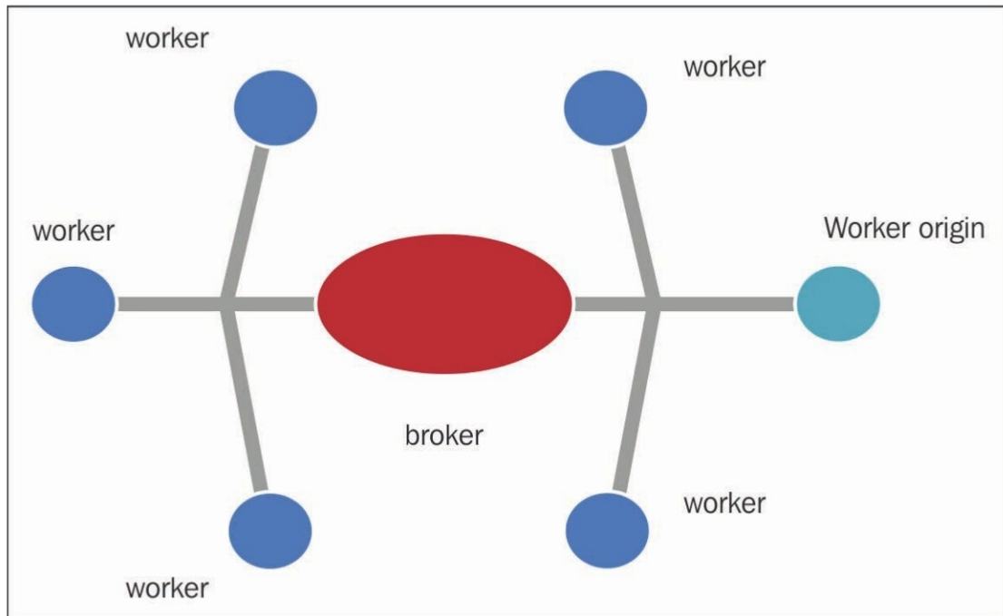
SCOOP架构
