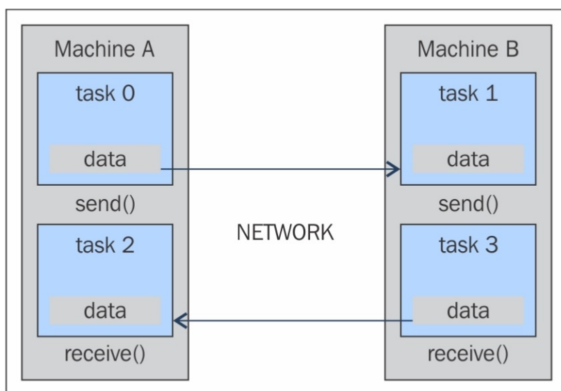
消息传递范式模型
