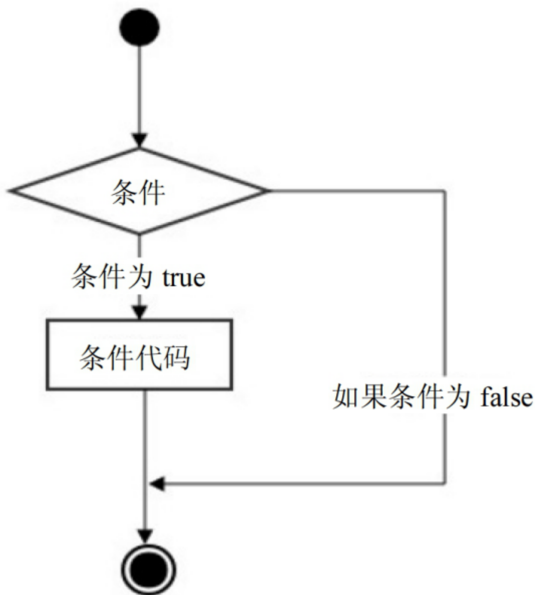
图6-5 if条件语句执行过程
