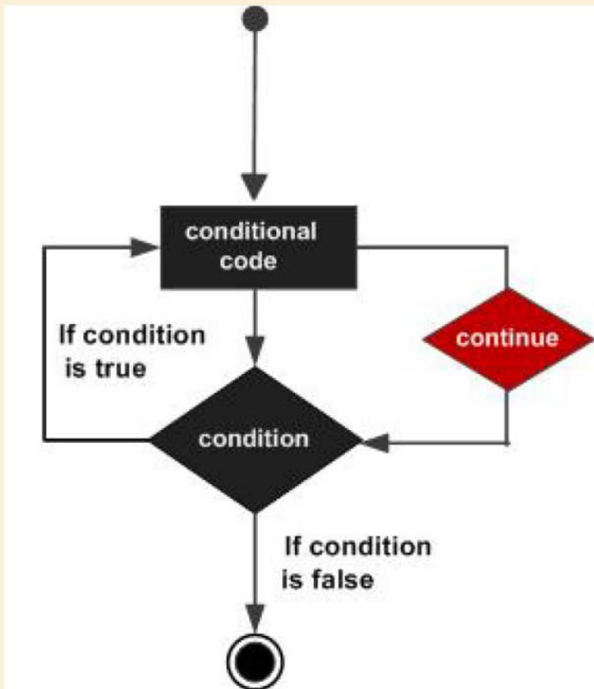
图6-10 continue执行流程
