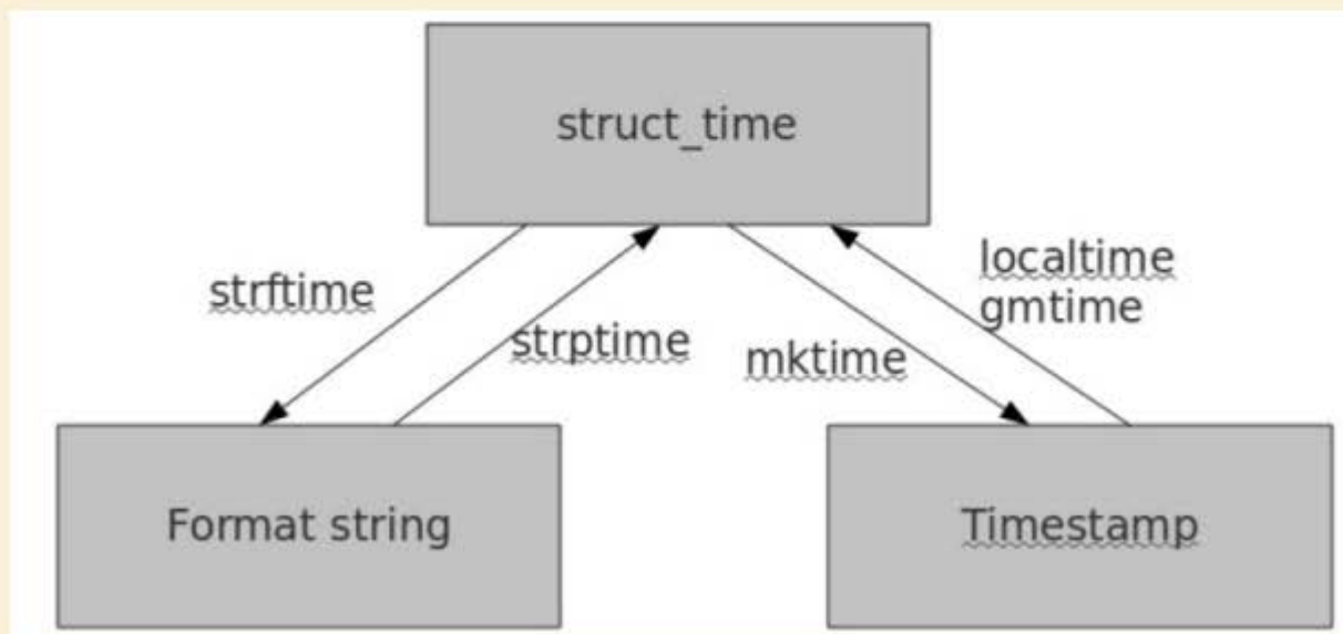
图10-1 时间格式转化1
