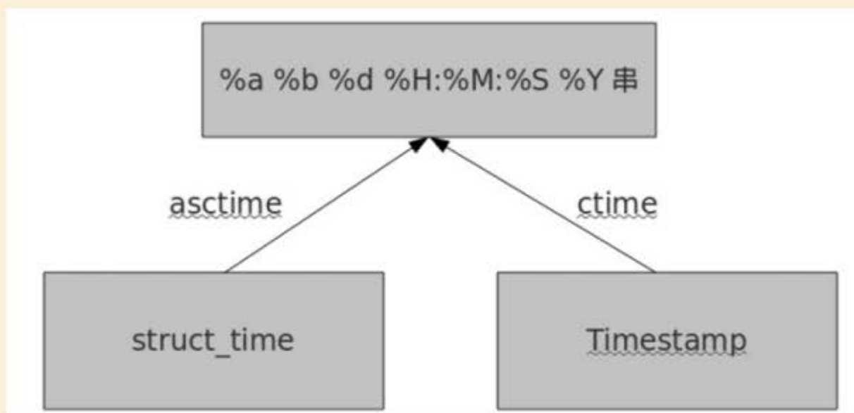
图10-2 时间格式转化2
