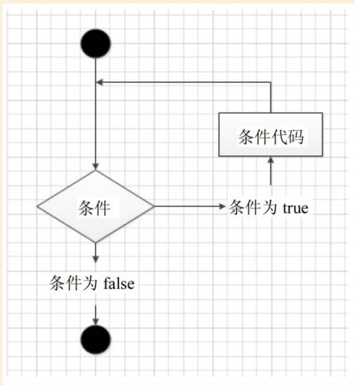
图6-6 循环语句执行流程
