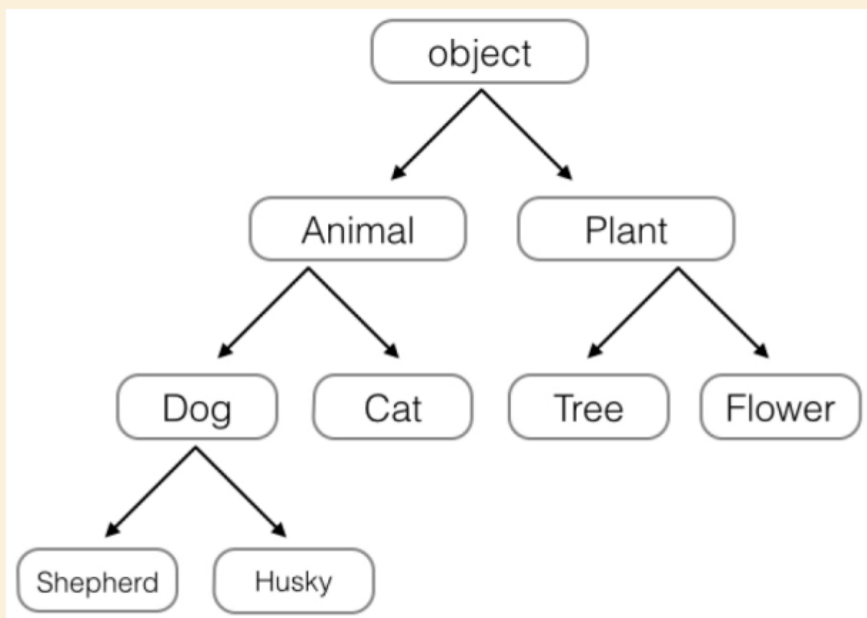
图8-1 继承树
