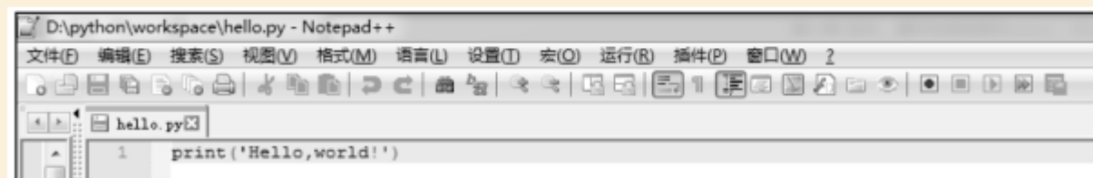
图6-2 Notepad++编辑器
