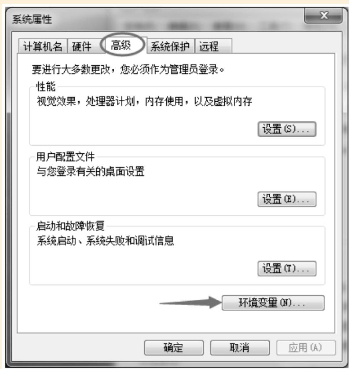
图1-18 系统属性
