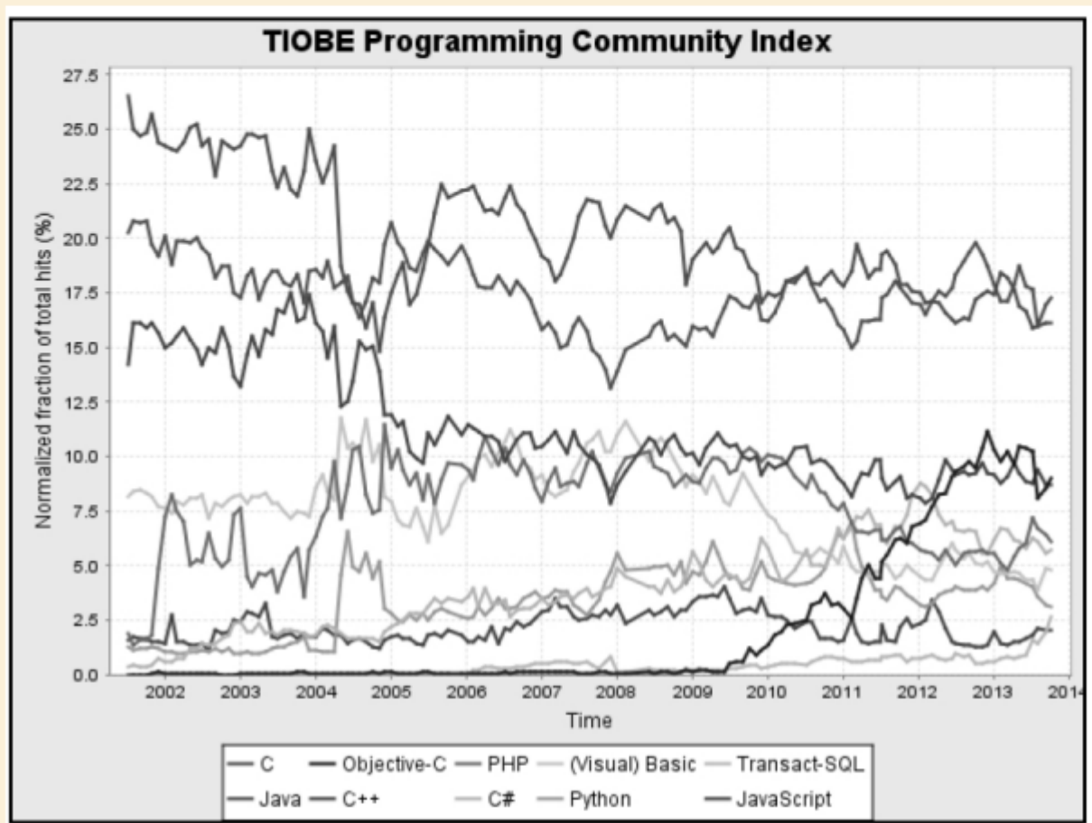
图1-1 TIOBE排行榜
