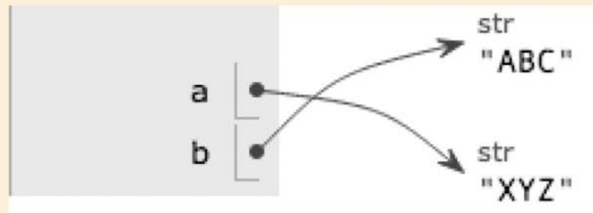
图2-5 a指向'XYZ'，b不变
