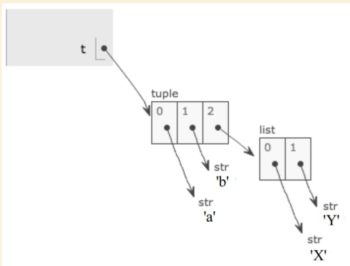
图3-2 元组“修改”
