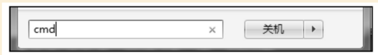
图1-12 输入cmd
