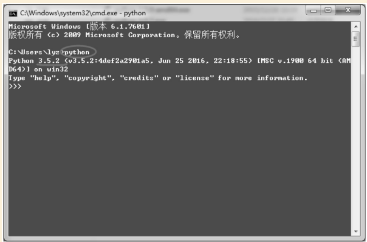
图1-14 Python命令
