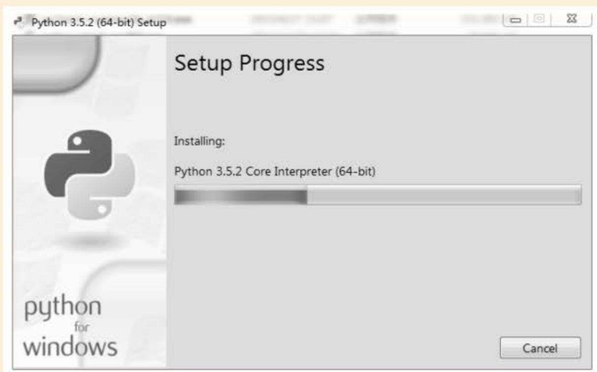
图1-9 安装进行中
