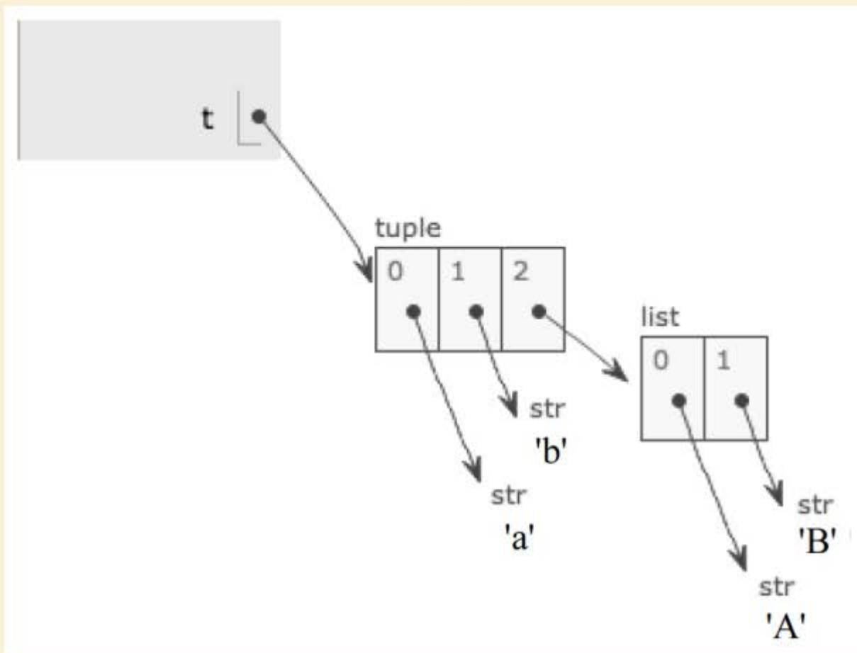
图3-1 元组定义
