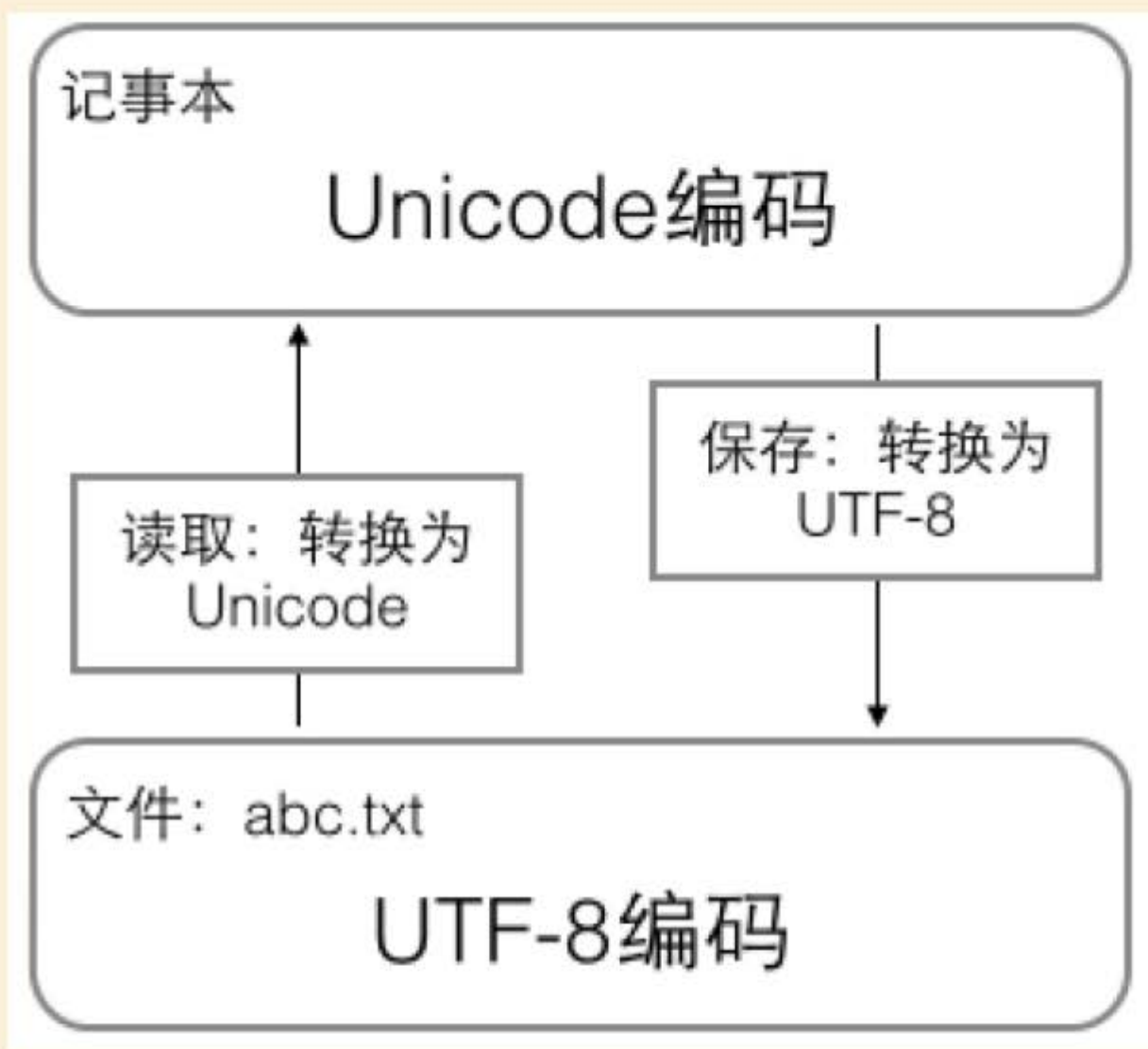
图2-8 字符转换
