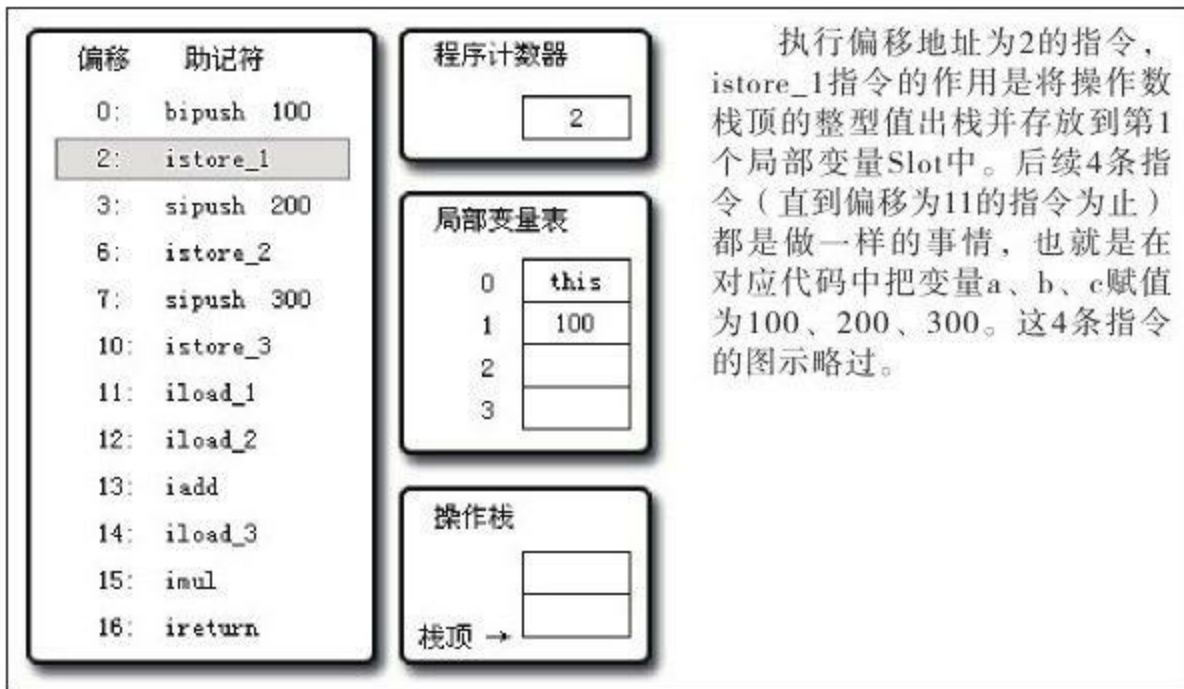
图 8-6 执行偏移地址为1的指令的情况
