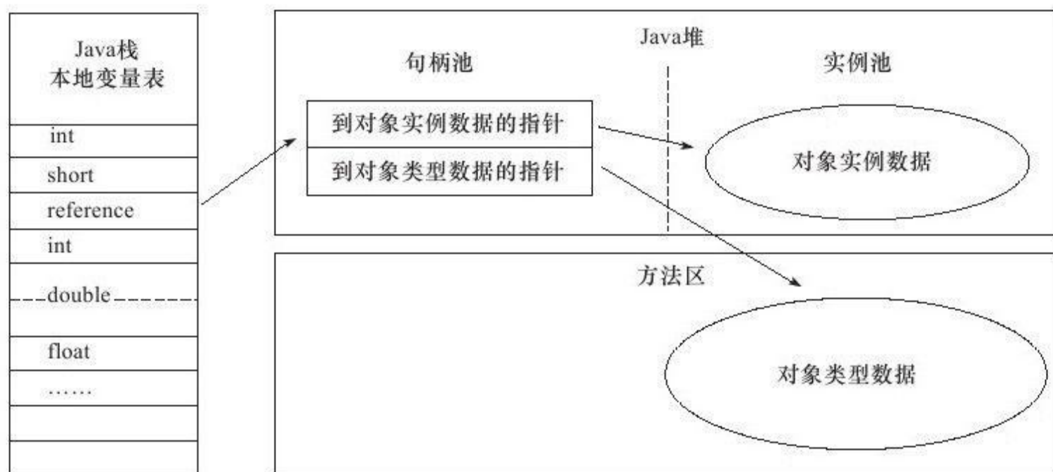
图 2-2 通过句柄访问对象
