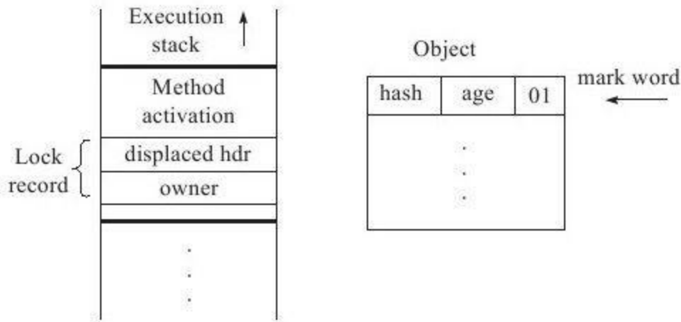
图 13-3 轻量级锁CAS操作之前堆栈与对象的状态 [1]
