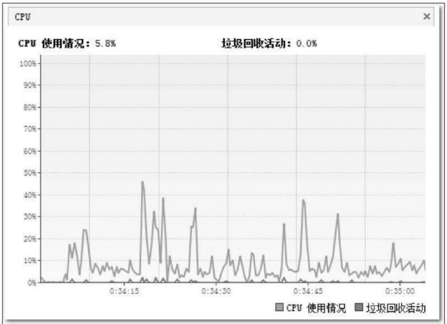
图 5-12 编译期间CPU曲线
