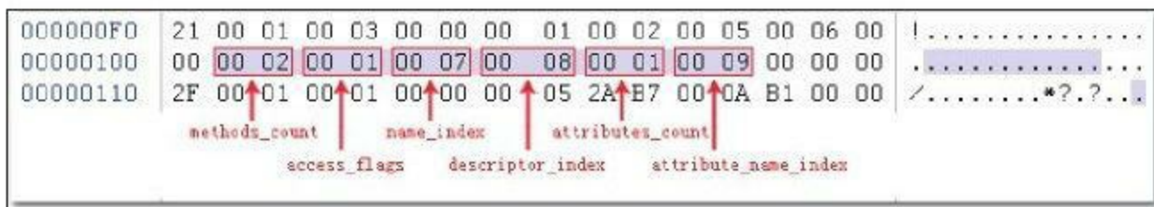
图 6-9 方法表结构实例
