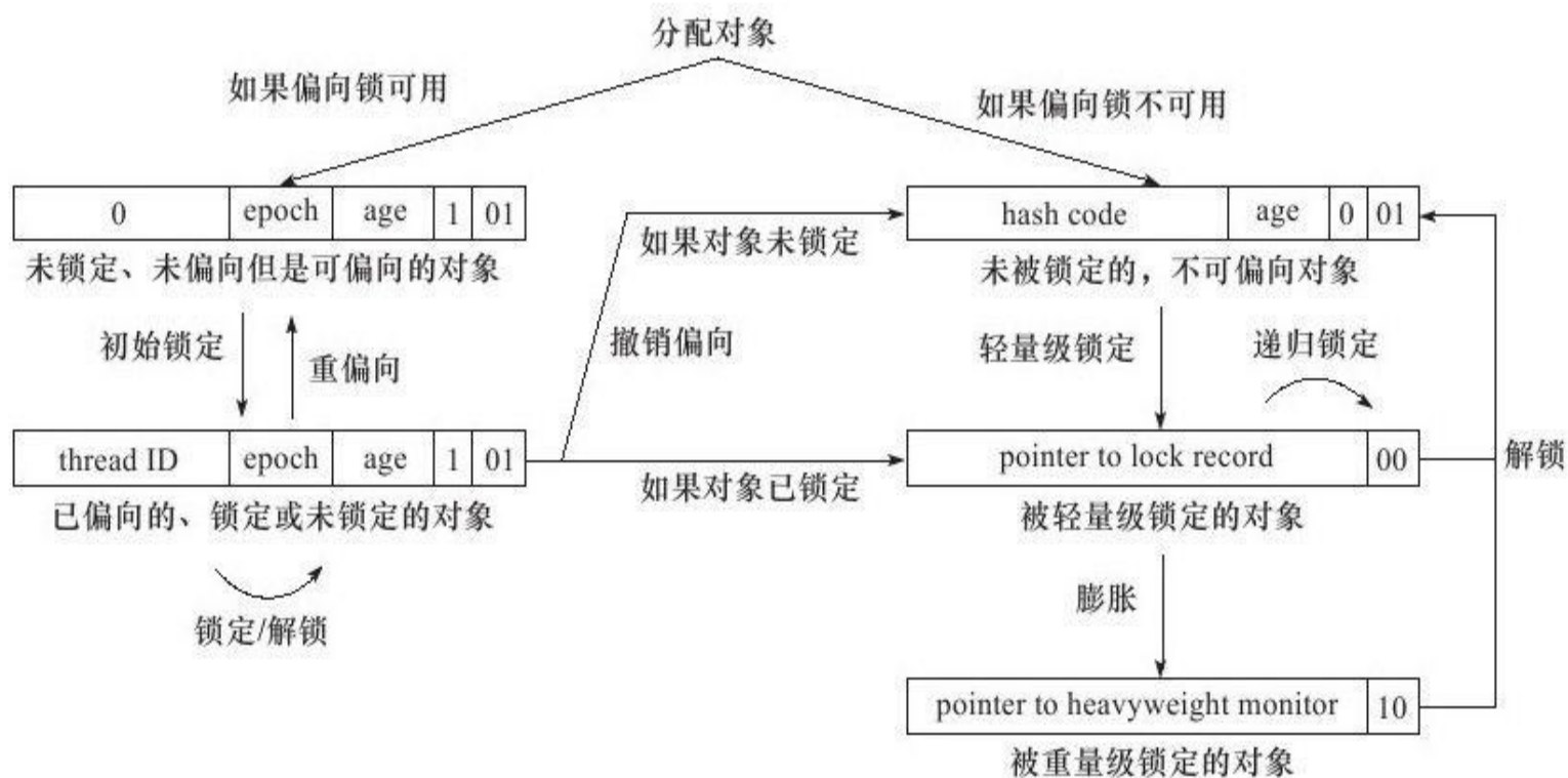
图 13-5 偏向锁、轻量级锁的状态转化及对象Mark Word的关系
