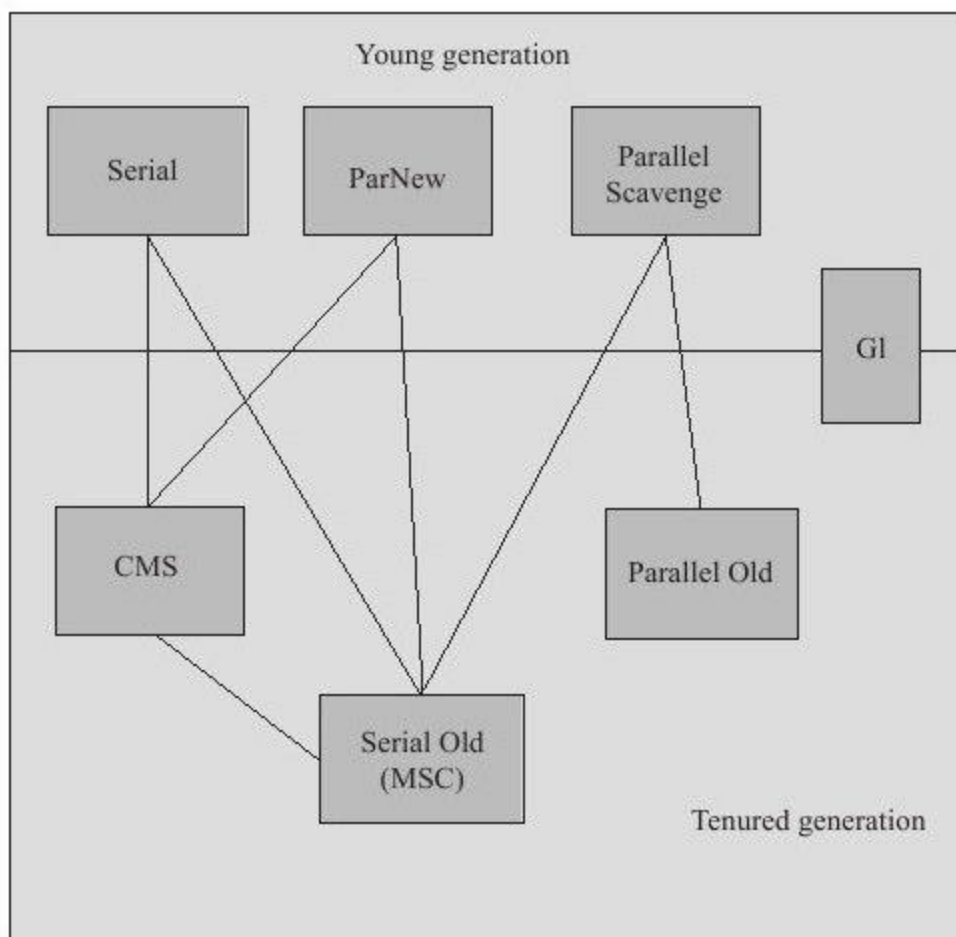
图 3-5 HotSpot虚拟机的垃圾收集器
