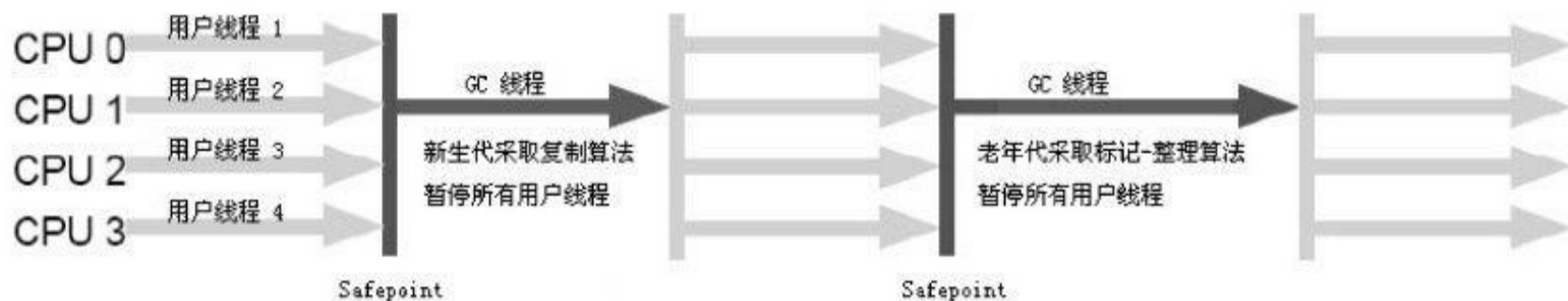
图 3-8 Serial/Serial Old收集器运行示意图
