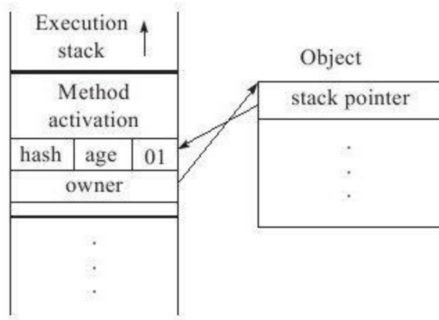
图 13-4 轻量级锁CAS操作之后堆栈与对象的状态
