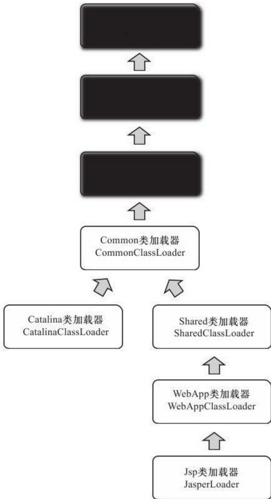
图 9-1 Tomcat服务器的类加载架构
