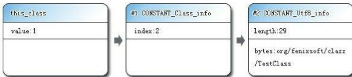
图 6-6 类索引查找全限定名的过程
