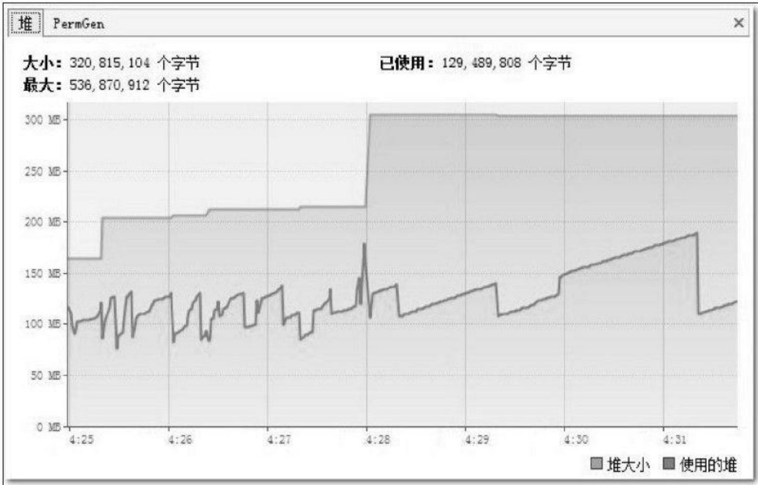
图 5-6 Java堆监视曲线
