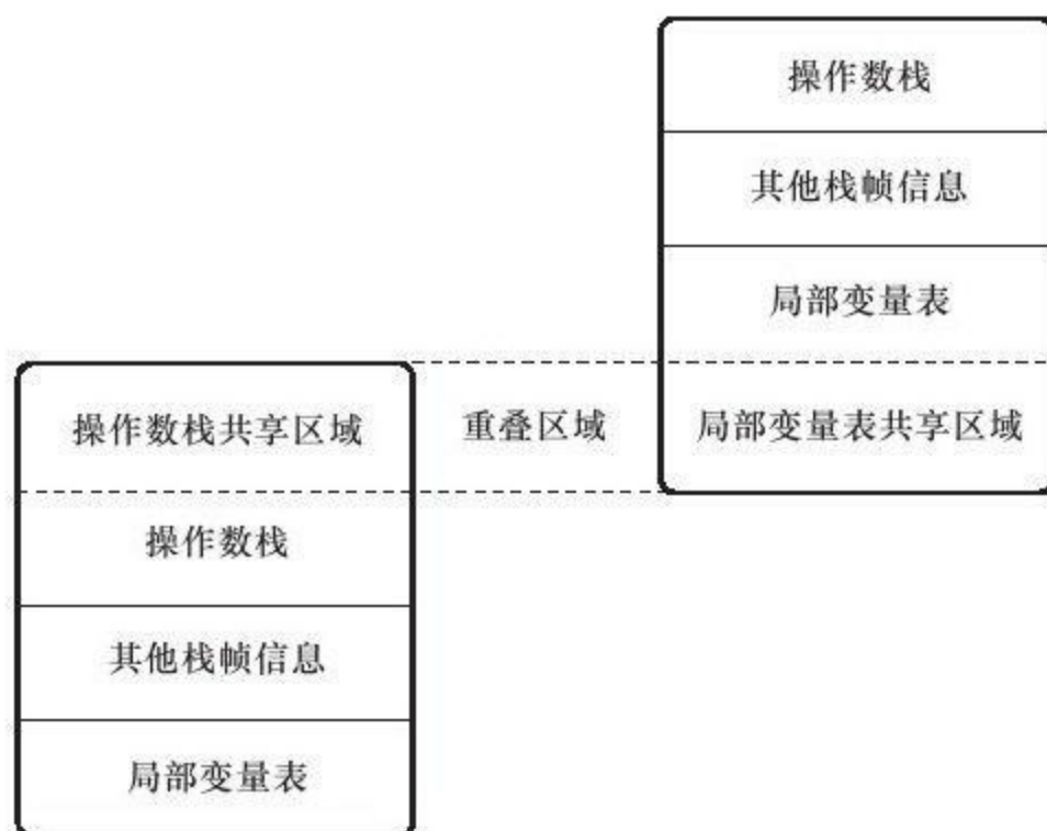
图 8-2 两个栈帧之间的数据共享
