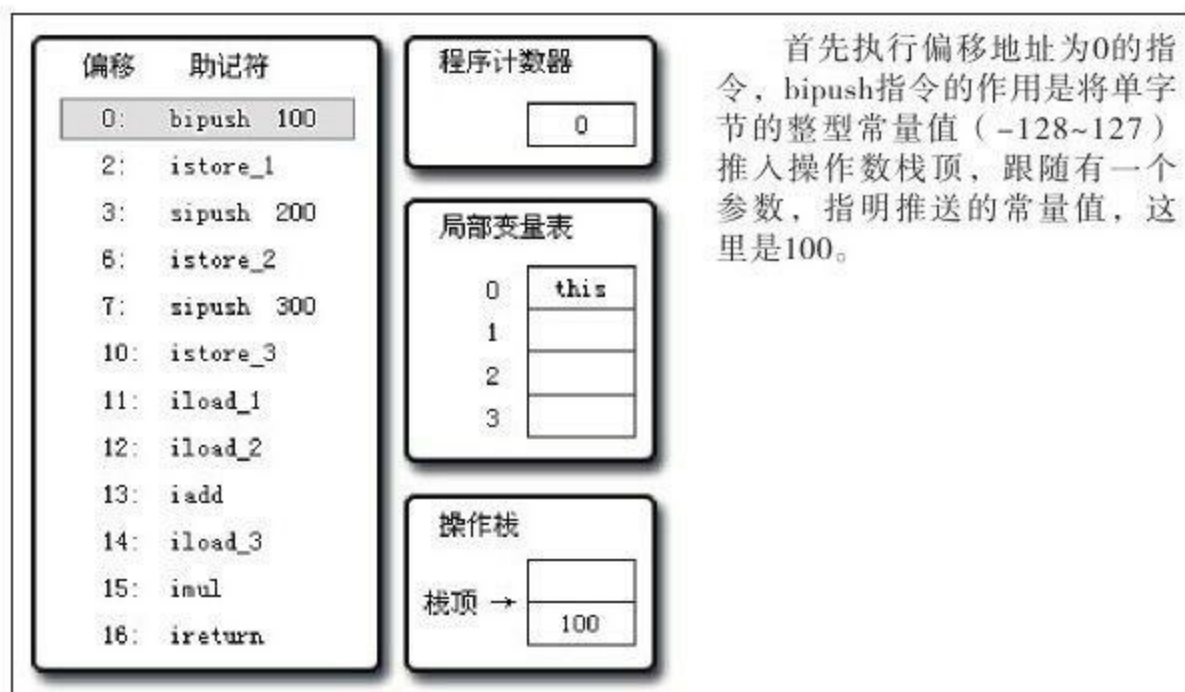
图 8-5 执行偏移地址为0的指令的情况
