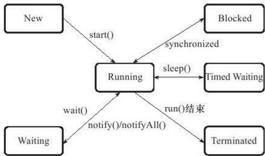
图 12-6 线程状态转换关系
