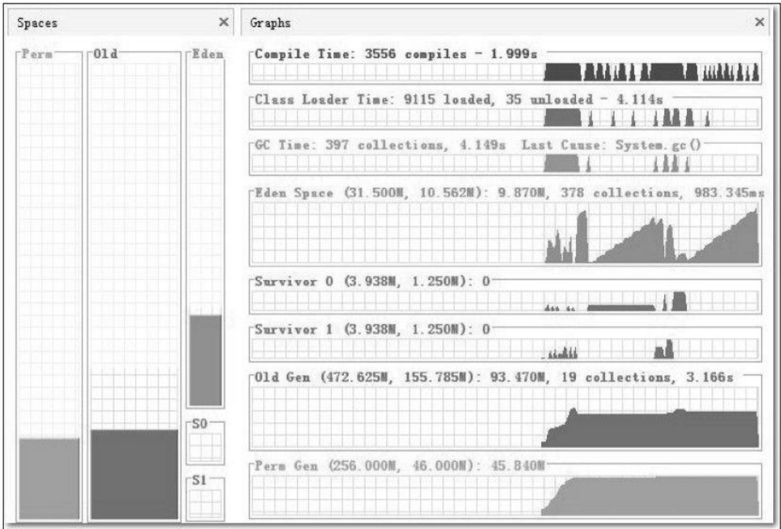
图 5-2 Eclipse原始运行数据
