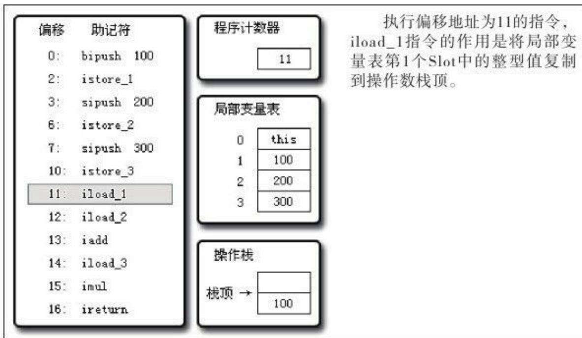
图 8-7 执行偏移地址为11的指令的情况
