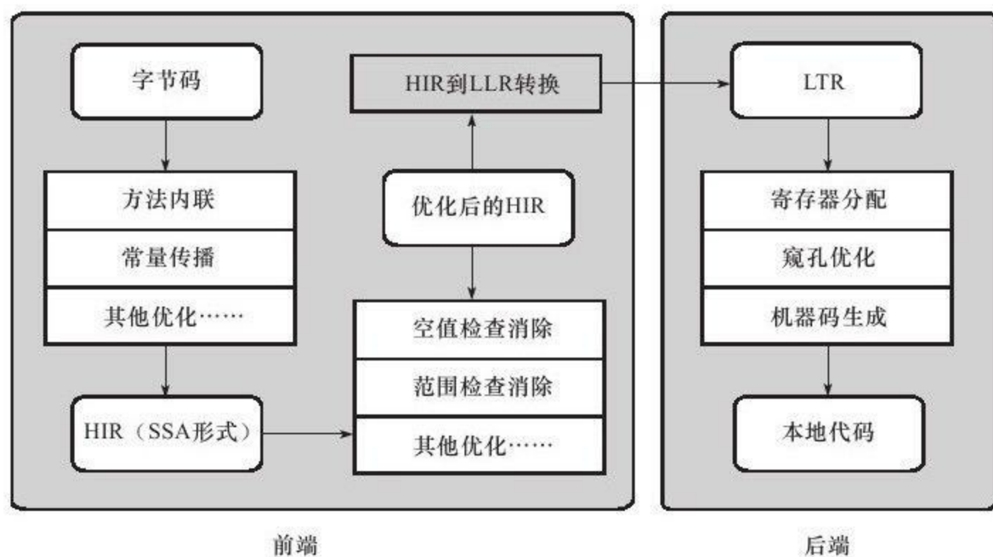
图 11-4 Client Compiler架构
