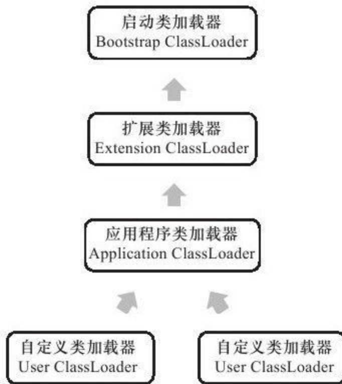
图 7-2 类加载器双亲委派模型
