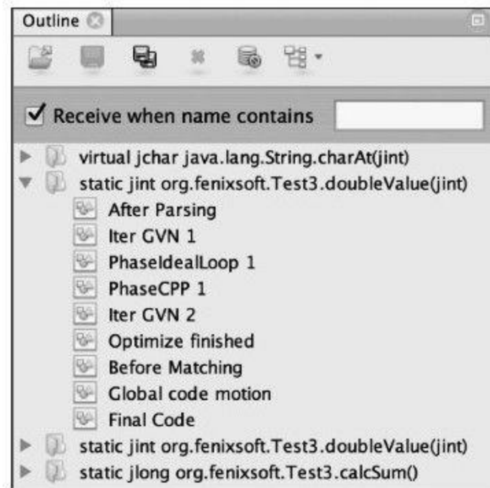
图 11-5 编译过的方法列表
