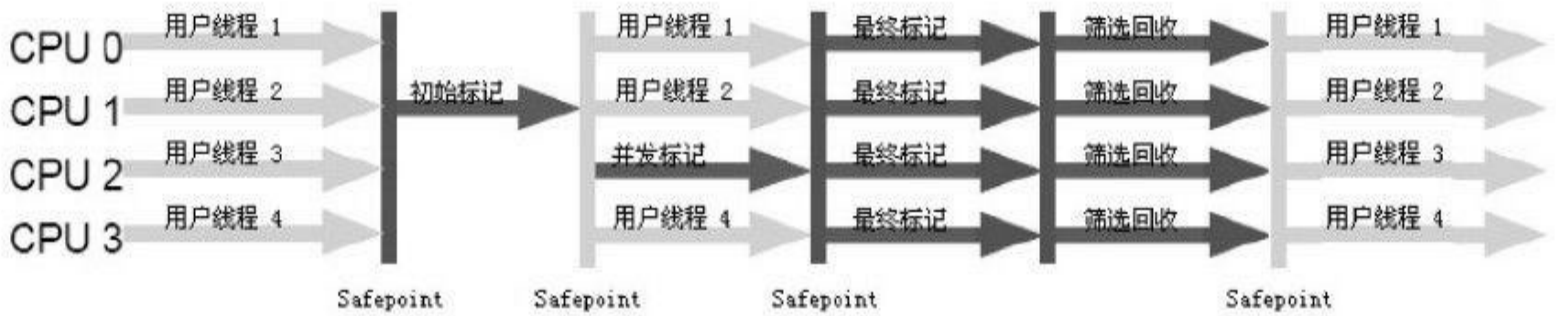
图 3-11 G1收集器运行示意图
