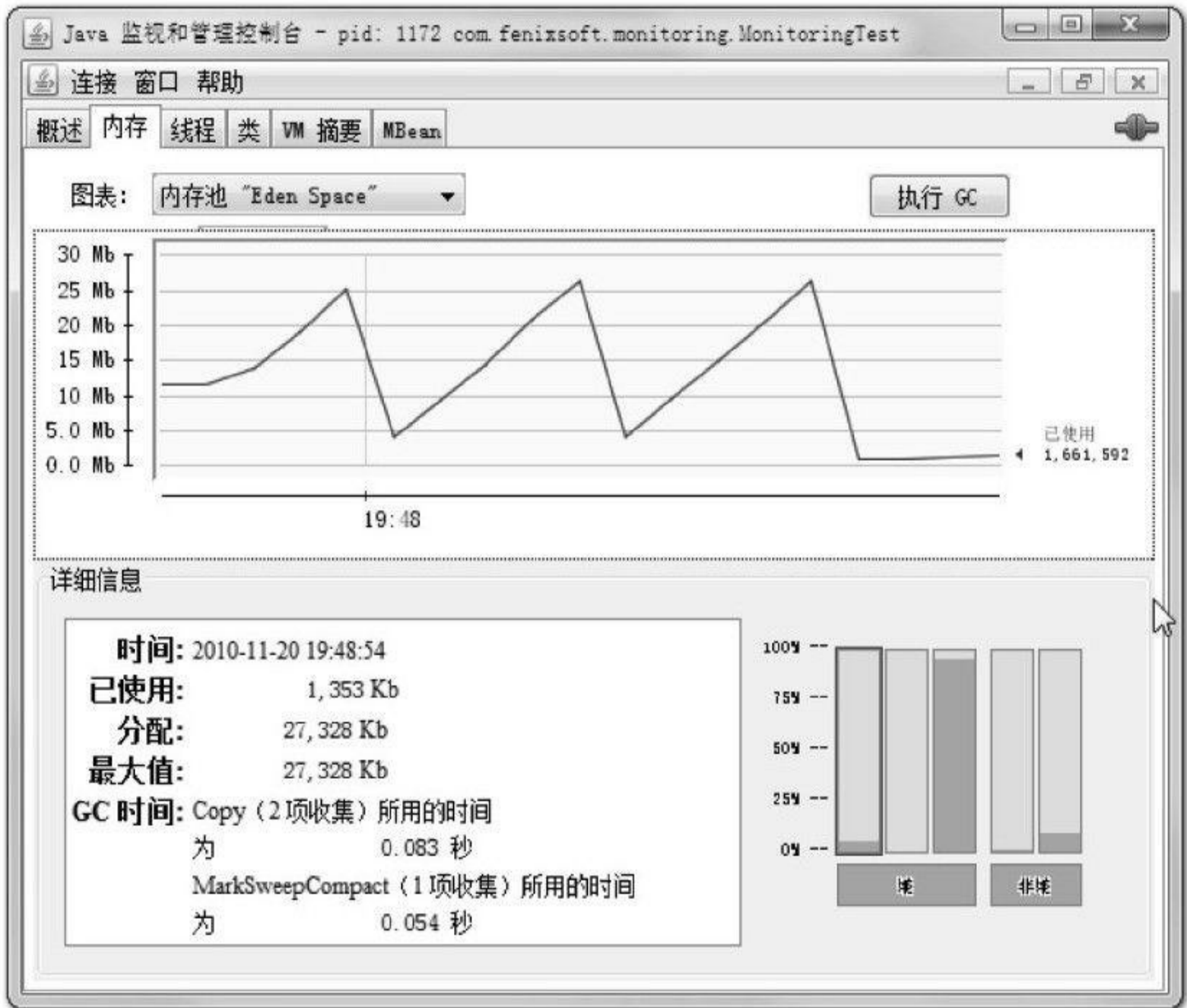
图 4-6 Eden区内存变化状况
