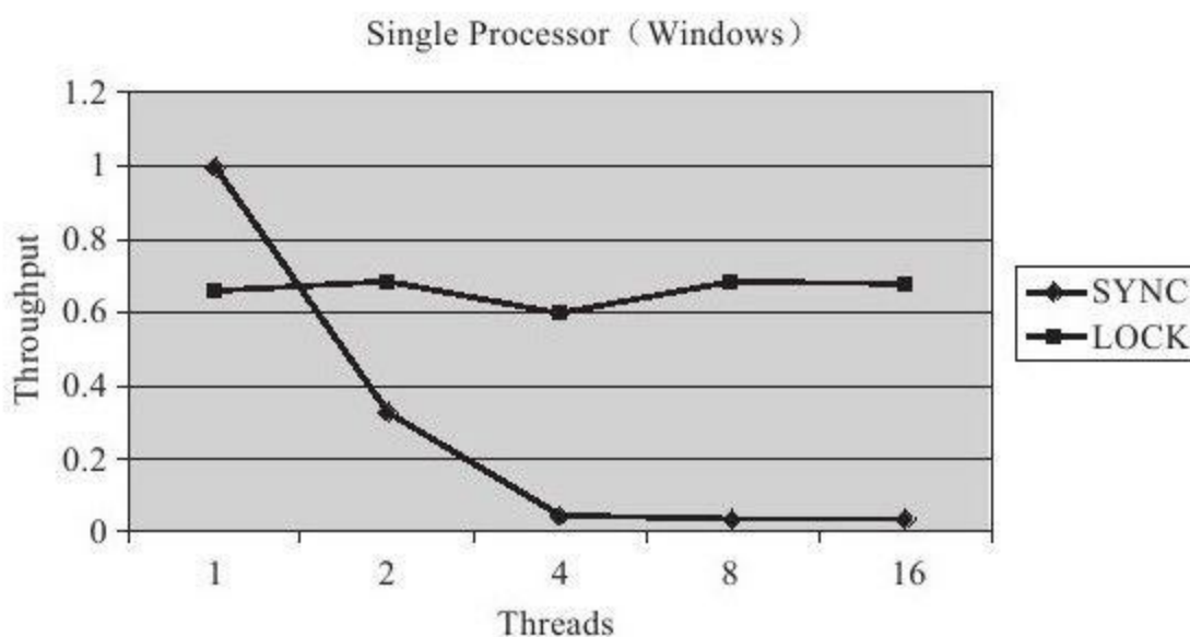
图 13-1 JDK 1.5、单核处理器下两种锁的吞吐量对比
