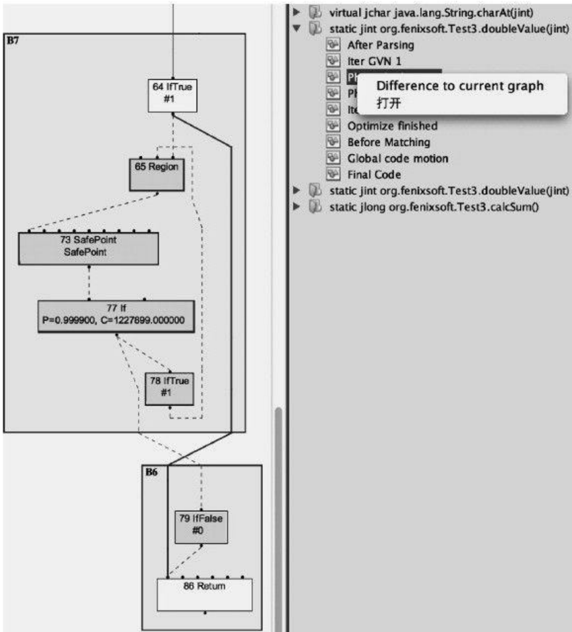
图 11-8 基本块图示 ( 3 )
