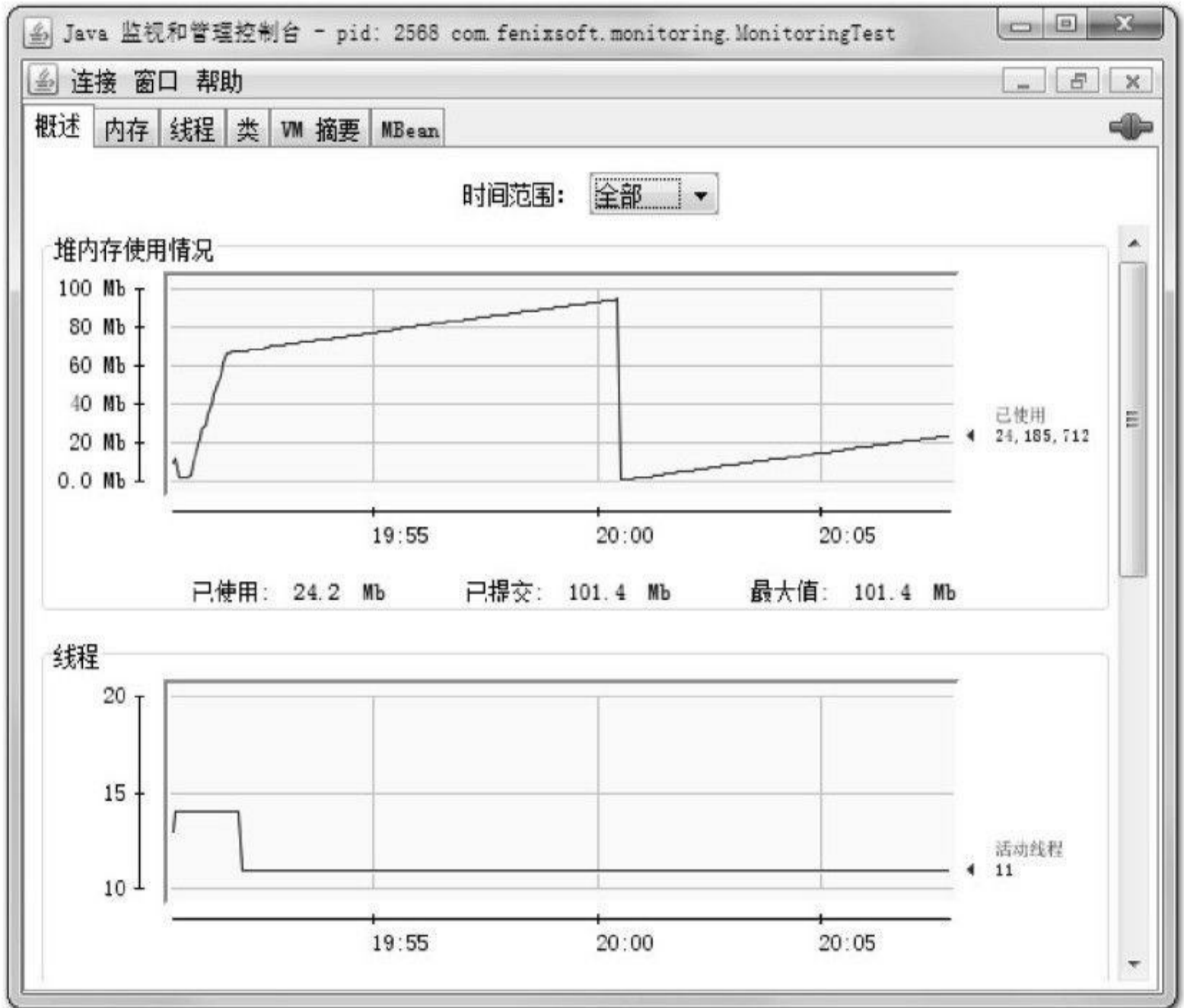
图 4-5 JConsole主界面
