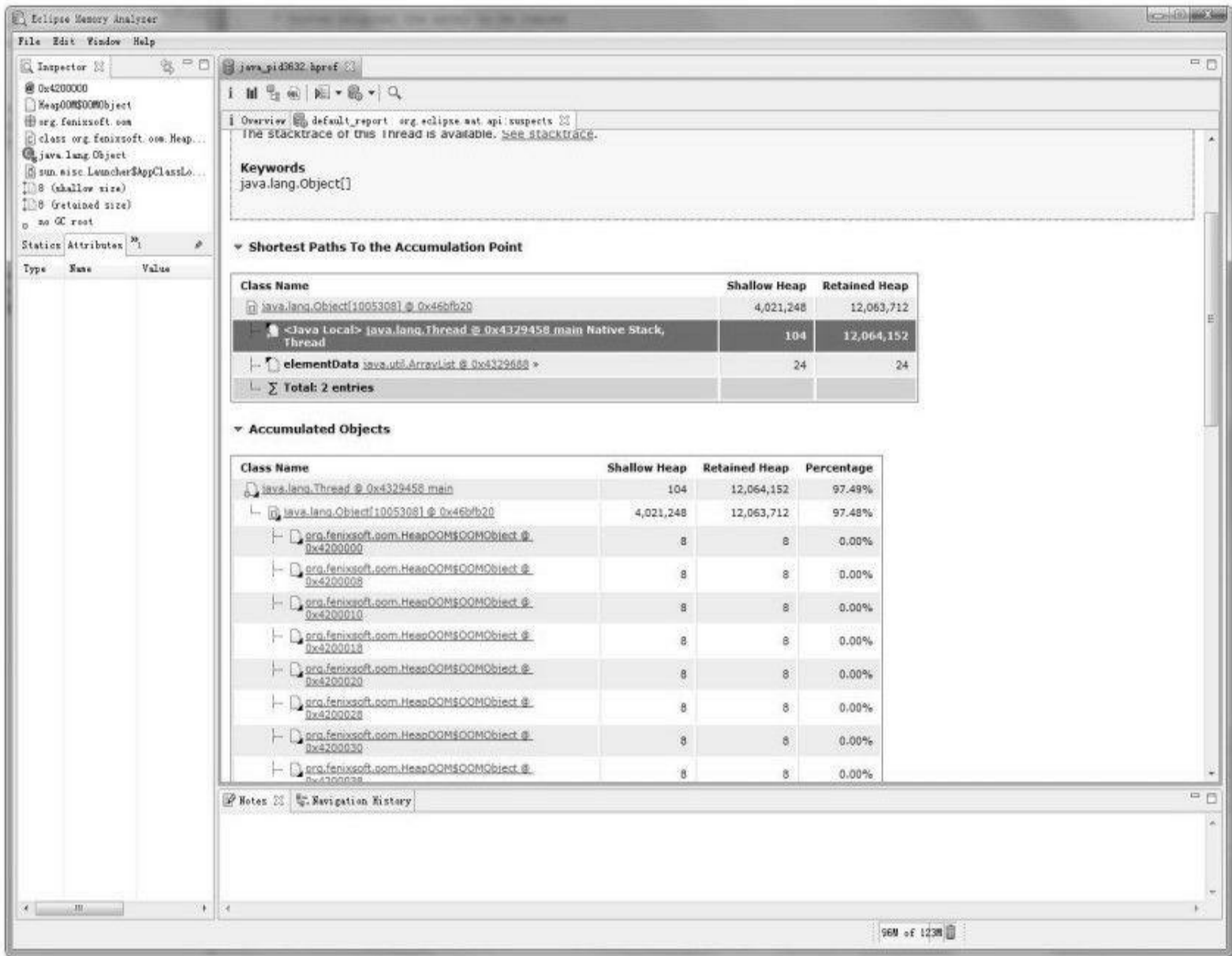
图 2-5 使用Eclipse Memory Analyzer打开的堆转储快照文件
