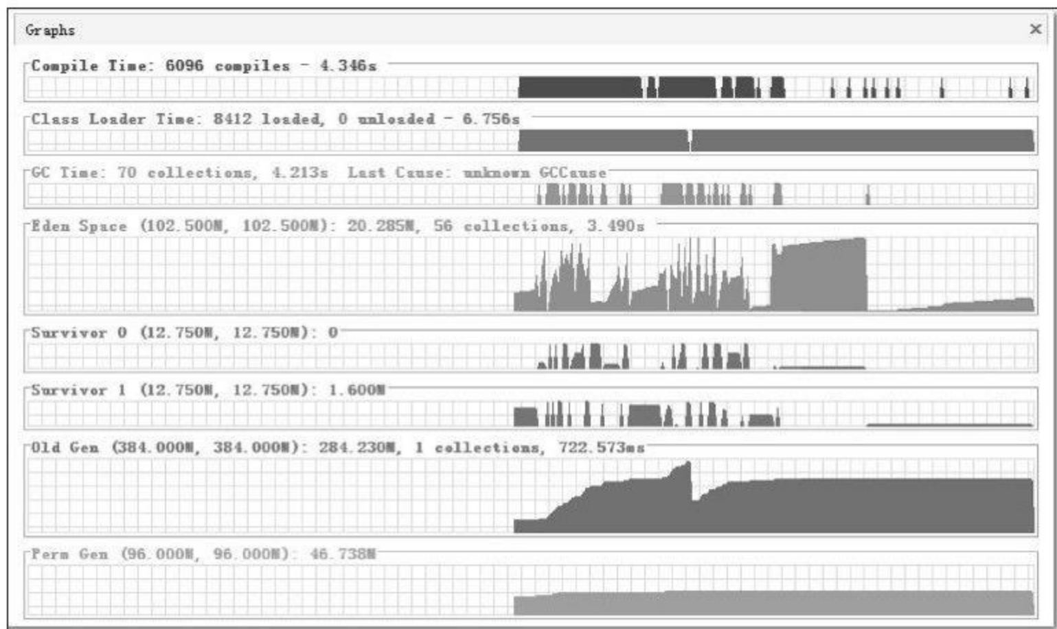
图 5-11 编译期间运行数据
