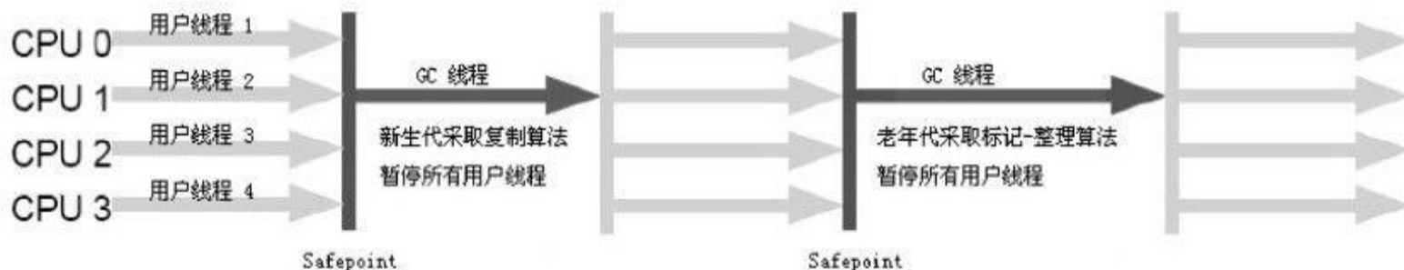
图 3-6 Serial/Serial Old收集器运行示意图
