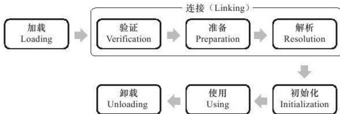
图 7-1 类的生命周期
