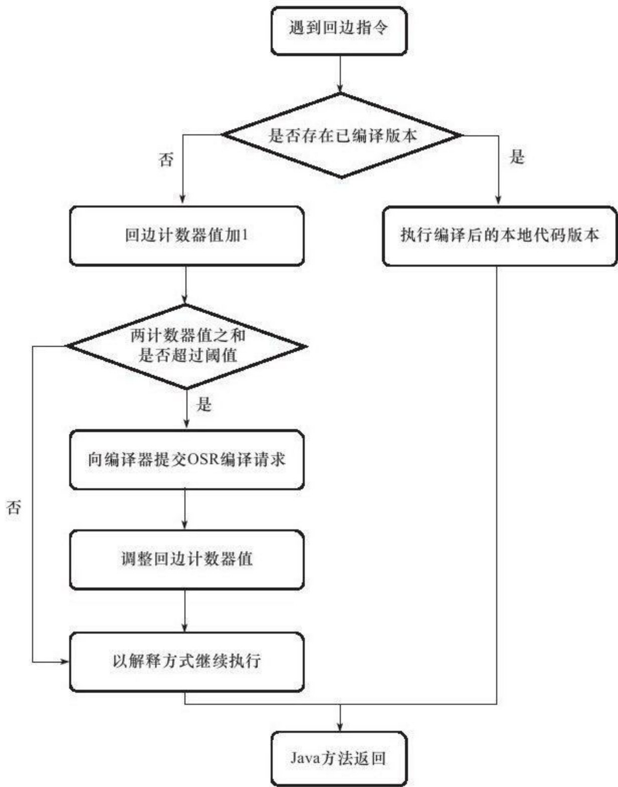
图 11-3 回边计数器触发即时编译
