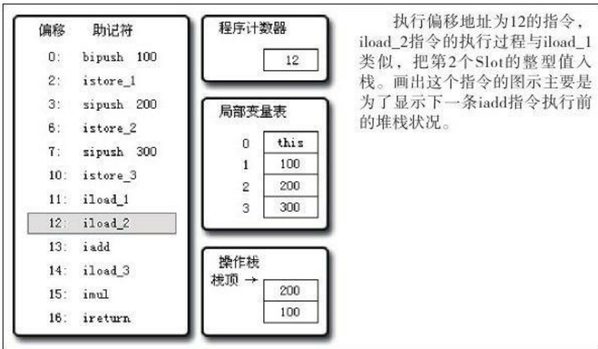
图 8-8 执行偏移地址为12的指令的情况
