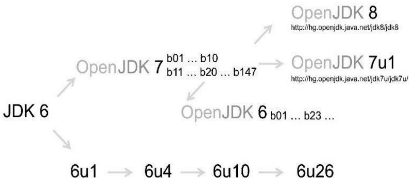
图 1-7 OpenJDK 6、OpenJDK 7、OpenJDK 7u、OpenJDK 8之间的关系
