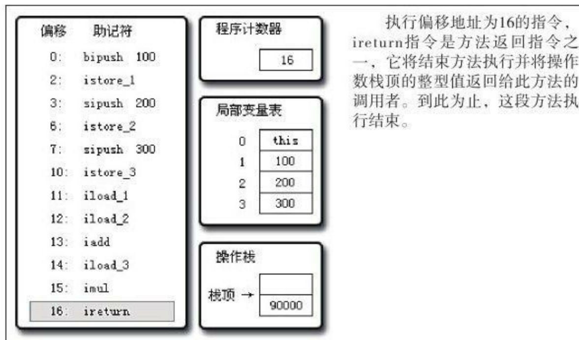
图 8-11 执行偏移地址为16的指令的情况
