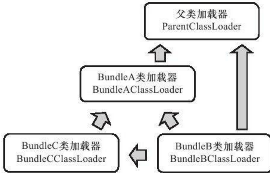
图 9-2 OSGi的类加载器架构
