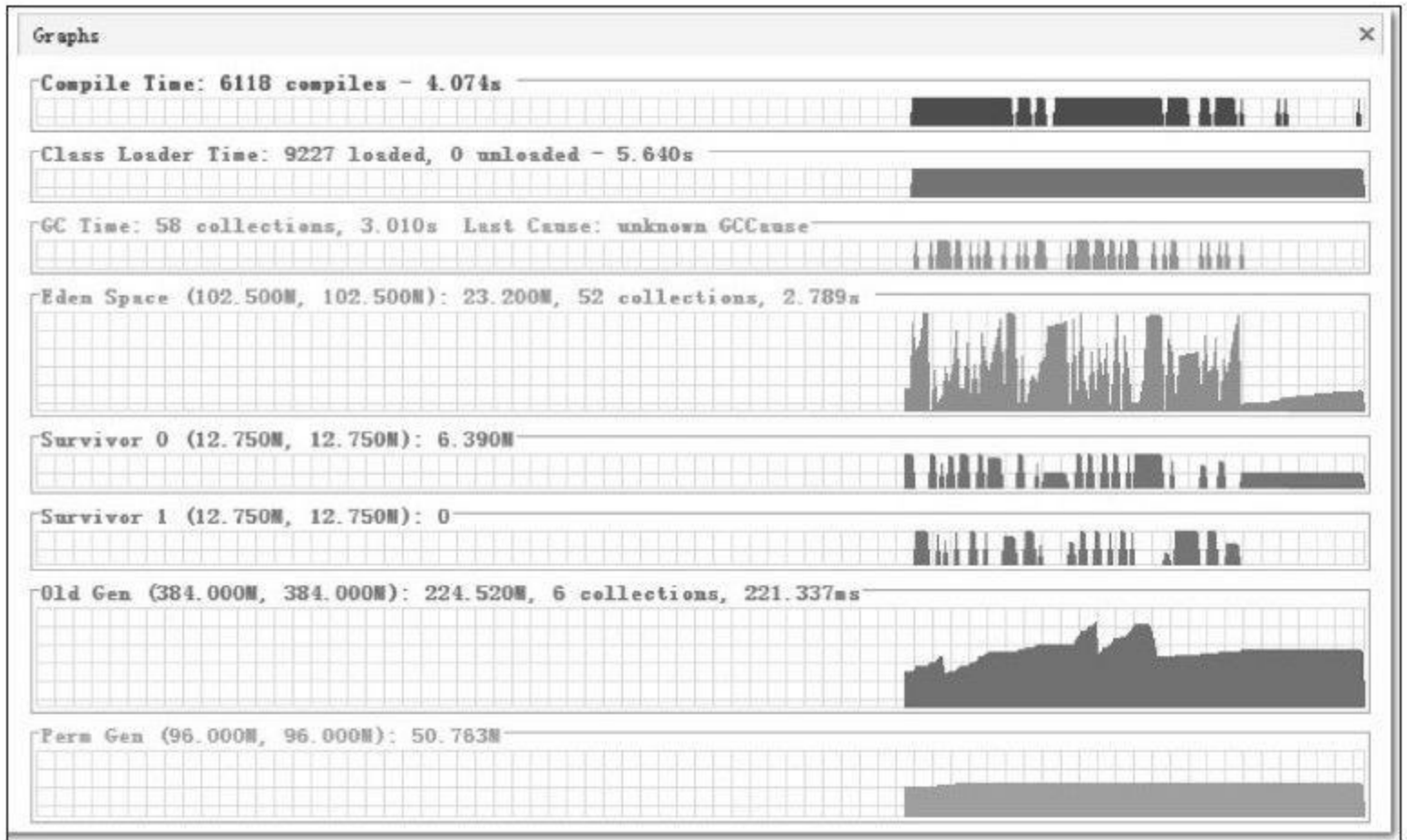
图 5-13 指定ParNew和CMS收集器后的GC数据
