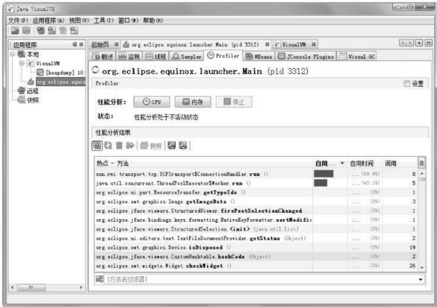
图 4-15 对应用程序进行CPU执行时间分析
