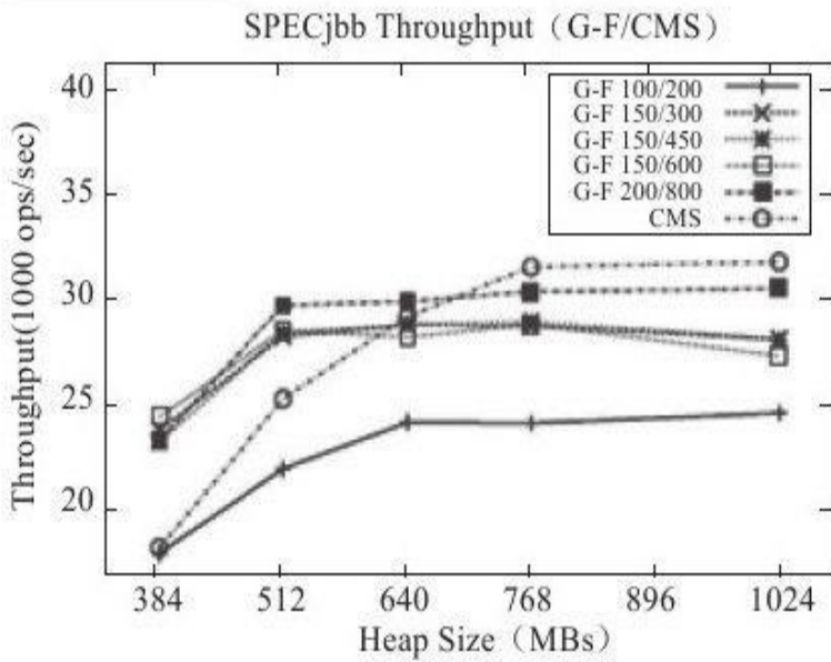
图 3-12 吞吐量测试结果
