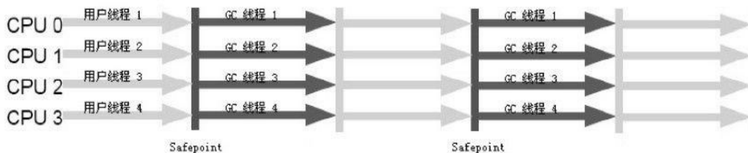
图 3-9 Parallel Scavenge/Parallel Old收集器运行示意图
