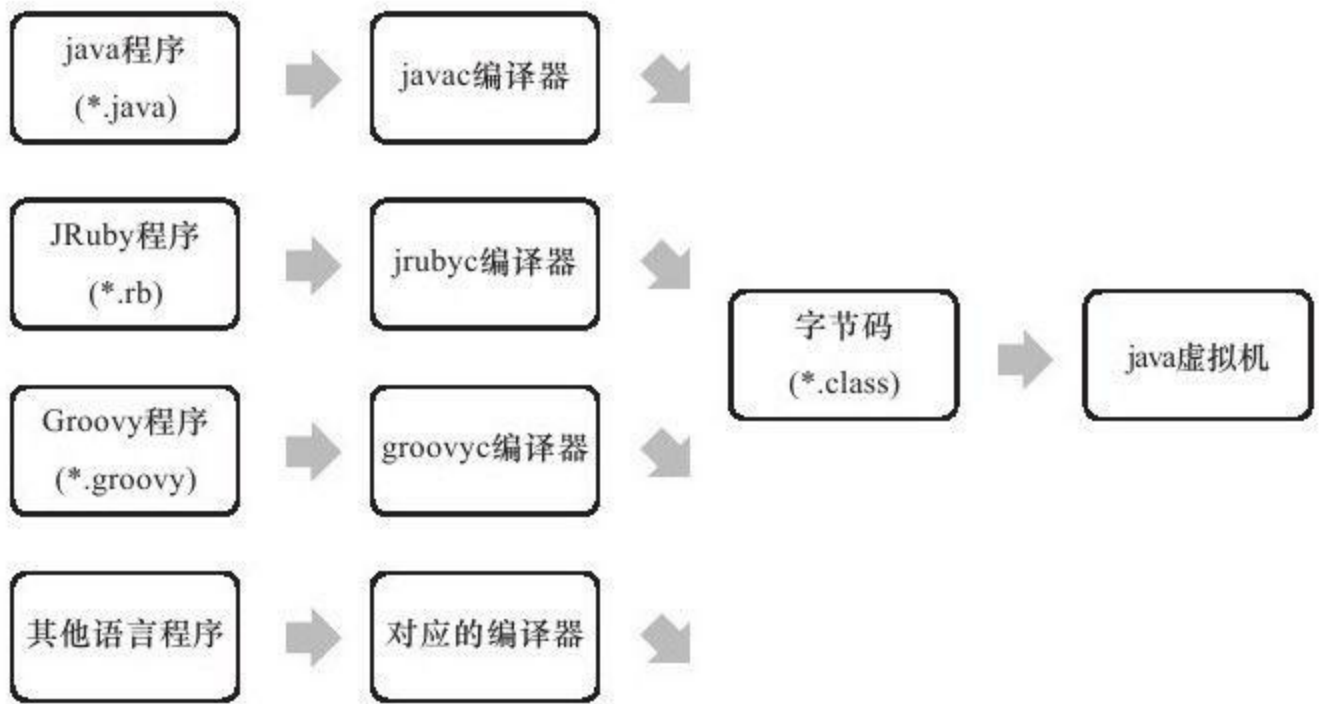
图 6-1 Java虚拟机提供的语言无关性
