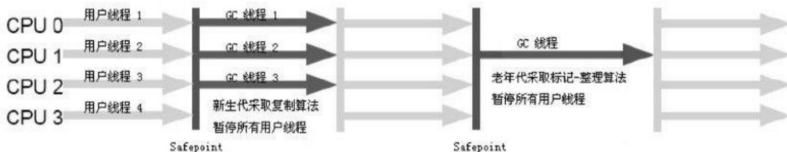
图 3-7 ParNew/Serial Old收集器运行示意图
