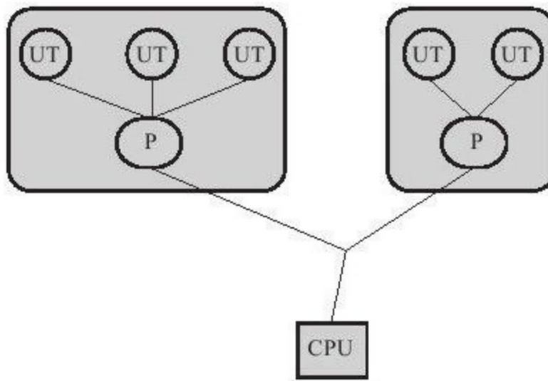
图 12-4 进程与用户线程之间1：N的关系
