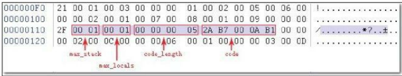
图 6-10 Code属性结构实例
