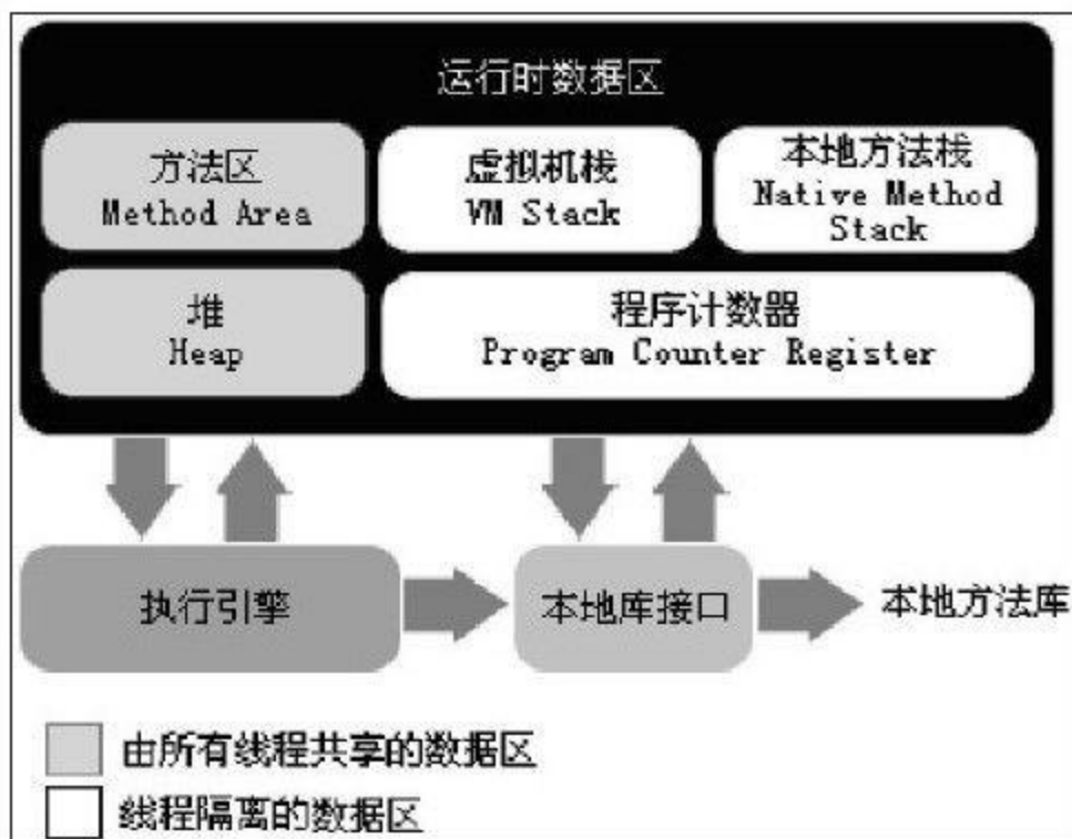
图 2-1 Java虚拟机运行时数据区
