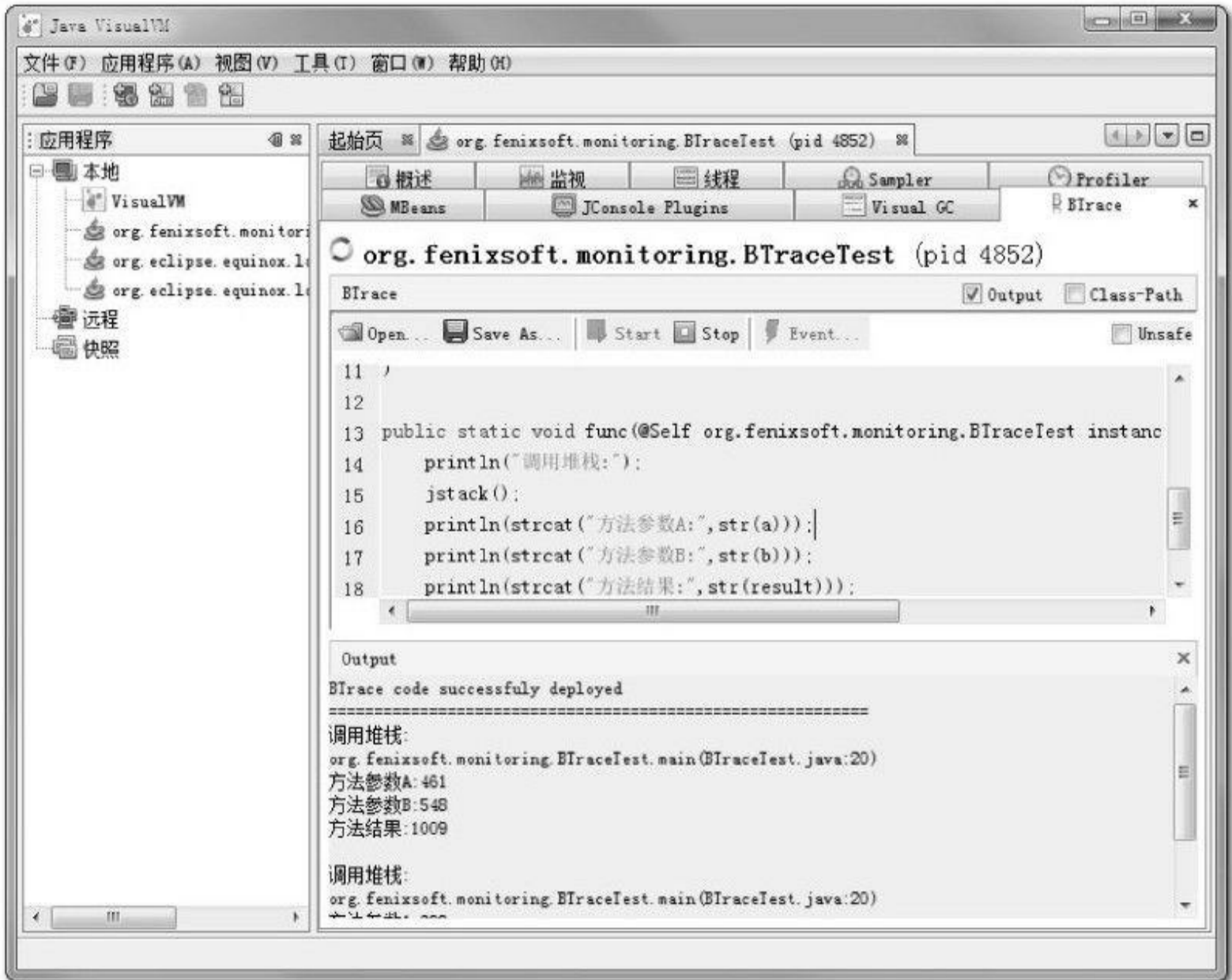
图 4-17 BTrace跟踪结果
