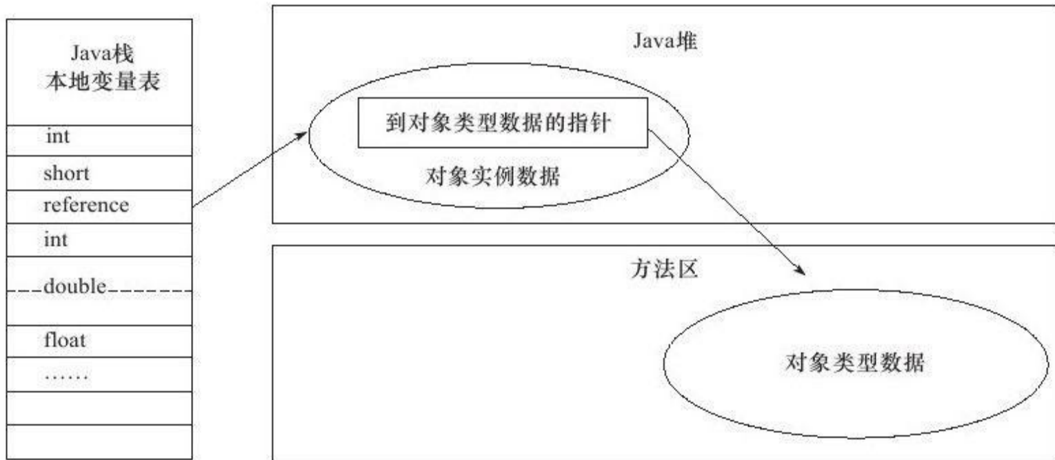
图 2-3 通过直接指针访问对象
