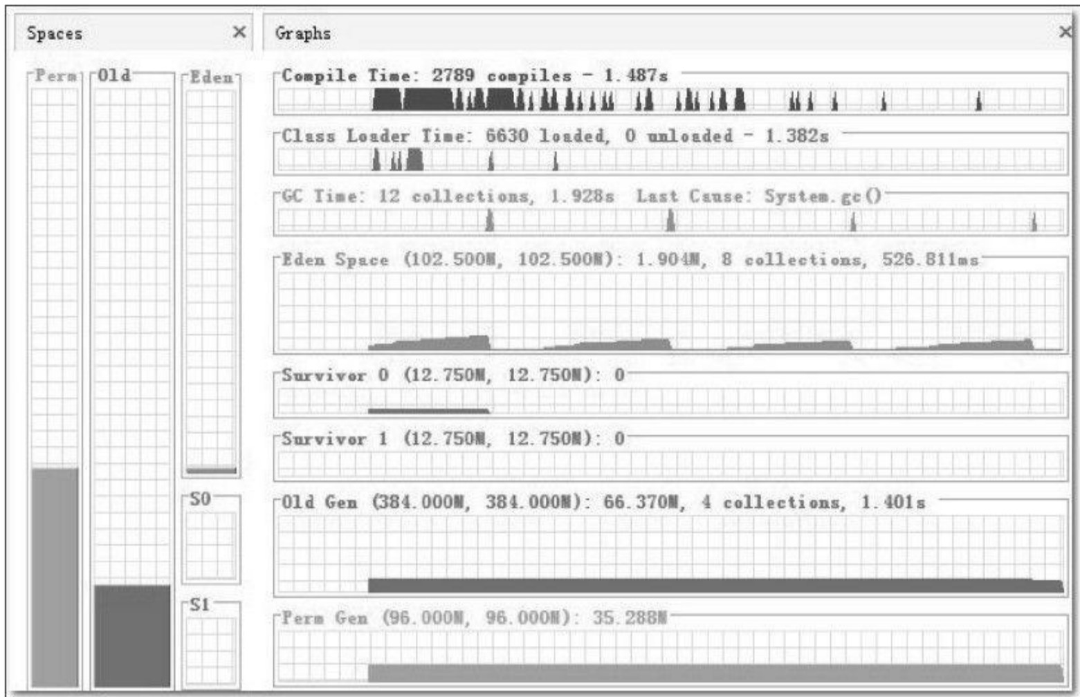
图 5-9 GC调整后的运行数据
