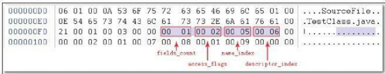
图 6-8 字段表结构实例
