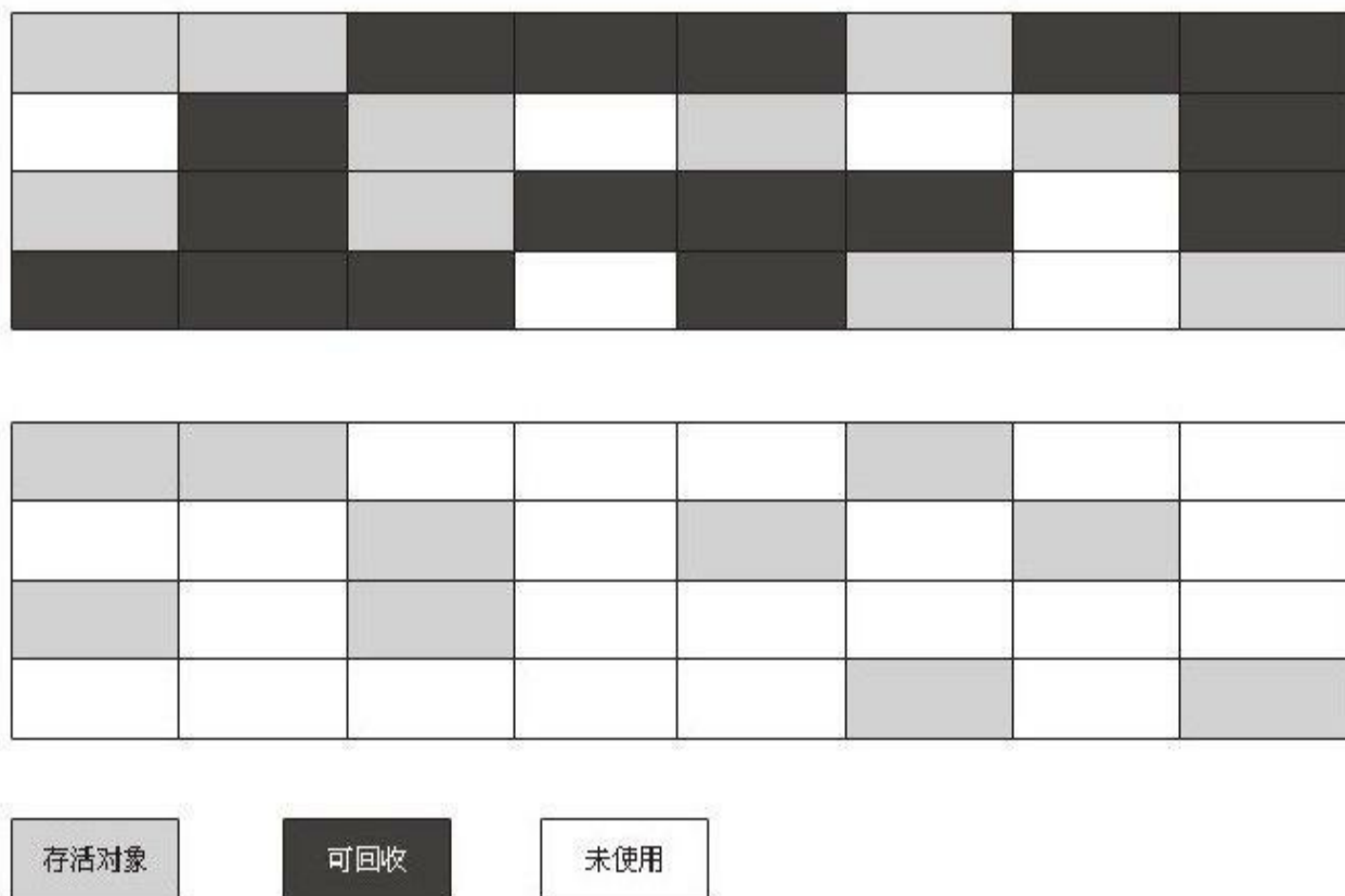
图 3-2 “标记-清除”算法示意图
