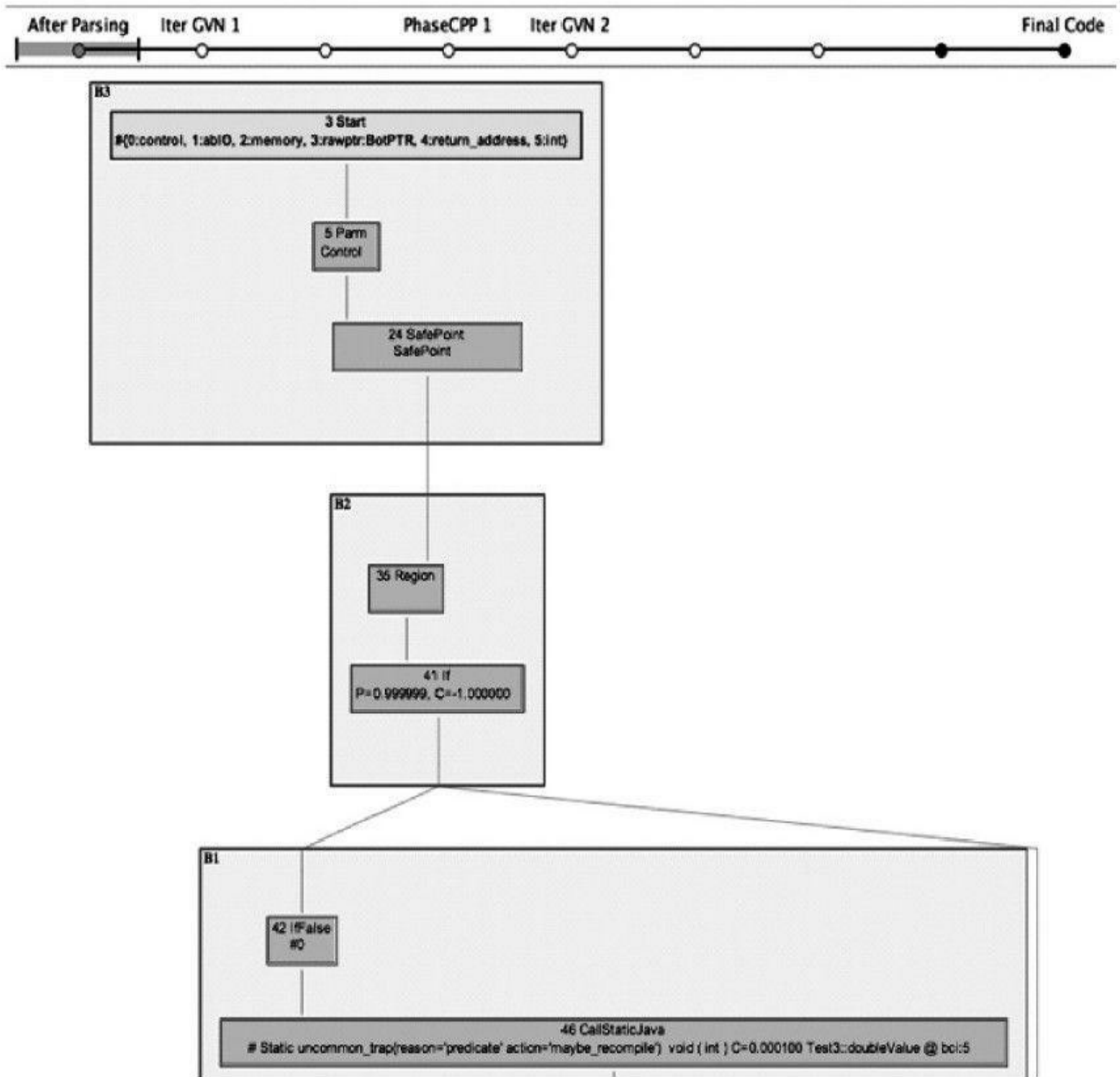
图 11-6 基本块图示 (1)
