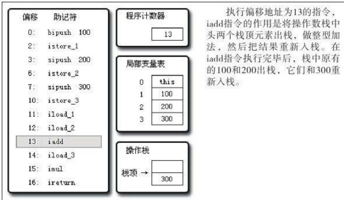
图 8-9 执行偏移地址为13的指令的情况
