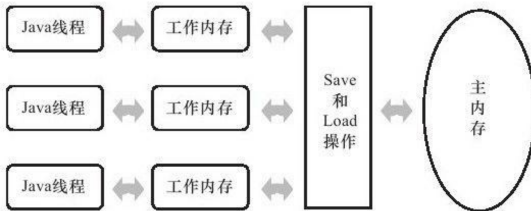
图 12-2 线程、主内存、工作内存三者的交互关系（请与图12-1对比）
