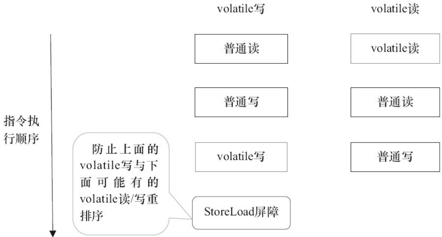
图3-22 指令序列示意图
