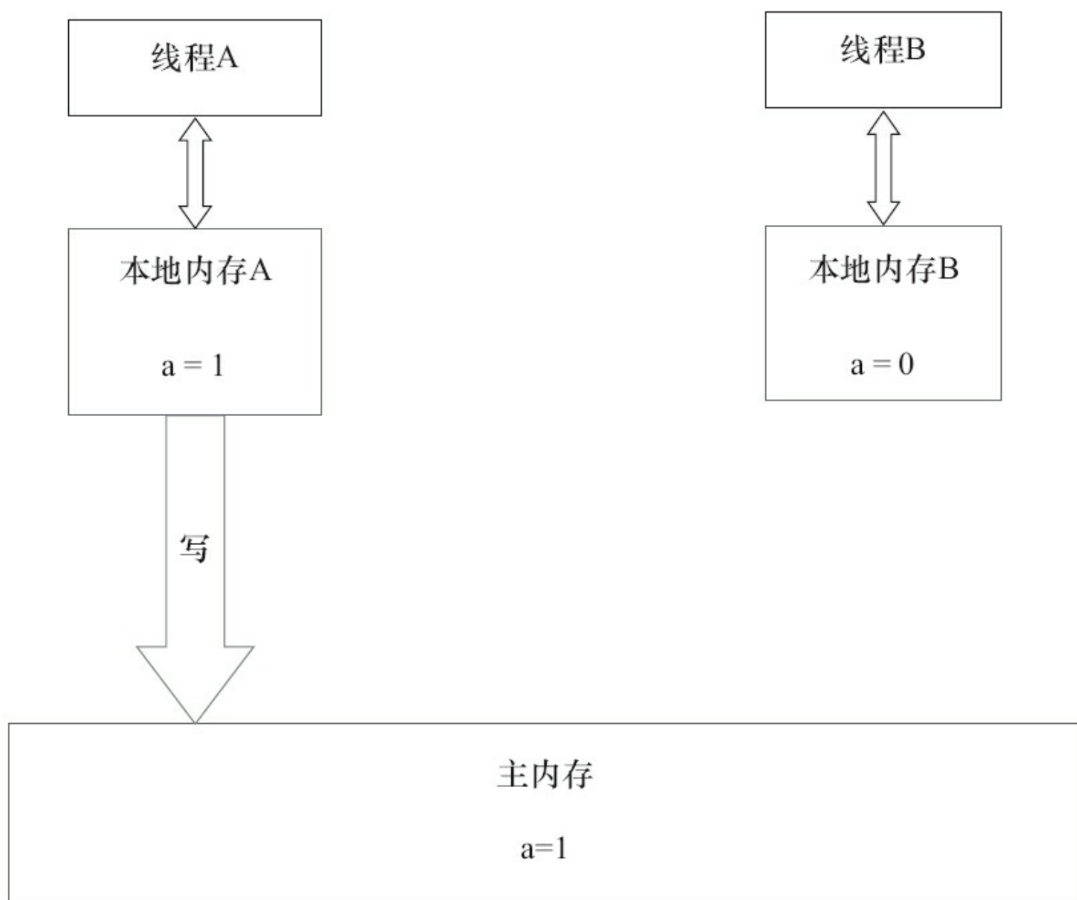
图3-25 共享数据的状态示意图
