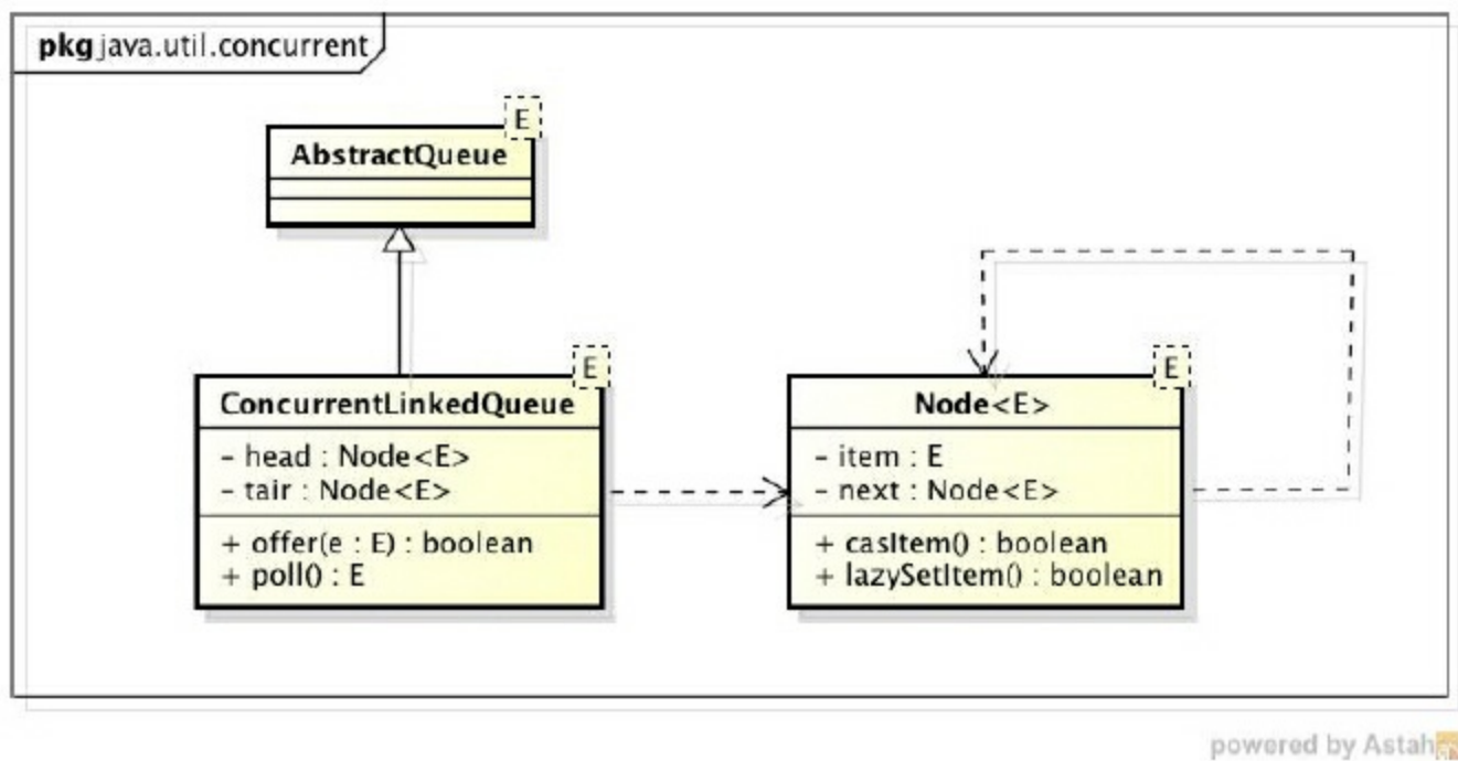
图6-3 ConcurrentLinkedQueue的类图
