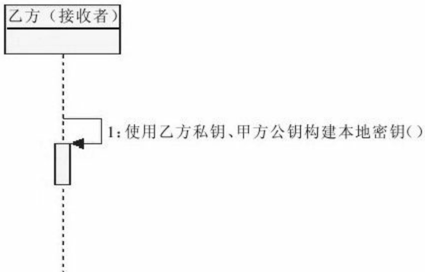
图 8-3 乙方构建DH算法本地密钥
