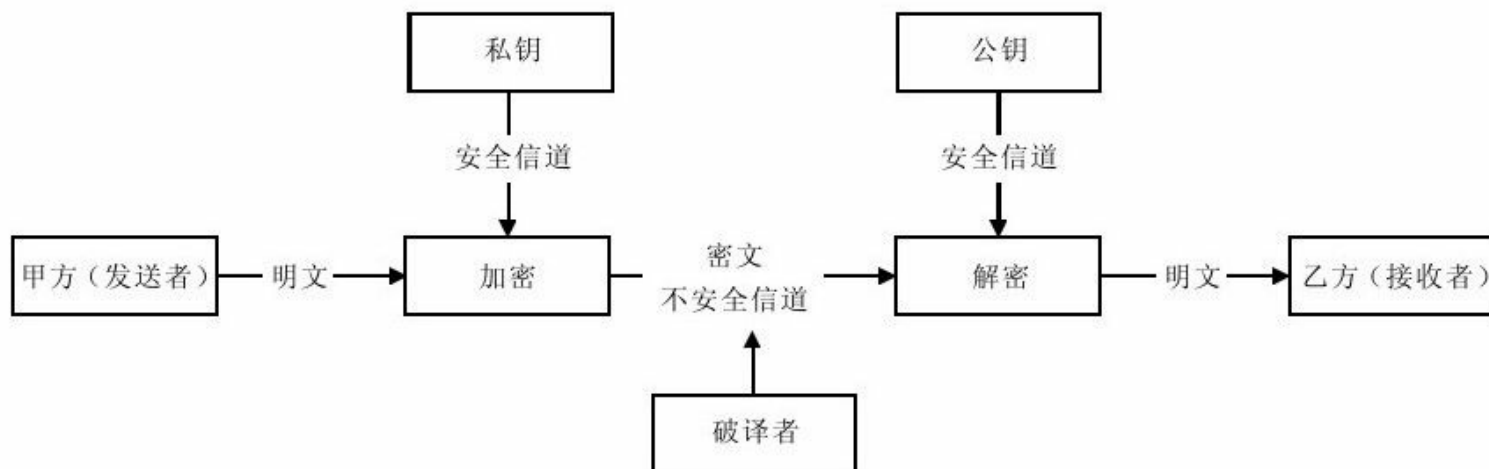
图 2-10 私钥加密-公钥解密的保密通信模型
