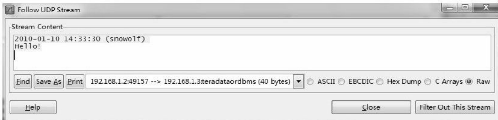
图 12-12 UDP交互内容明文
