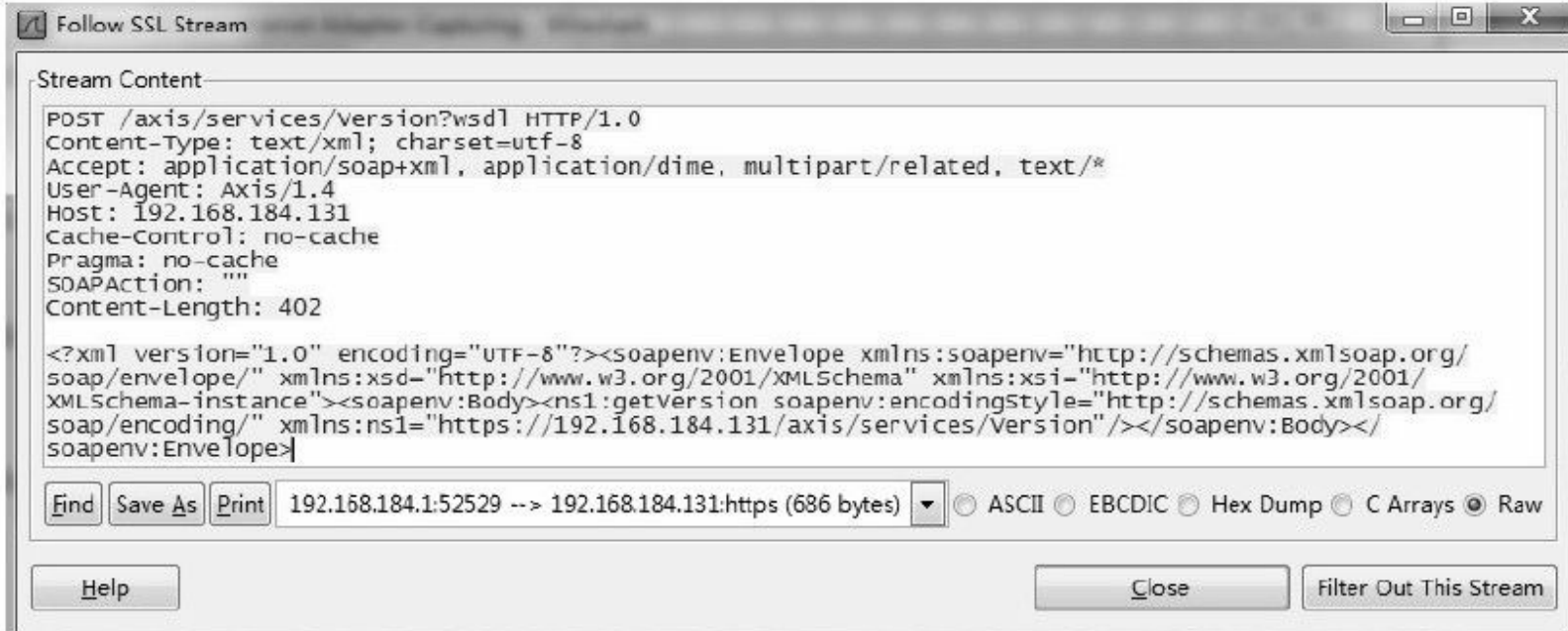
图 12-37 SOAP请求解密内容
