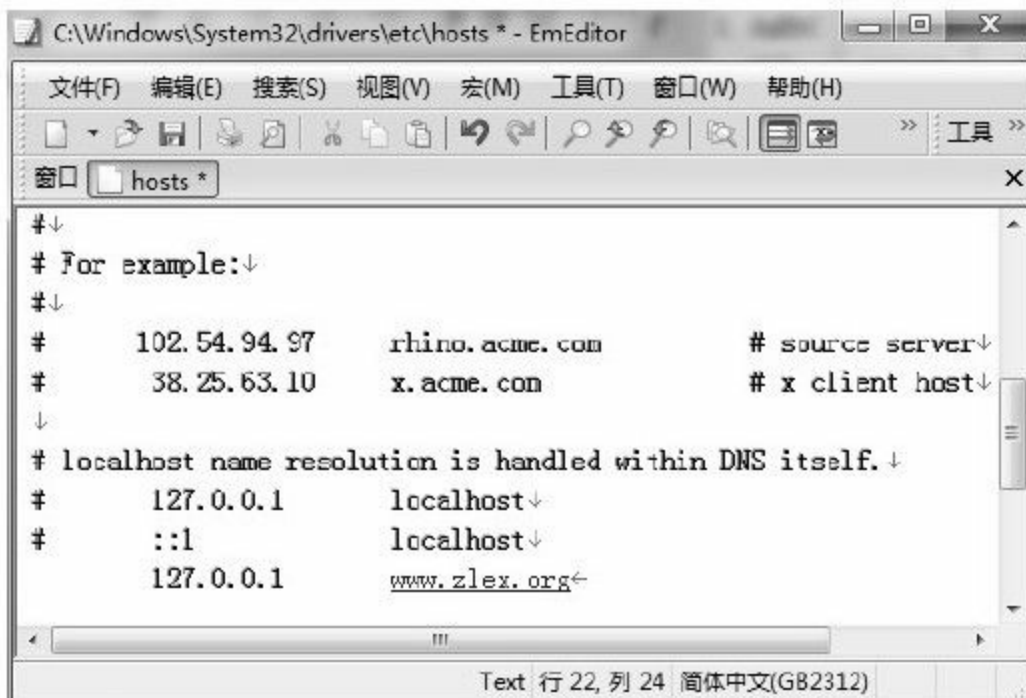
图 11-12 配置hosts文件
