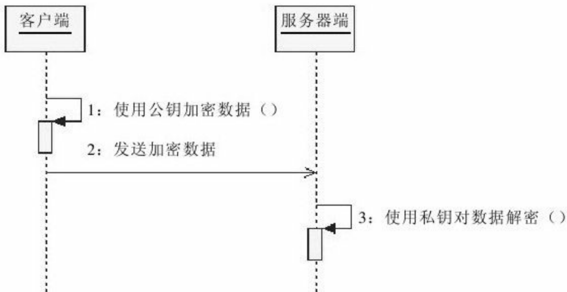
图 10-5 客户端请求服务器
