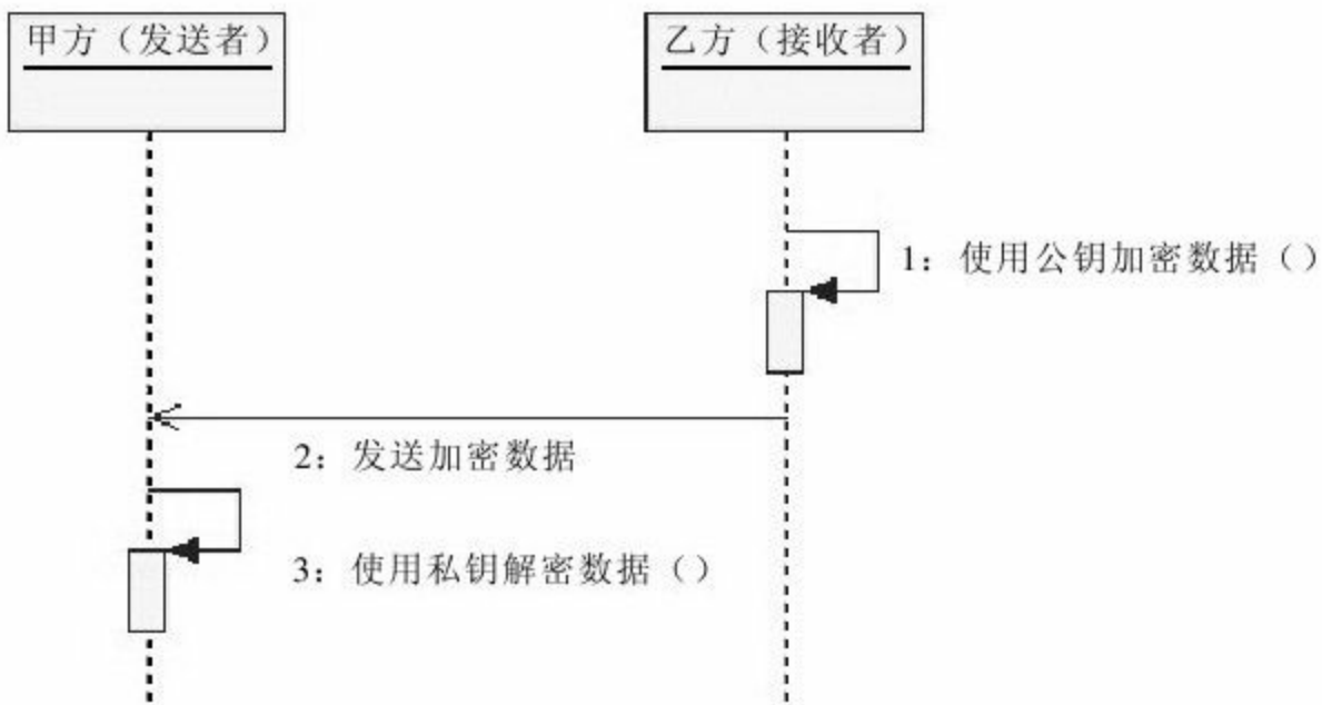
图 8-7 乙方向甲方发送RSA算法加密数据
