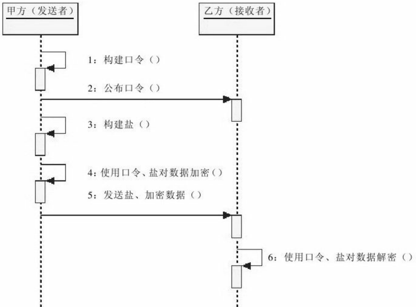
图 7-4 基于PBE算法的消息通信模型
