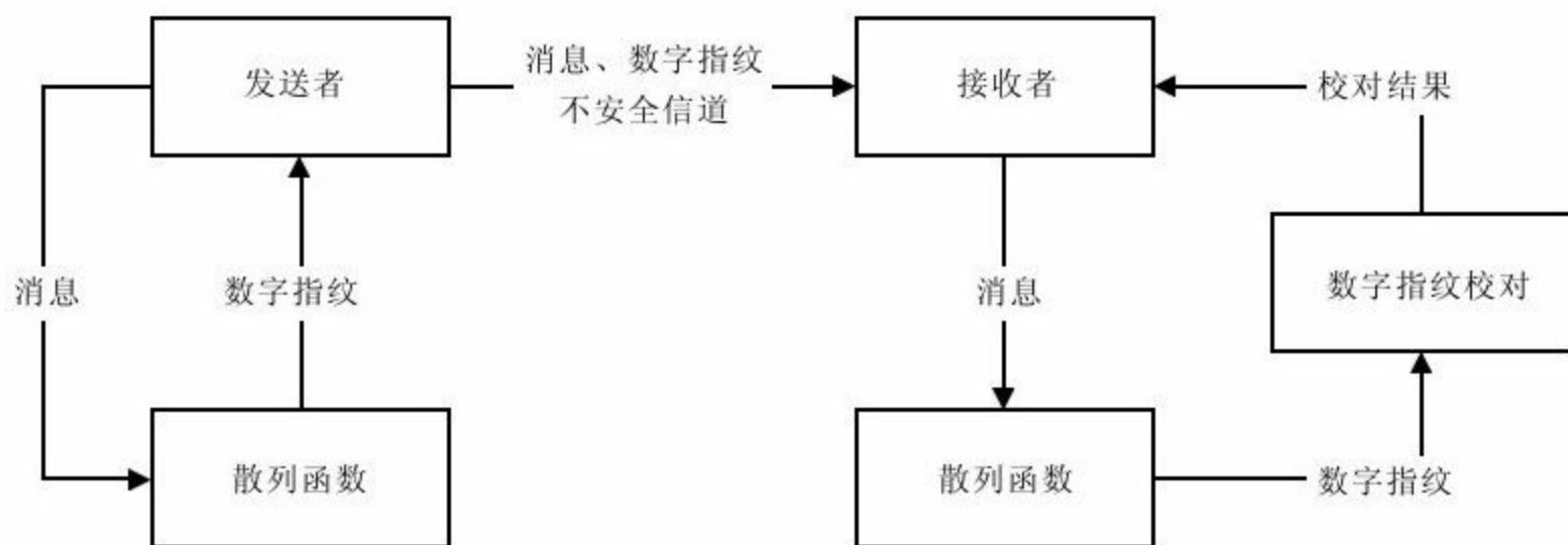
图 2-12 消息认证流程
