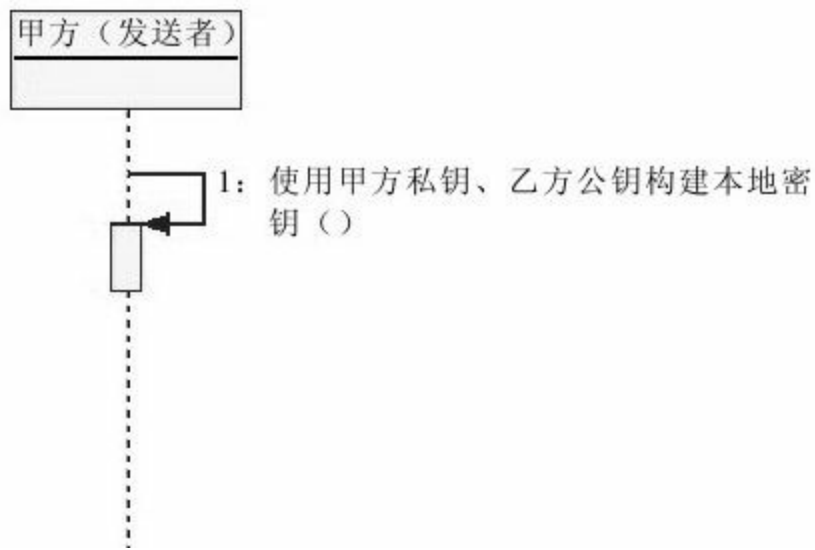
图 8-2 甲方构建DH算法本地密钥
