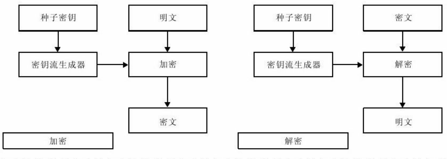
图 2-3 流密码加密与解密流程
