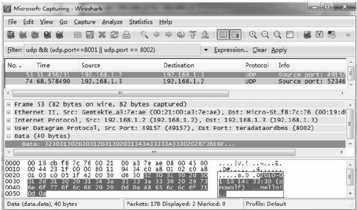
图 12-11 UDP交互消息拦截1
