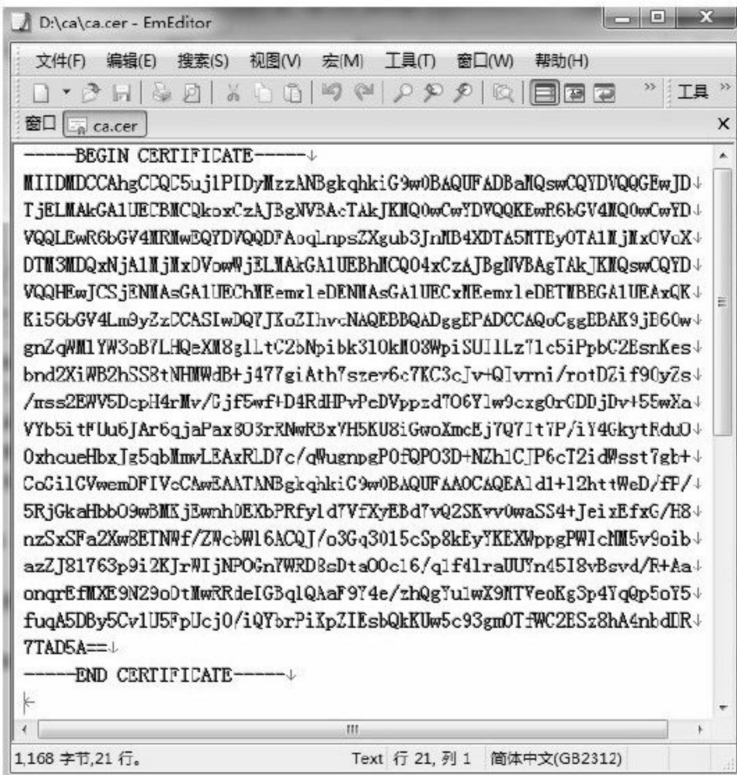
图 10-3 数字证书的Base64编码格式
