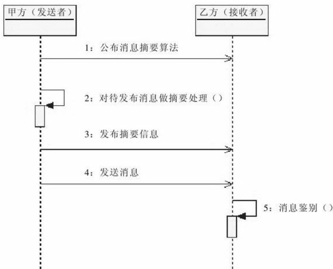
图 6-5 基于MD/SHA算法的消息传递
