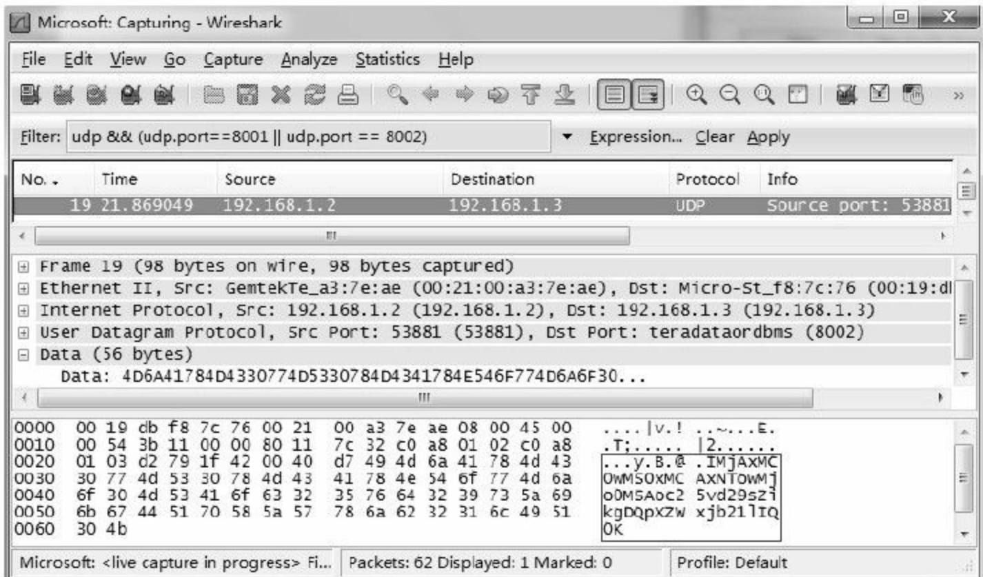
图 12-13 UDP交互消息拦截2
