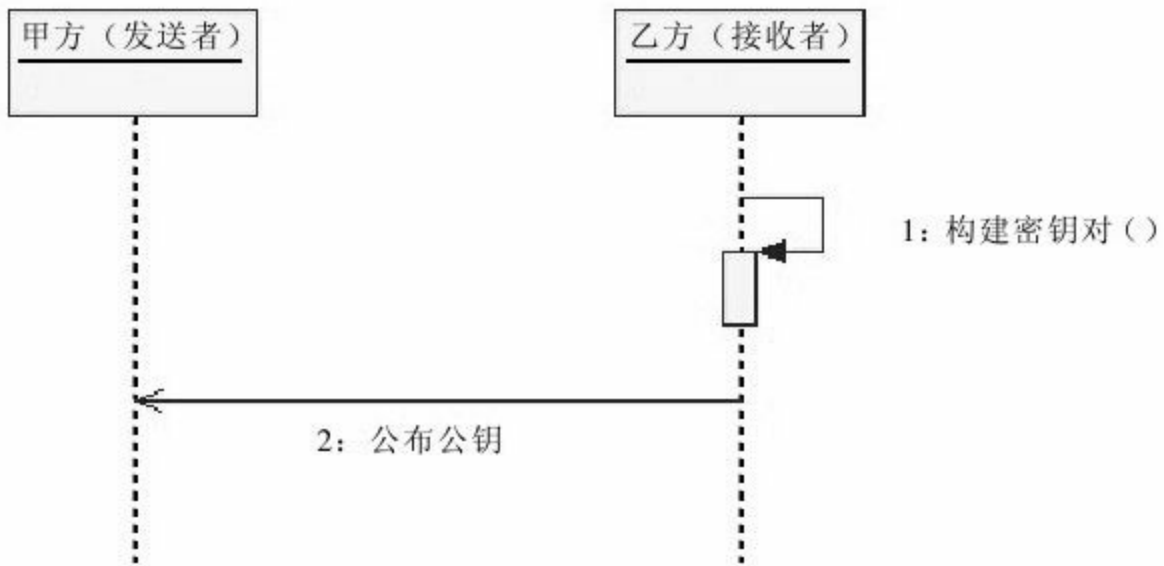
图 8-8 构建ElGamal密钥对
