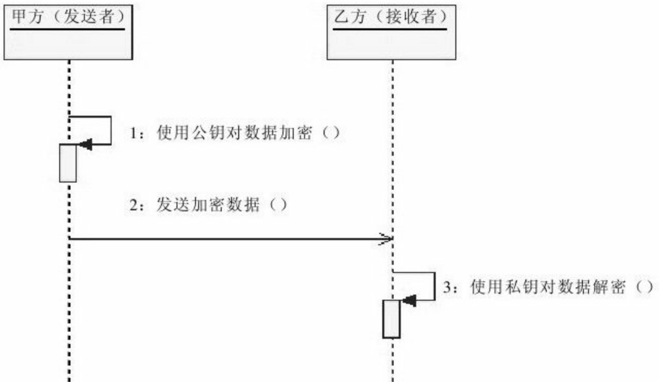
图 8-9 甲方向乙方发送ElGamal加密数据
