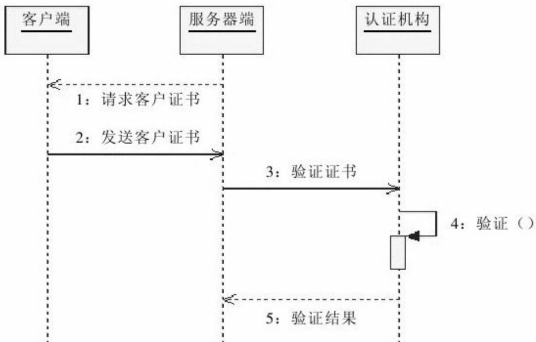
图 11-8 服务器端验证客户证书
