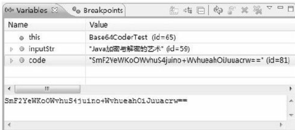
图 5-2 Base64 Debug 1
