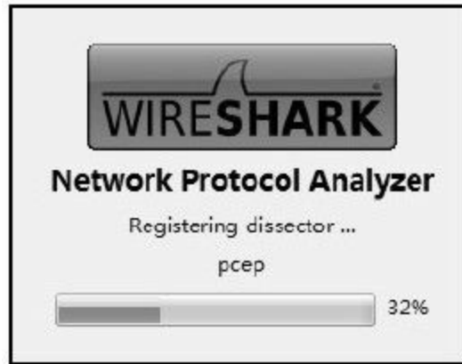
图 3-2 WireShark
