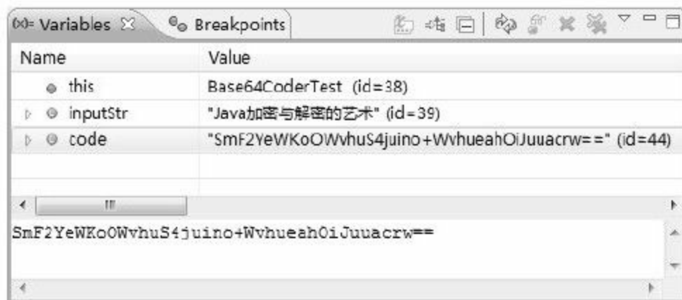
图 5-3 Base64 Debug 2
