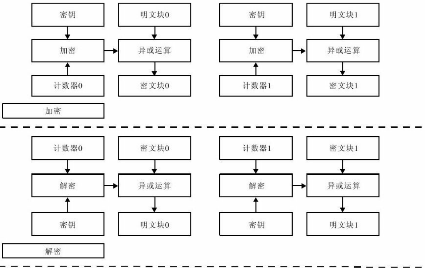
图 2-8 计数器模式
