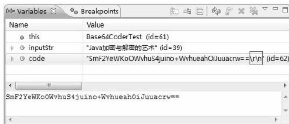
图 5-4 Base64 Debug 3
