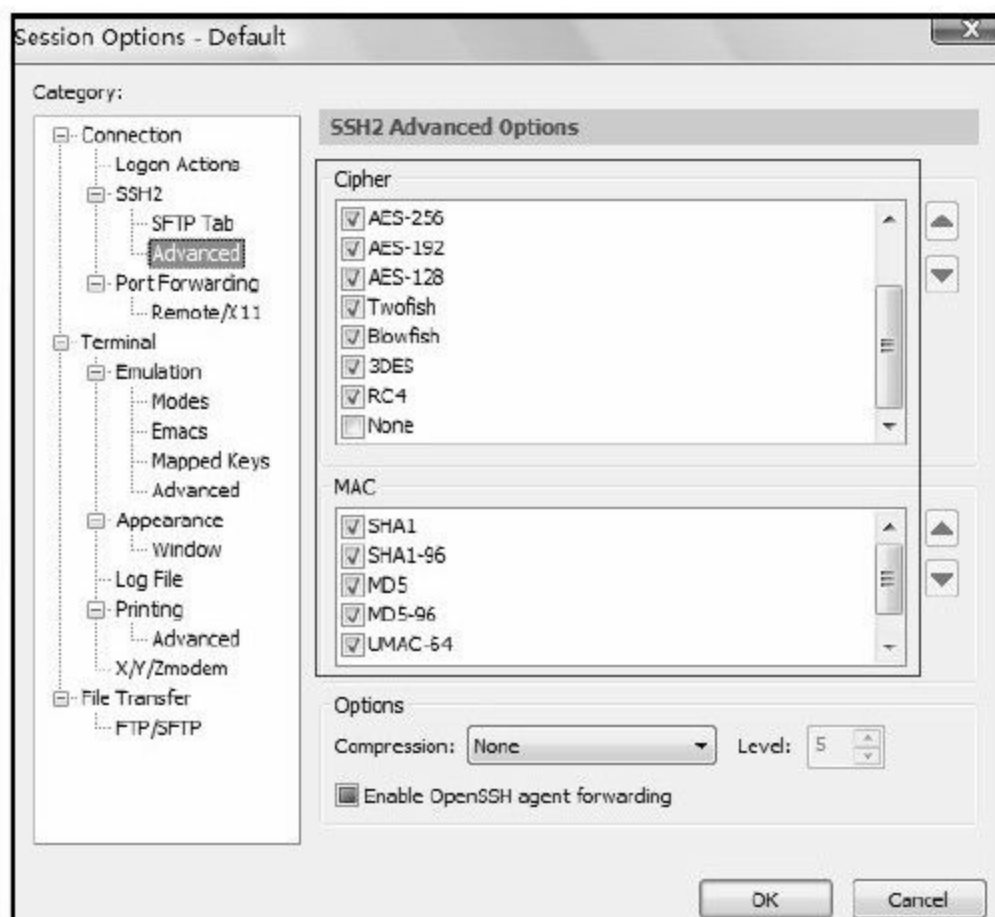
图 6-6 SecureCRT配置界面中的加密算法
