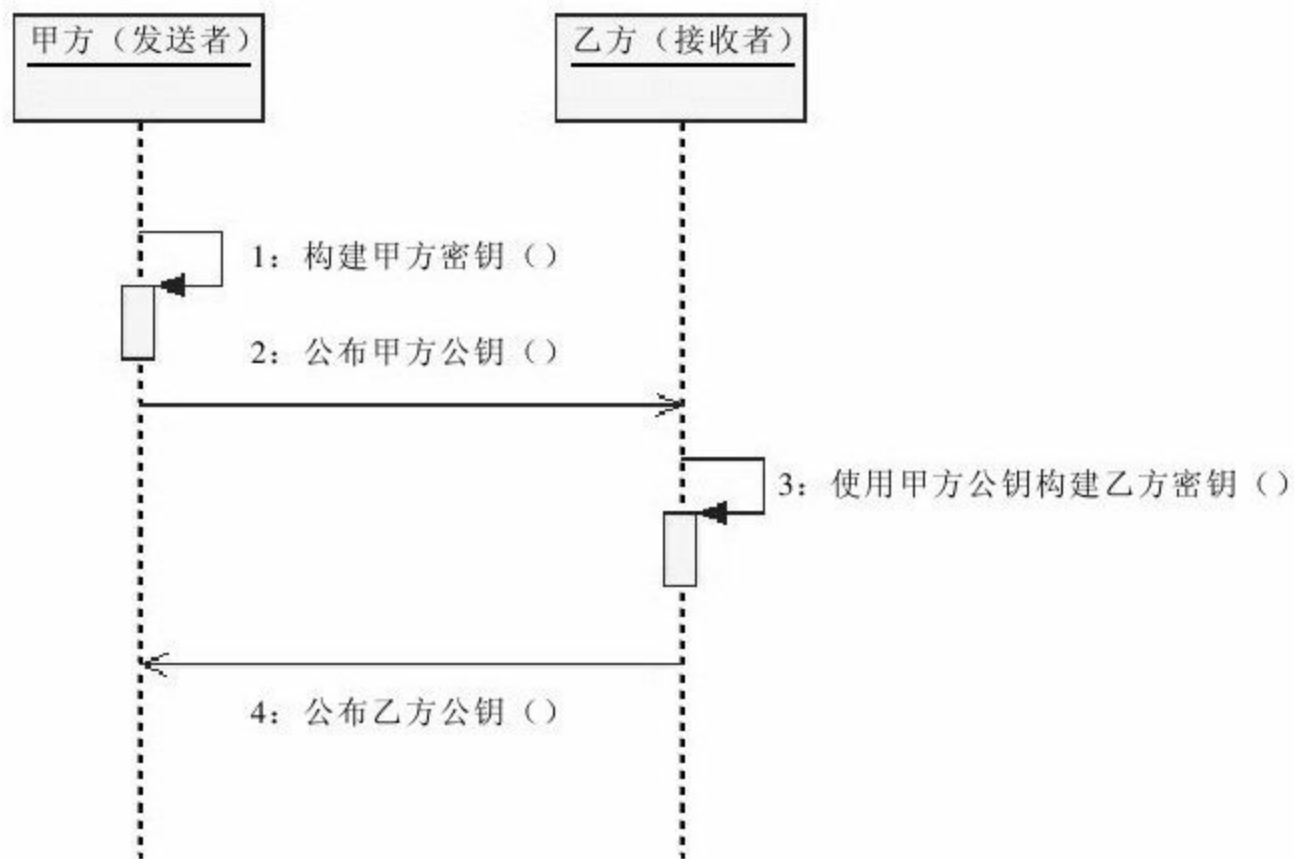
图 8-1 初始化DH算法密钥对
