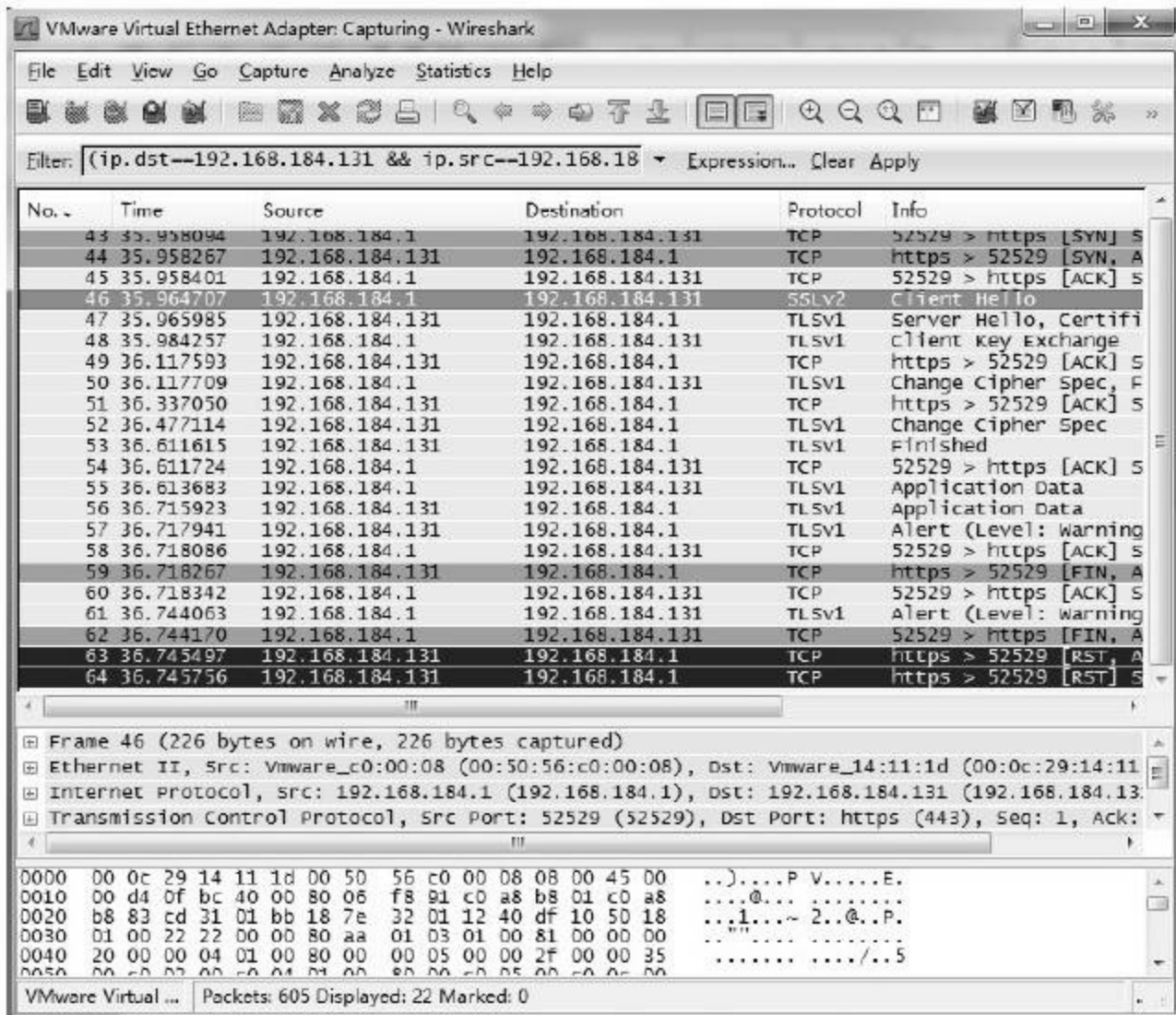
图 12-35 Wireshark监测结果2
