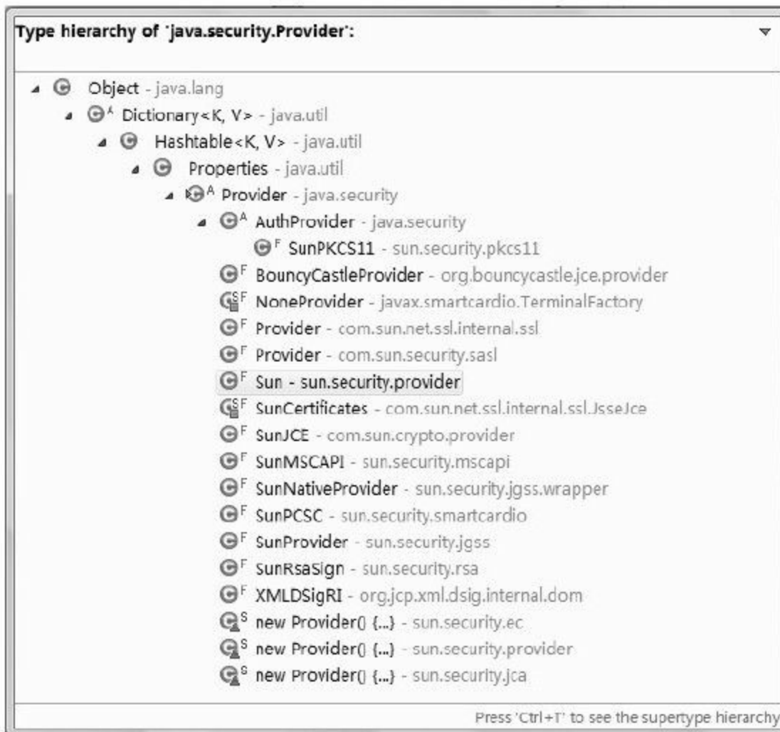
图 3-3 Provier类及其子类
