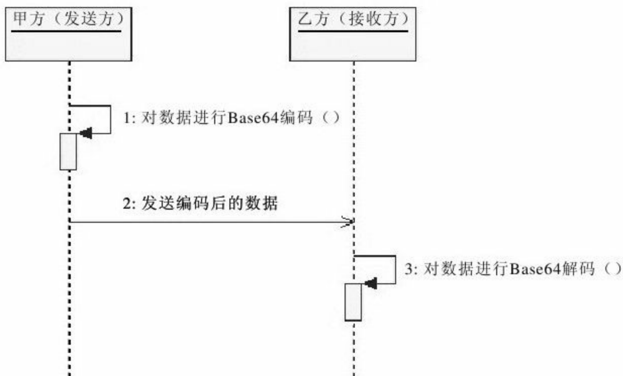
图 5-1 基于Base64算法的消息传递模型
