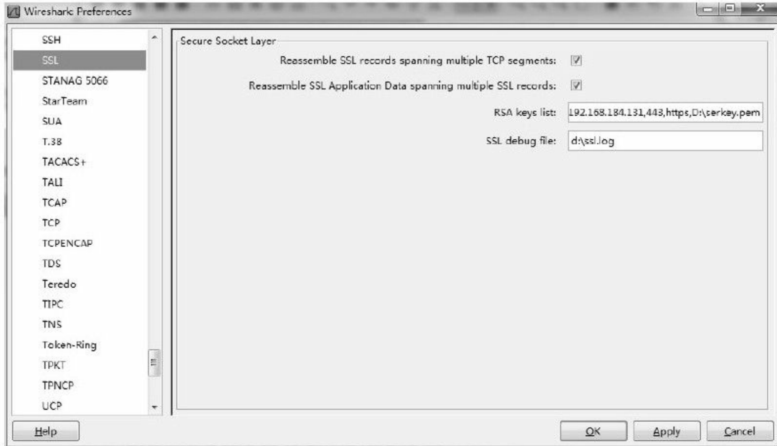
图 12-34 配置SSL协议
