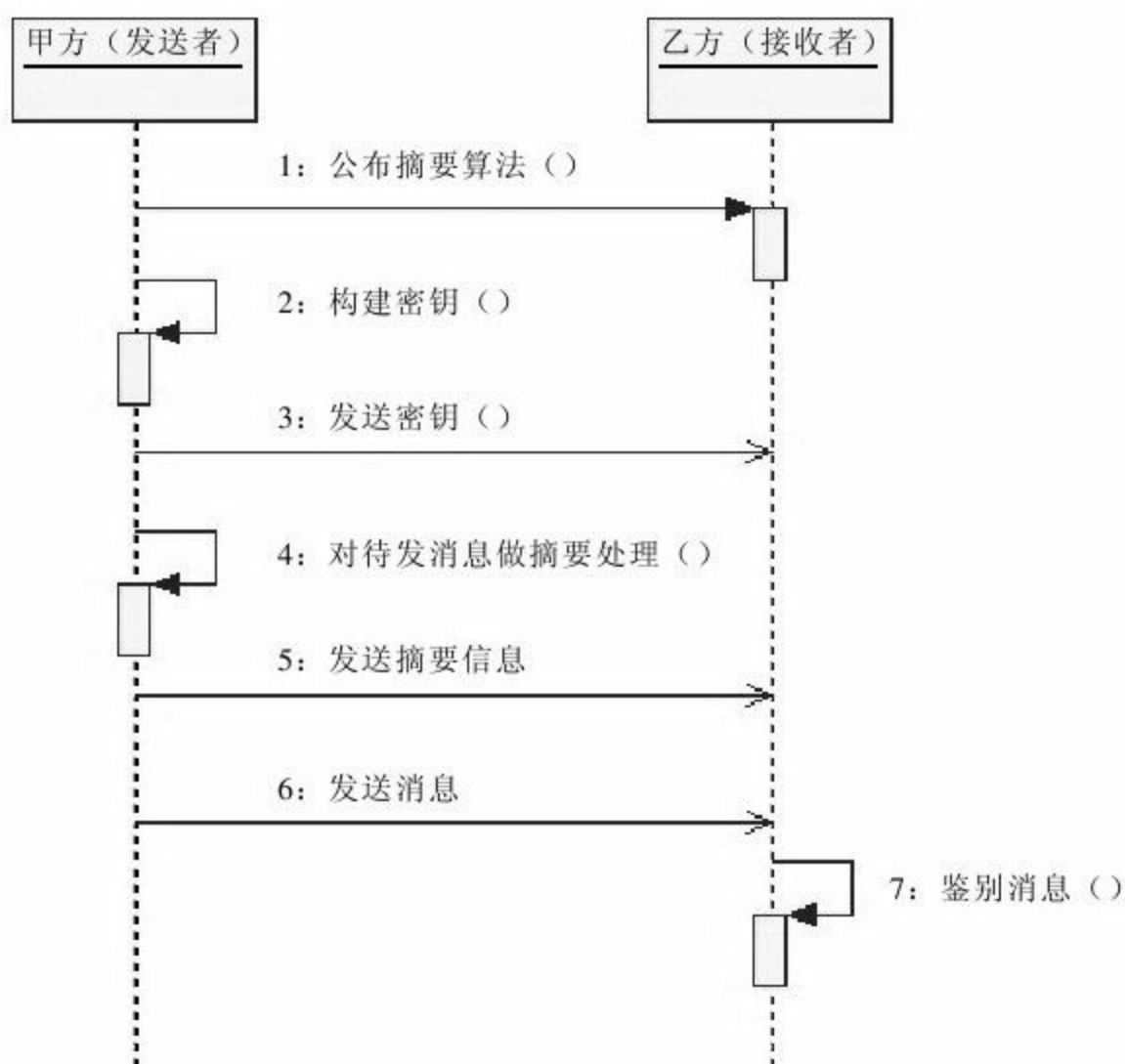
图 6-7 基于MAC算法的消息传递模型
