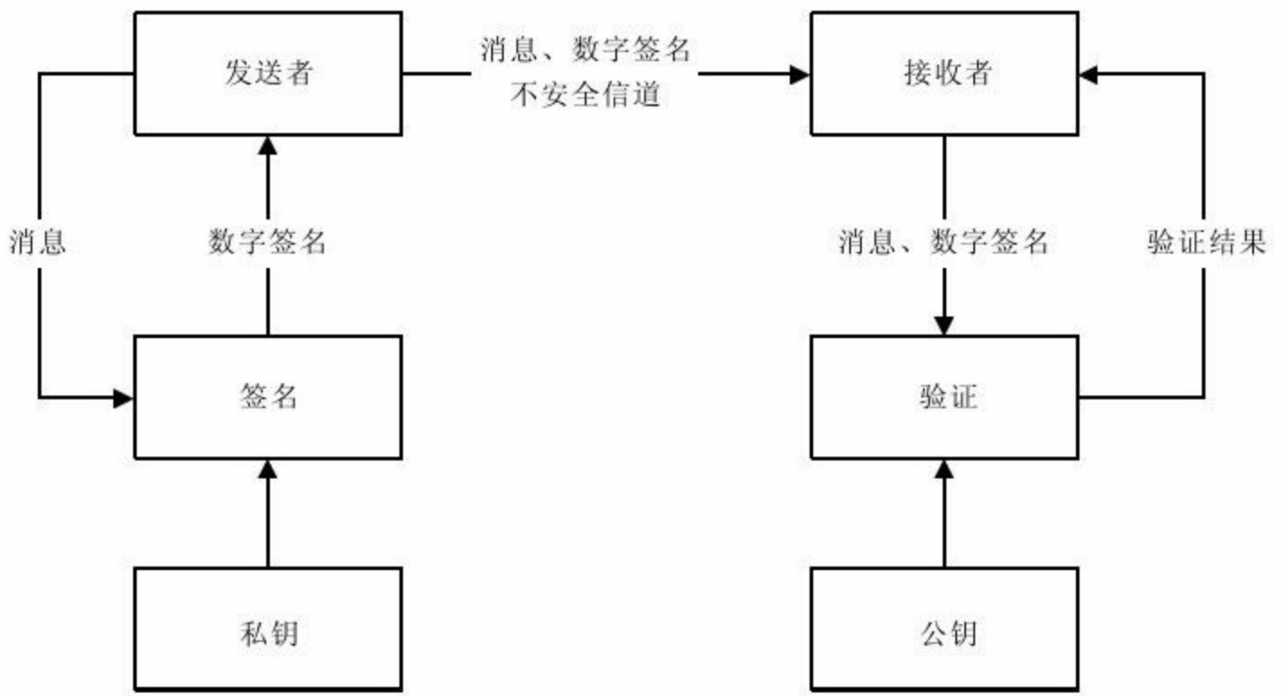
图 2-13 数字签名认证流程
