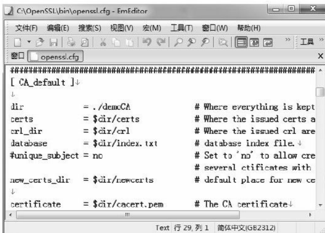
图 10-15 OpenSSL初始配置
