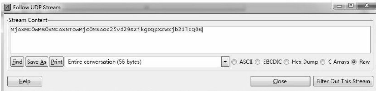
图 12-14 UDP交互内容Base64编码
