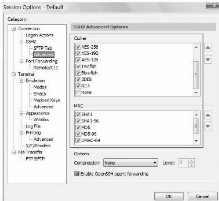
图 7-3 SecureCRT配置界面中的加密算法
