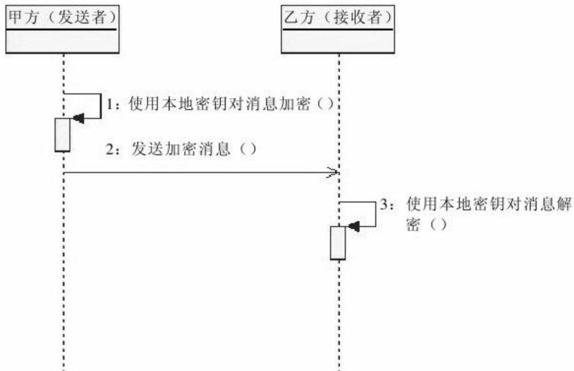
图 8-4 DH算法加密消息传递
