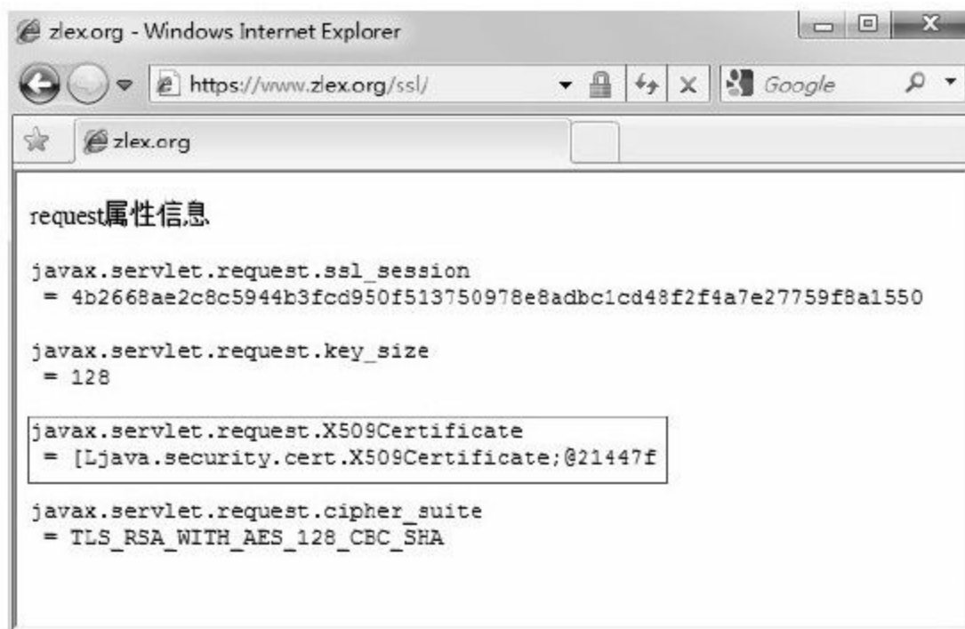
图 11-29 SSL/TLS协议中的request属性2
