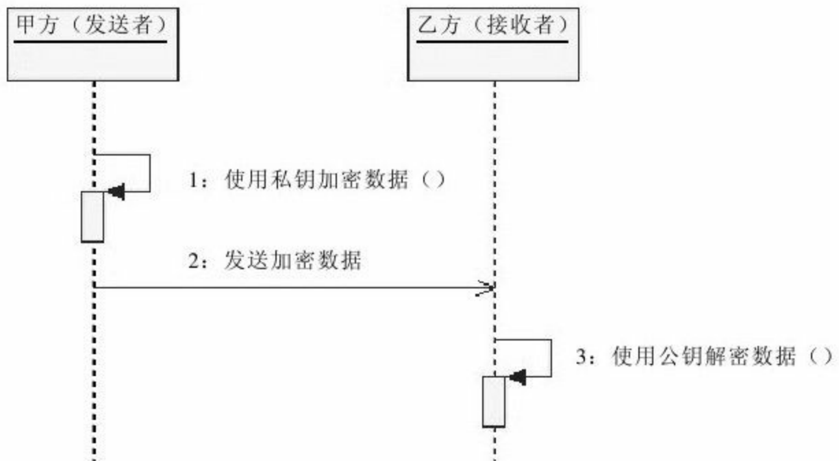
图 8-6 甲方向乙方发送RSA算法加密数据
