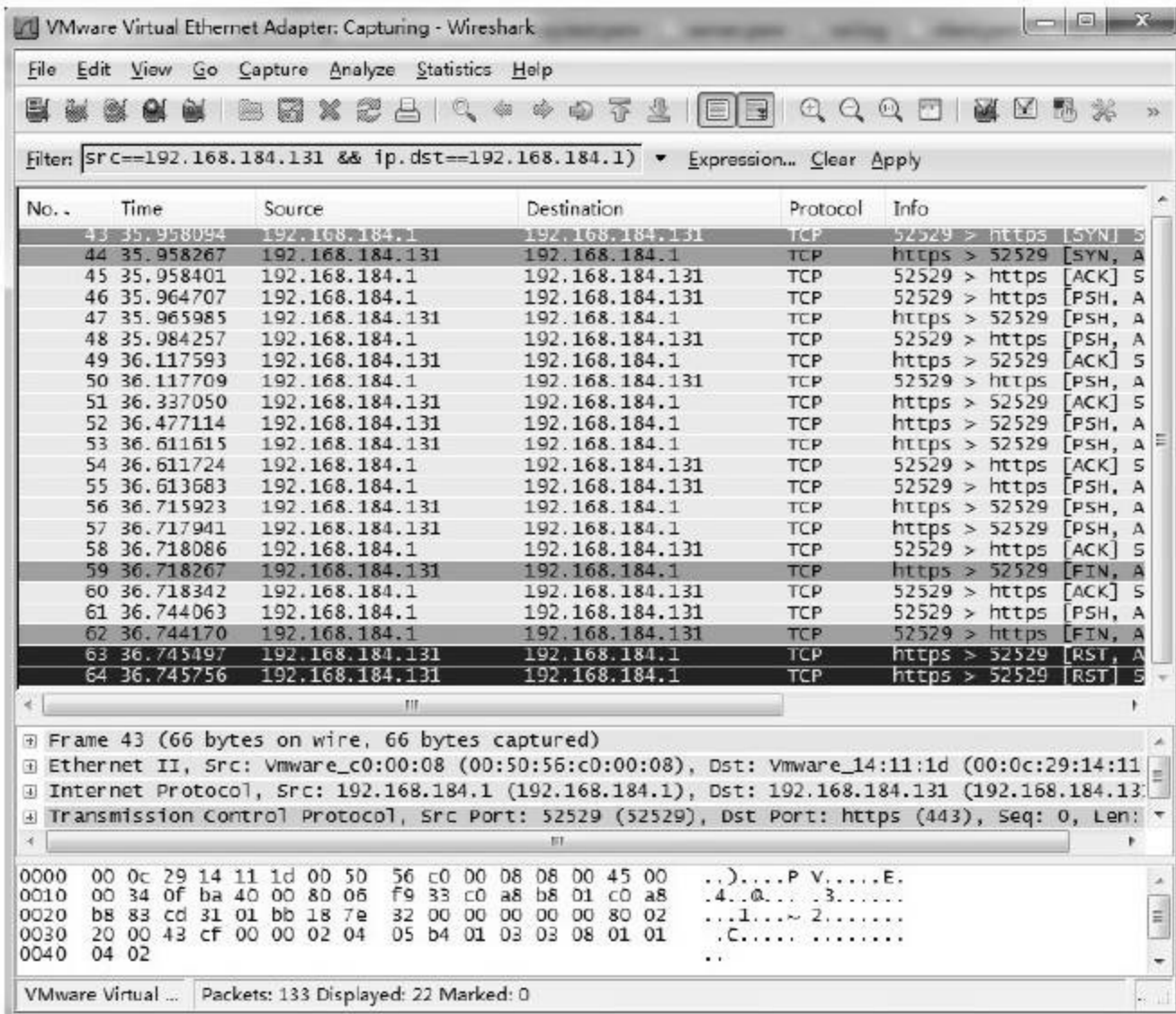
图 12-30 Wireshark监测结果1
