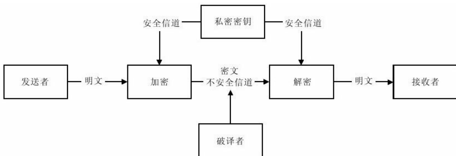
图 2-2 对称密码体制的保密通信模型
