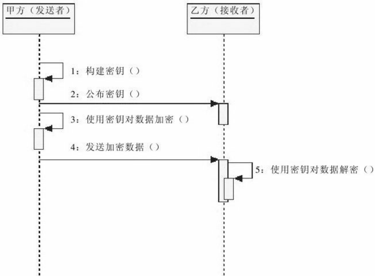
图 7-2 基于DES算法的消息传递模型
