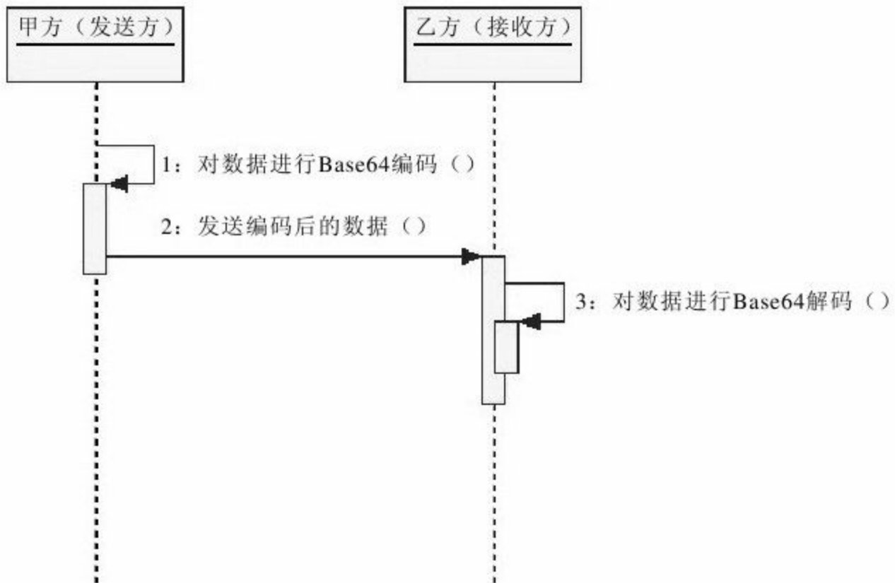
图 7-1 基于Base64算法的消息交互模型
