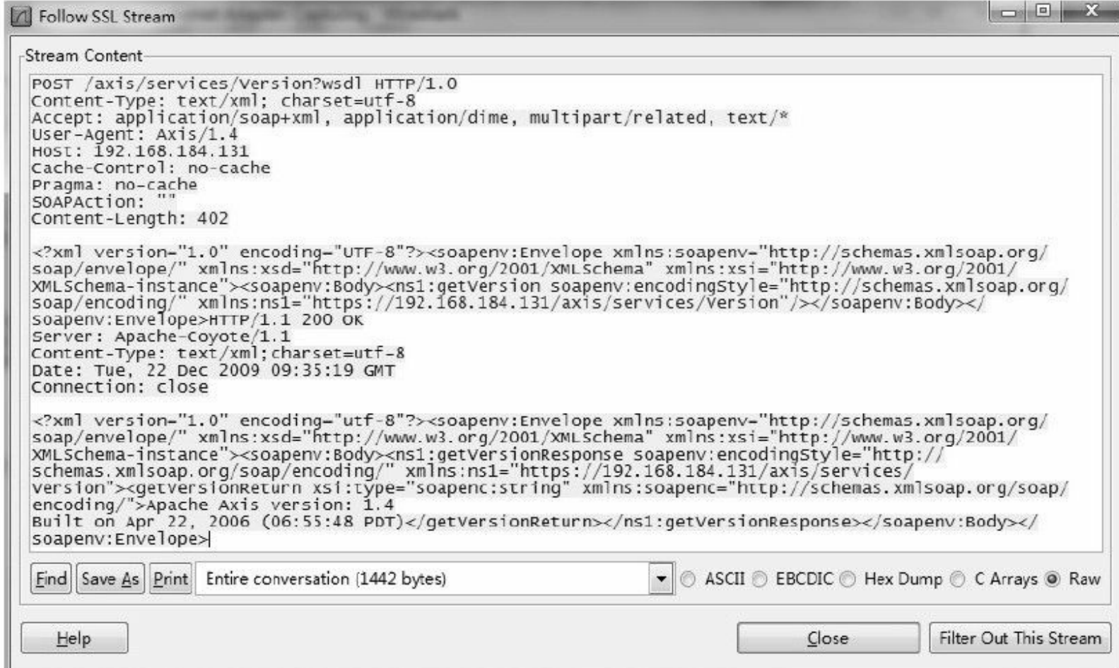
图 12-42 SOAP交互内容
