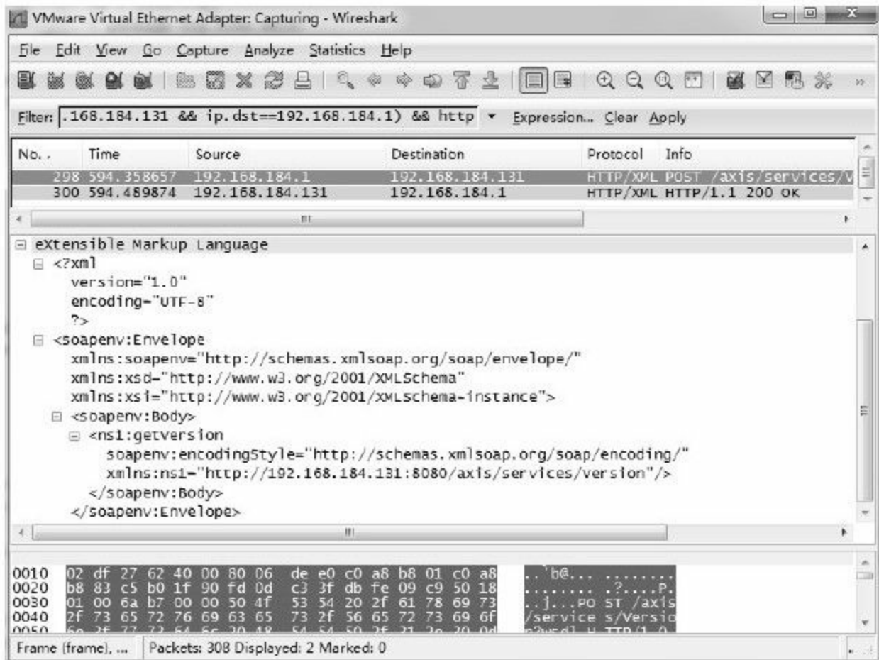
图 12-22 SOAP请求和回应信息
