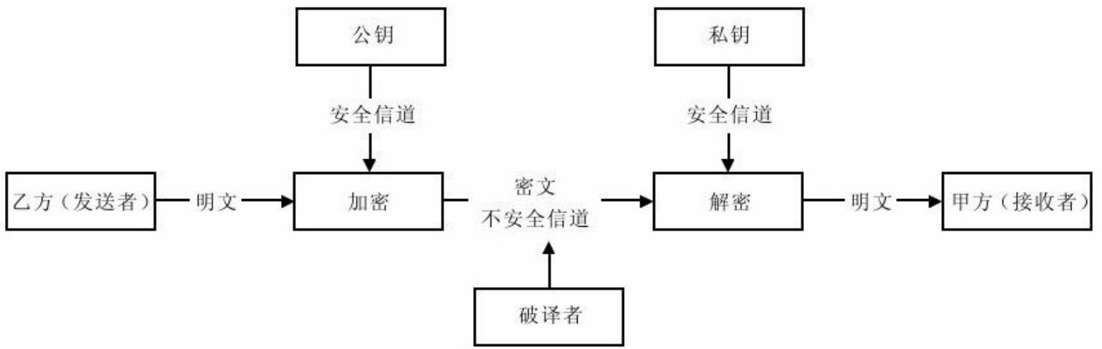
图 2-11 公钥加密-私钥解密的保密通信模型
