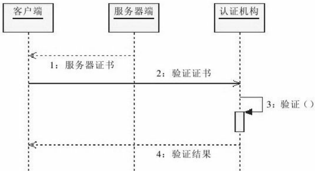
图 11-7 客户端验证服务器证书
