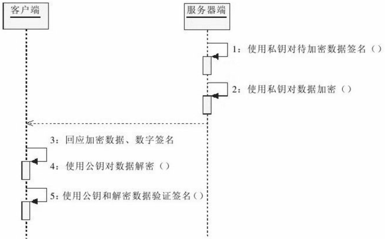
图 10-6 服务器端响应客户端
