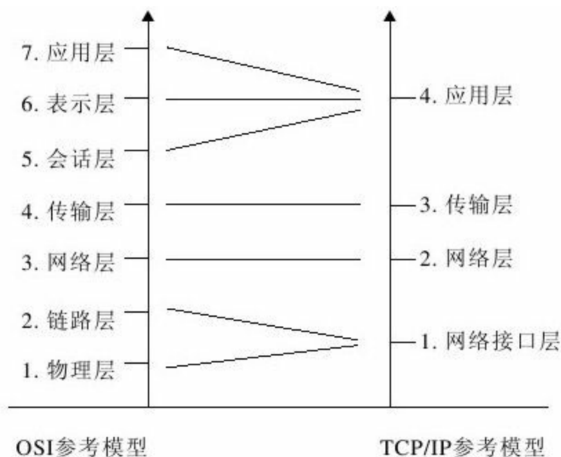
图 1-3 OSI参考模型和TCP/IP参考模型对比
