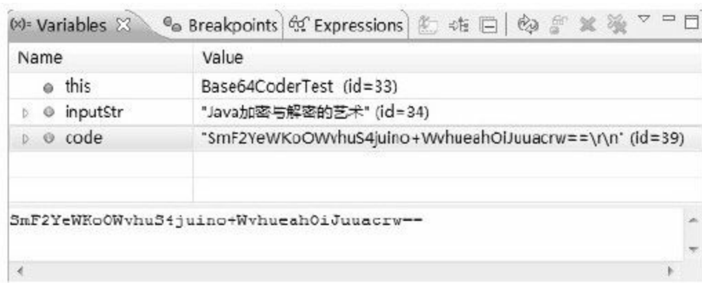
图 5-5 Base64 Debug 4
