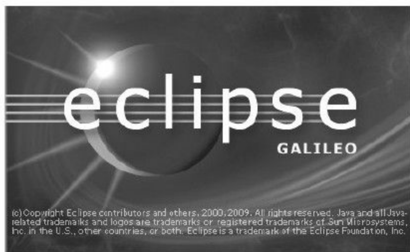
图 3-1 Eclipse Galileo
