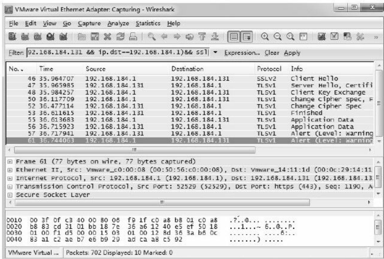
图 12-36 Wireshark监测结果3
