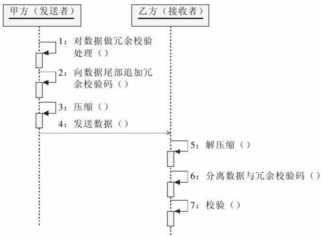
图 6-9 压缩/解压缩数据传递模型
