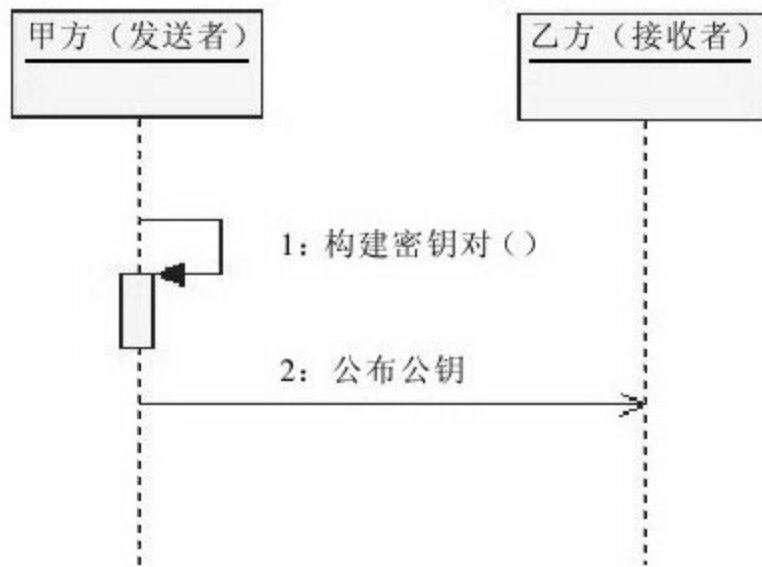
图 8-5 构建RSA算法密钥对
