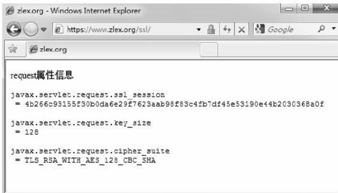
图11-21 SSL/TLS协议中的request属性1
