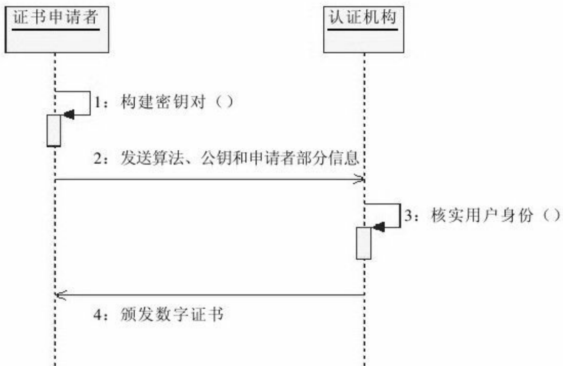
图 10-4 数字证书颁发流程
