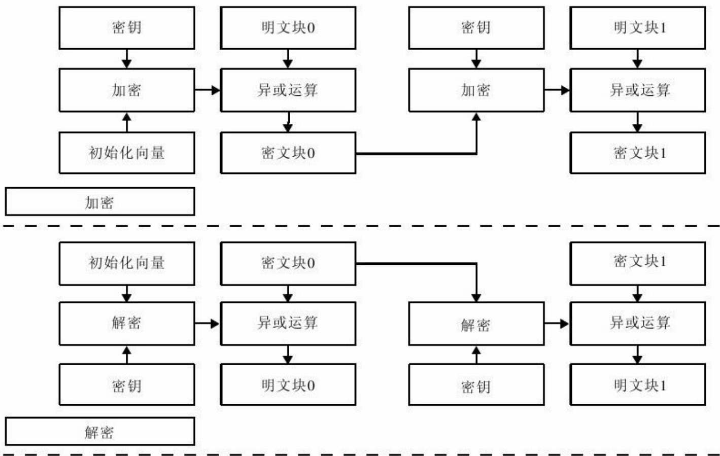
图 2-6 密文反馈模式
