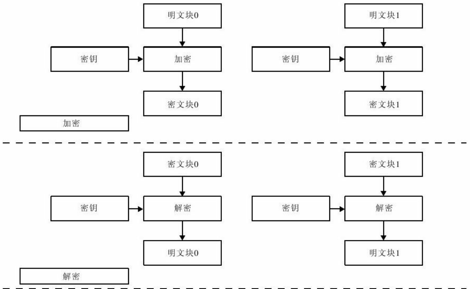
图 2-4 电子密码本模式
