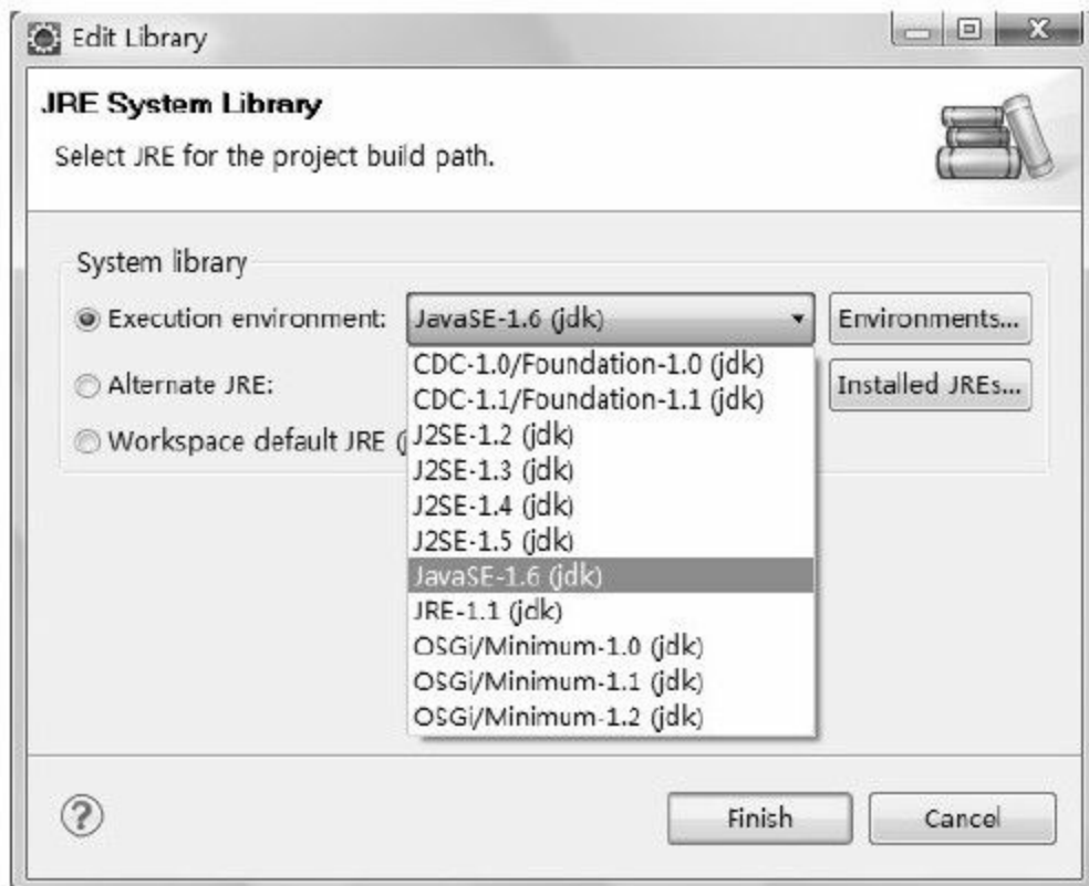
图 5-6 在Eclipse中设置项目的JRE
