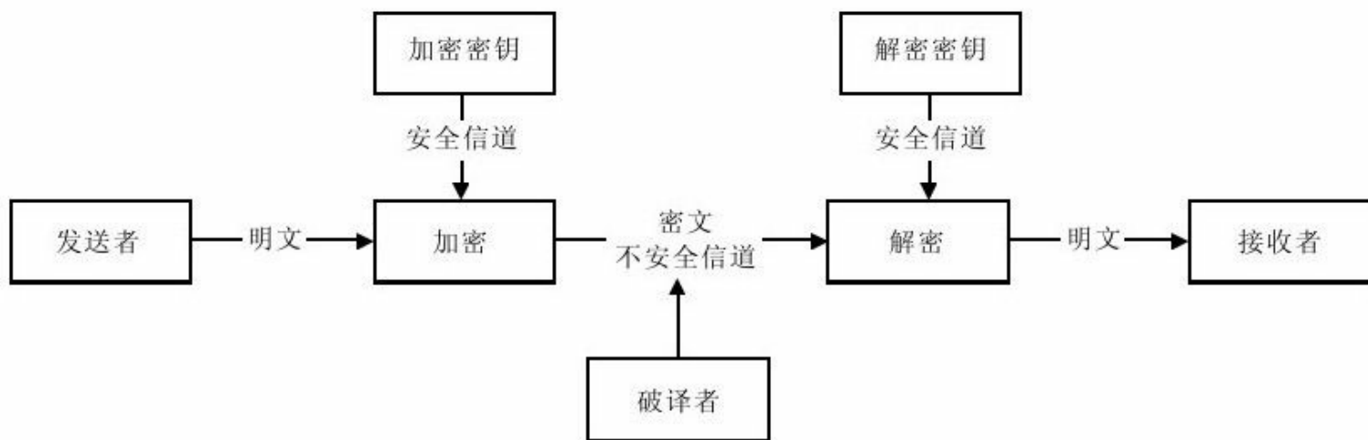
图 2-1 保密通信模型
