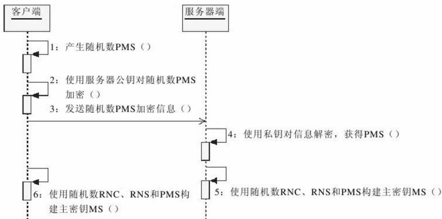
图 11-9 构建主密钥MS
