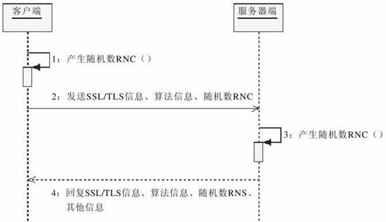
图 11-6 对等协商加密算法
