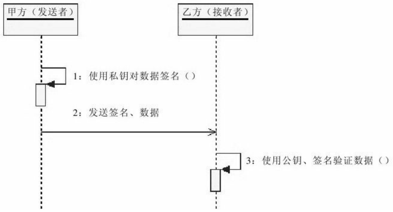
图 9-2 甲方向乙方发送数据
