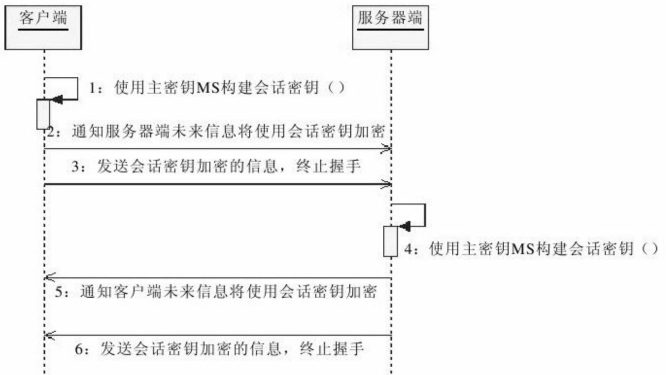
图 11-10 构建会话密钥
