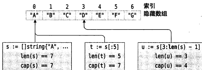
图 4-3 切片与其底层数组的概念图
