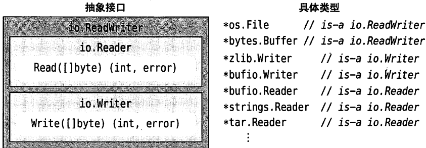
图 6-1 用于读写字节切片的接口和类型
