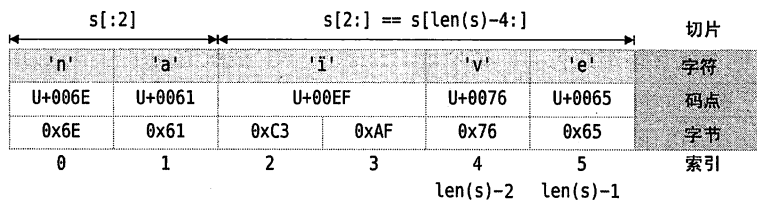
图 3-1 字符串剖析
