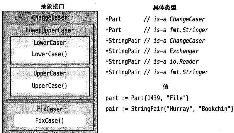
图 6-2 Caser 接口、类型和示例值
