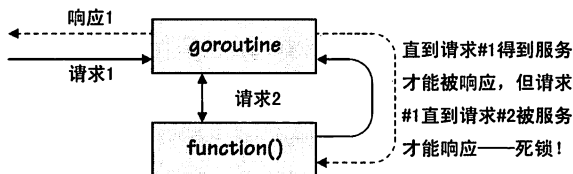
图 7-2 死锁：一个试图用对自身的请求来服务于请求的 goroutine
