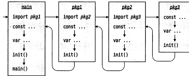
图 5-1 程序的启动顺序
