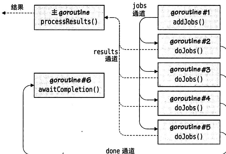
图 7-5 多个独立的并发作业
