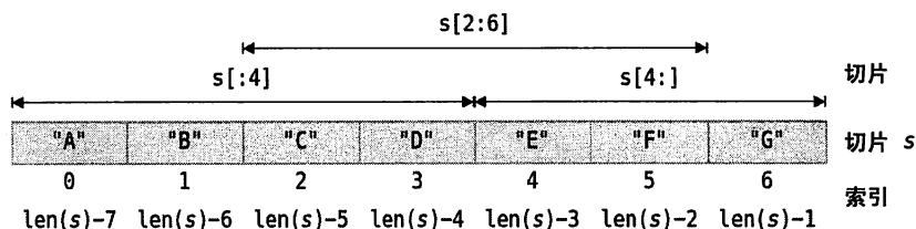
图 4-4 切片剖析
