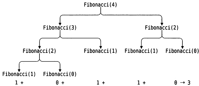
图 5-2 递归的 Fibonacci
