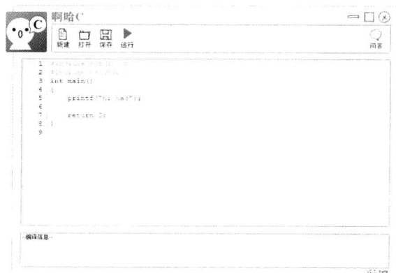
图 2-10 删除 system("pause")
