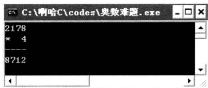
图 5-1 运行结果
