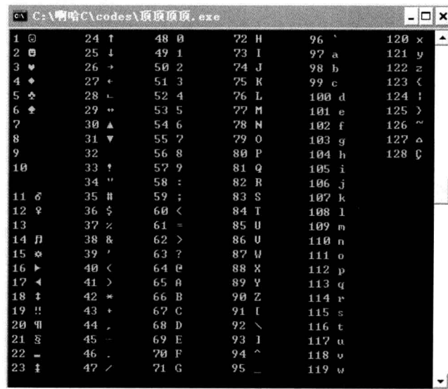
图 7-4 ASCII 字符
