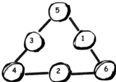
图 5-2 三角形三边之和相等
