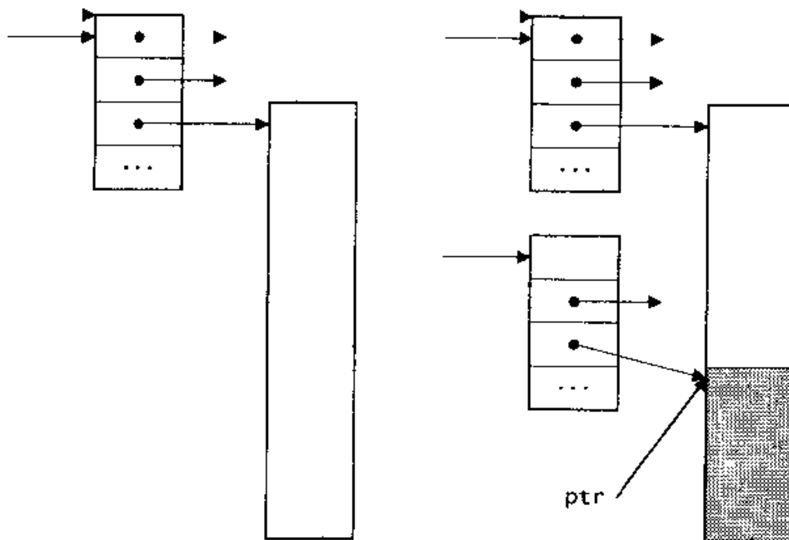
图5-2 分配一空闲块的末端
