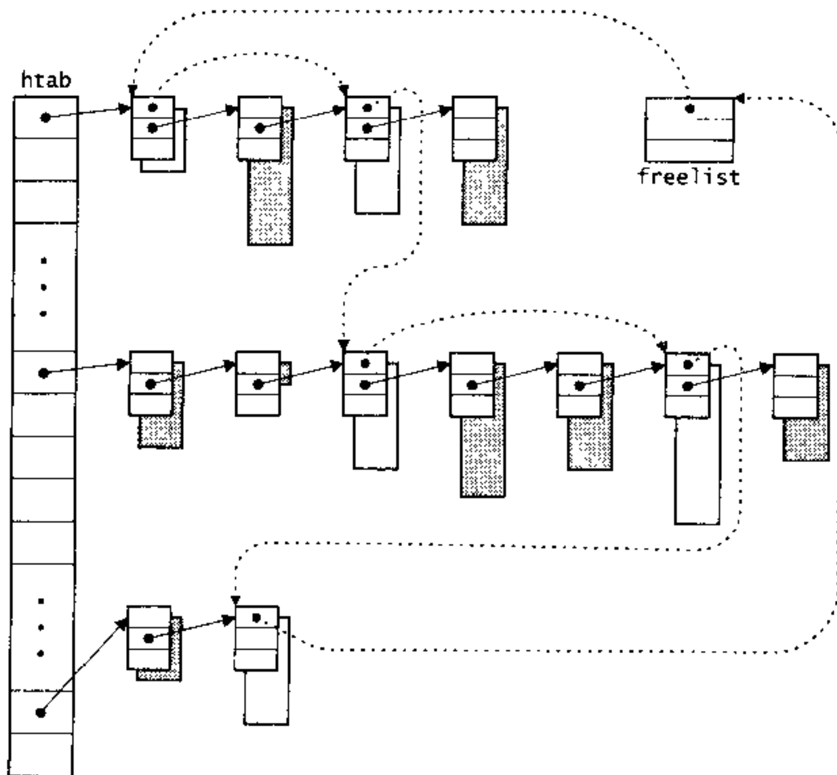
图5-1 htab和freelist的结构
