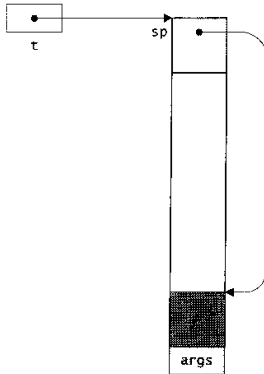
图20-5 Thread_T结构与堆栈的分配
