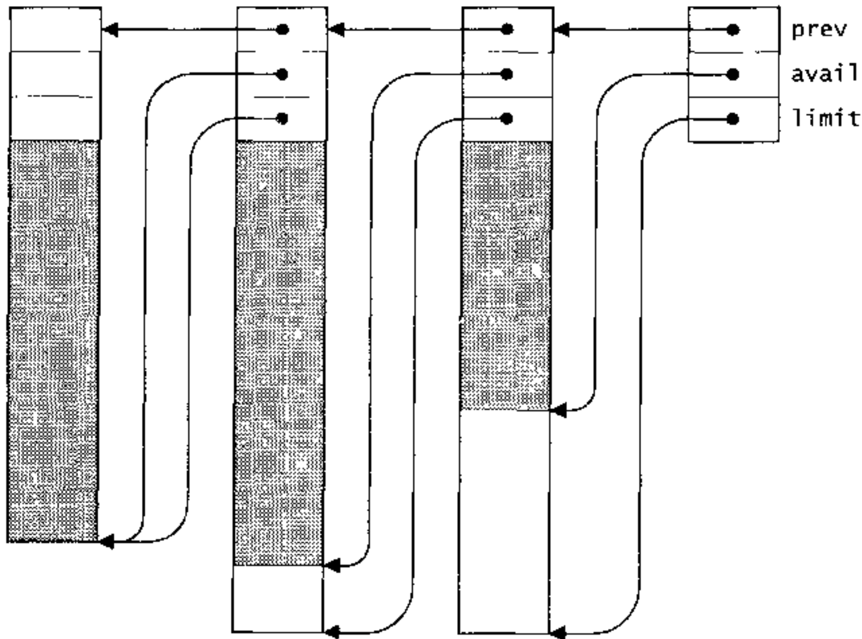
图6-1 有三个存储块的实存块
