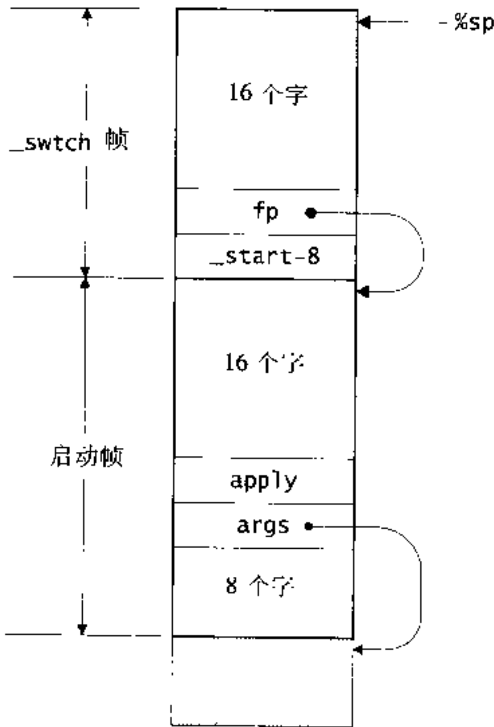
图20-7 SPARC上的启动和初始_swatc帧
