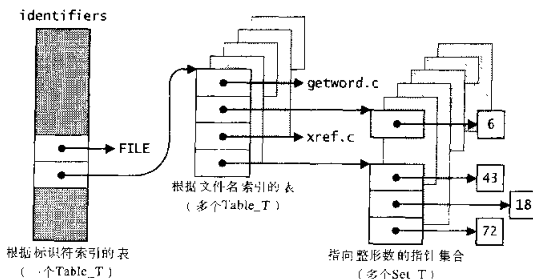
图9-1 交叉引用列表的数据结构
