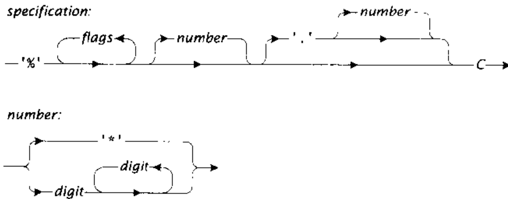
图14-1 转换说明符语法
