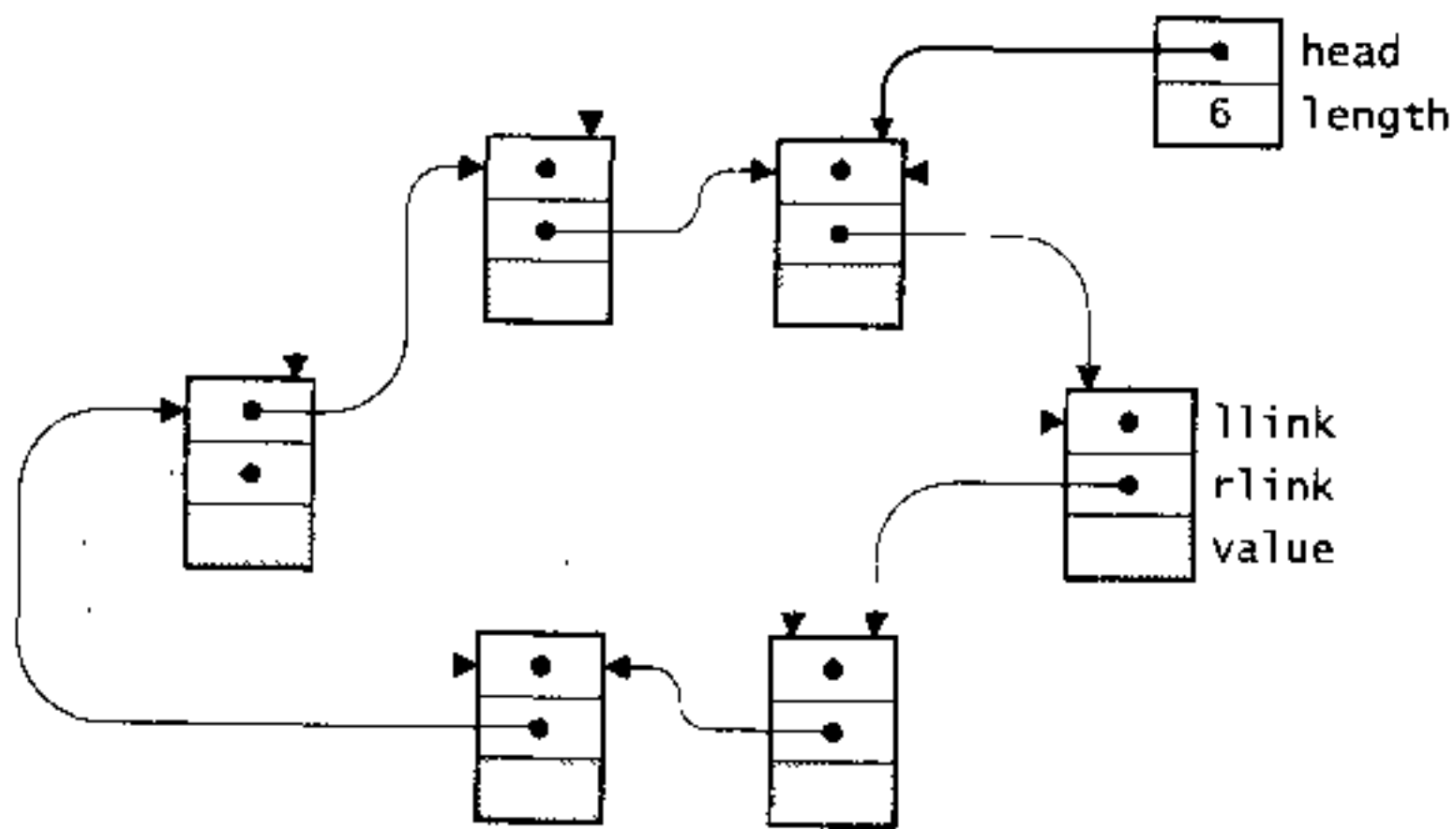
图12-1 一个六元素的环
