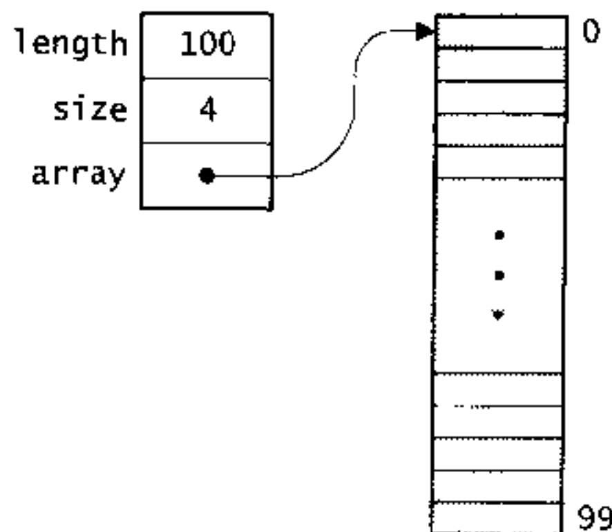
图10-1 由Array_new(100, sizeof int)创建的Array_T
