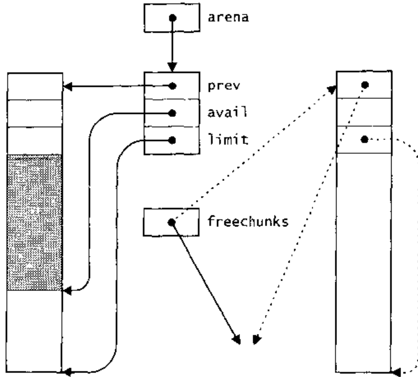
图6-2 当 nfree < THRESHOLD 时释放存储块
