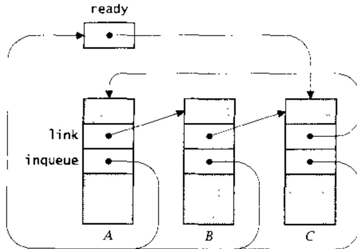
图20-3 就绪队列中的三个线程
