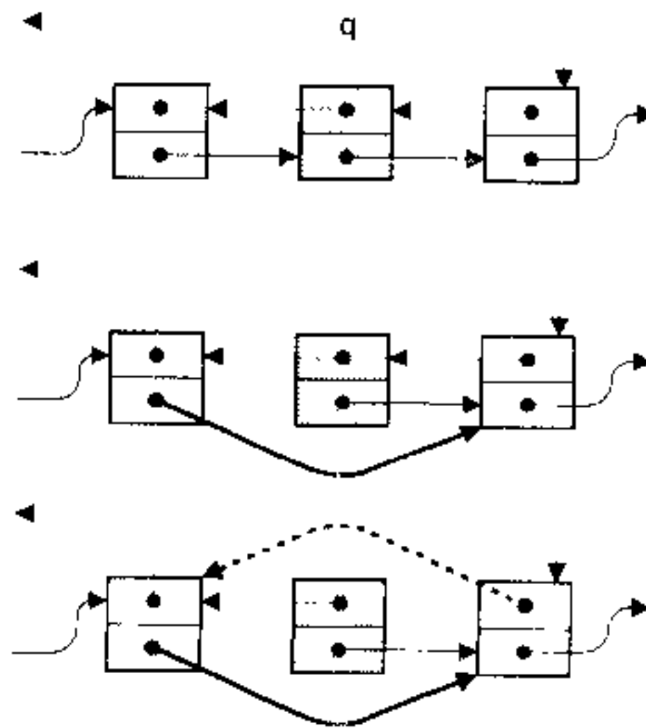
图12-4 删除节点 q
