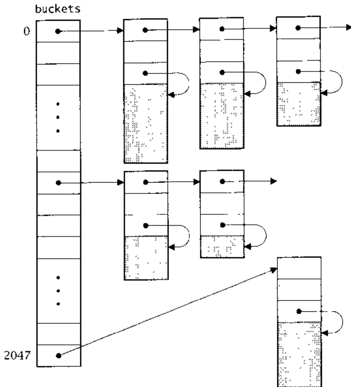
图3-2 Hash表结构
