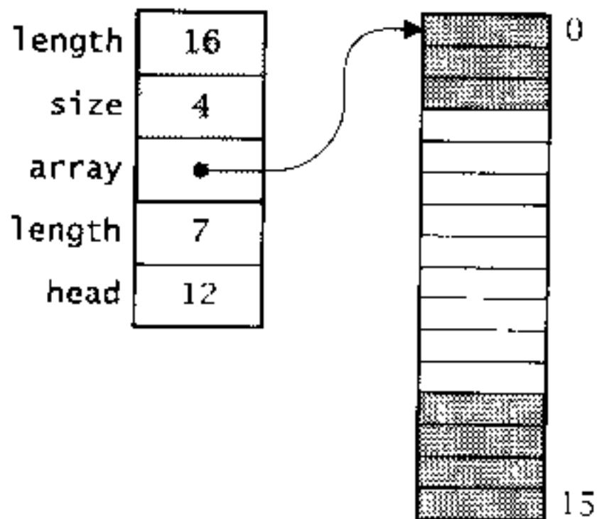
图11-1 16元素的序列
