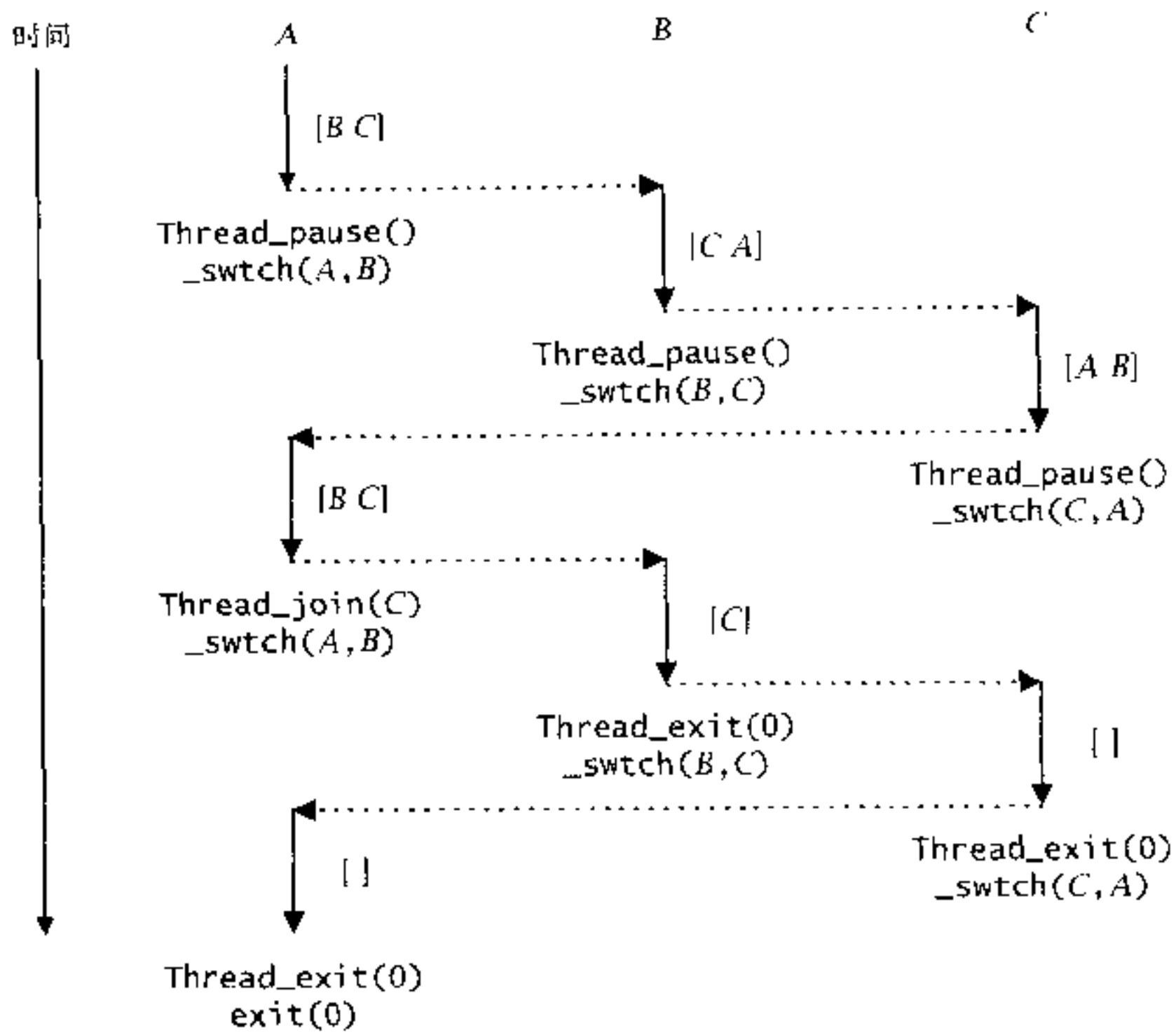
图20-4 三个线程之间的上下文切换
