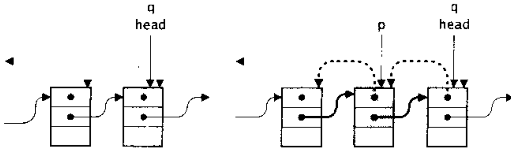
图12-2 将一个新值插入到head的左边
