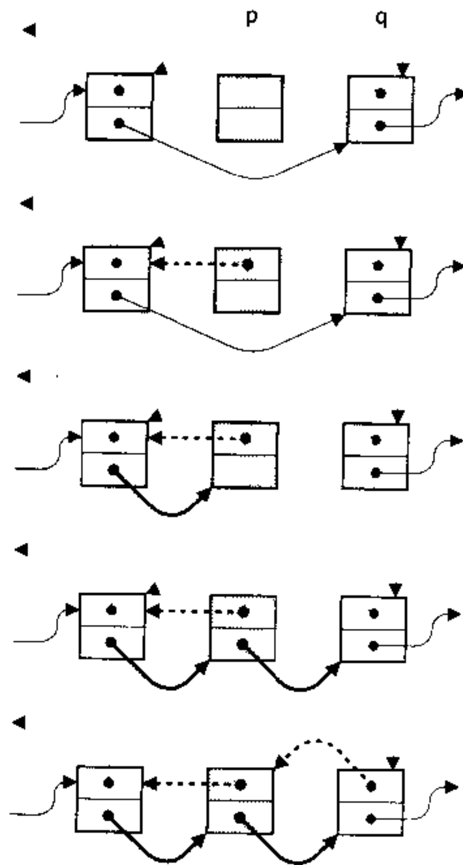
图12-3 将一个新的节点插入到q的左边
