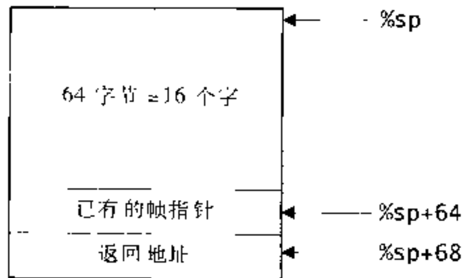
图20-6 _swtch 堆栈帧的布局
