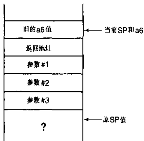
图 18.3 link 指令期间的堆栈帧
