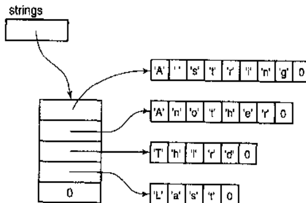
图 6.1 指向字符串的指针的数组
