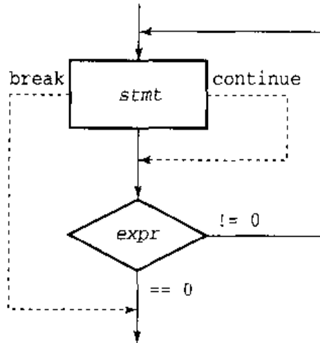
图 4.3 do 语句的执行过程
