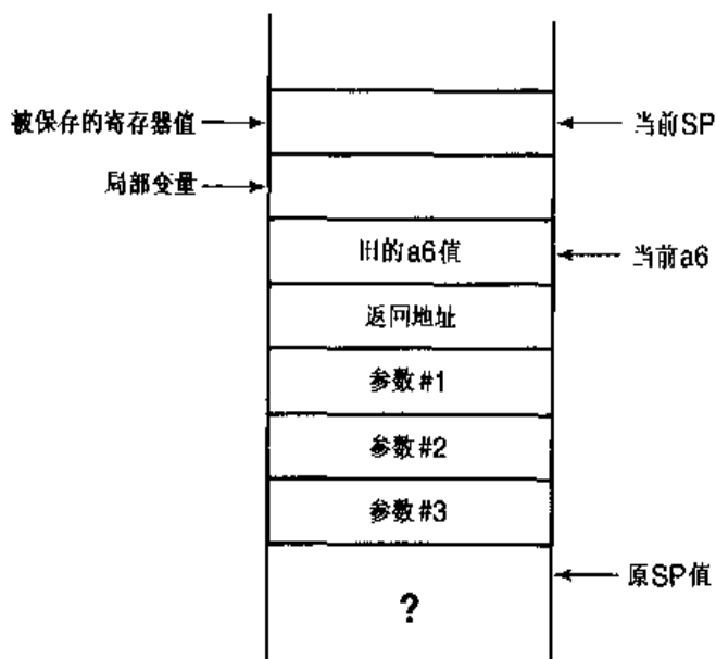
图 18.4 link 指令之后的堆栈帧
