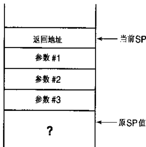
图 18.2 在跳转了程序指令之后的堆栈帧
