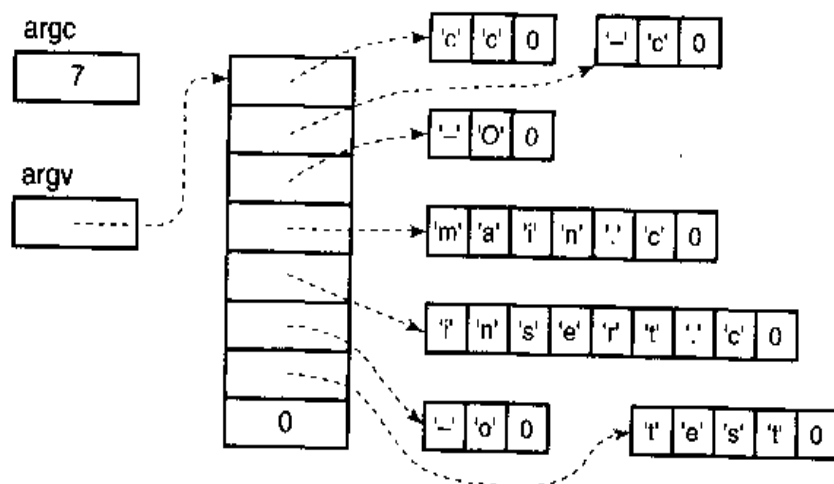
图 13.1 命令行参数
