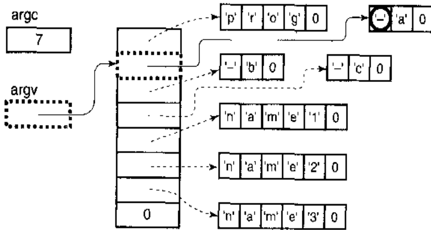
图 13.2 访问参数
