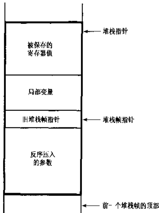
图 18.5 堆栈帧布局
