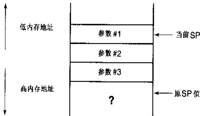
图 18.1 压入参数后的堆栈帧
