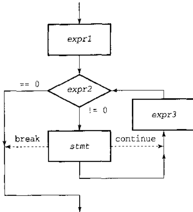
图 4.2 for 语句的执行过程
