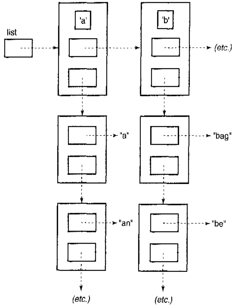
图 12.1 一个索引表
