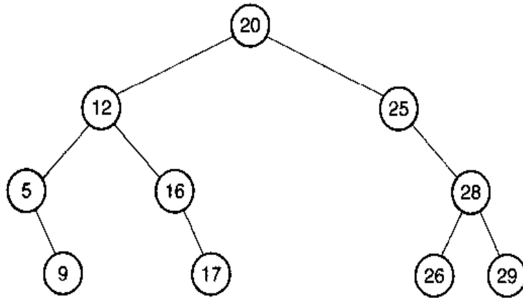
图 17.1 二叉搜索树
