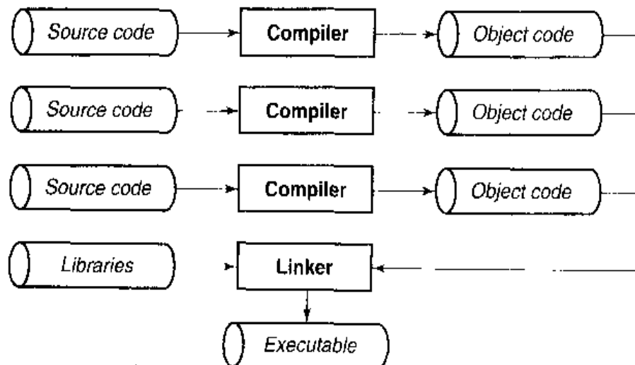
图 2.1 编译过程
