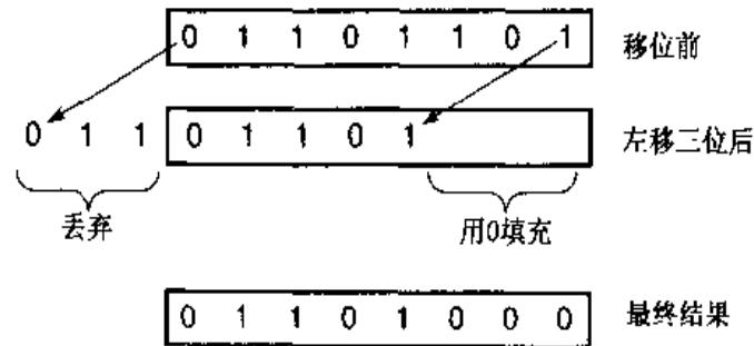
图 5.1 左移 3 位
