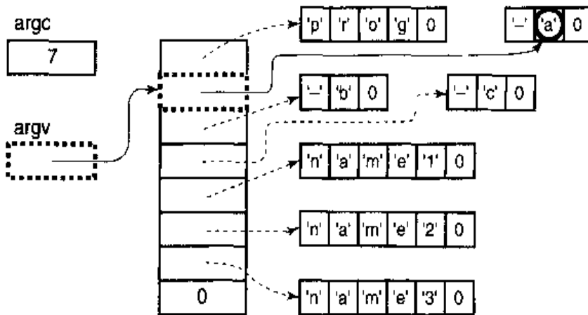
图 13.3 访问参数中的下一个字符
