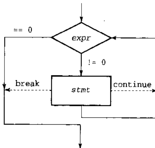
图 4.1 while 语句的执行过程
