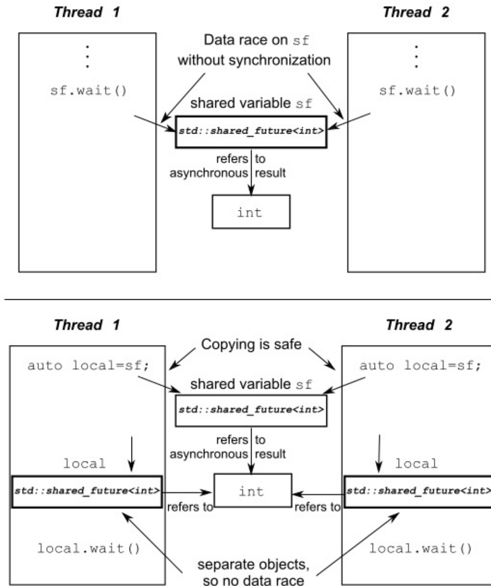
图4.1 使用多个 std::shared_future 对象来避免数据竞争
