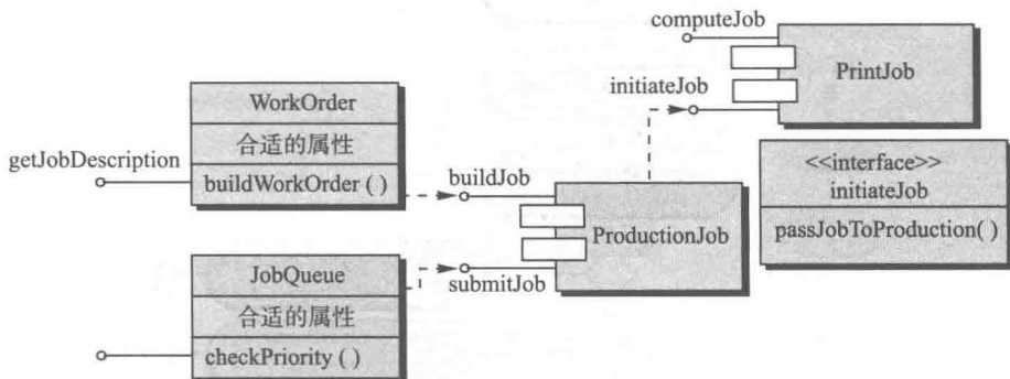
图 13-7 为 PrintJob 重构接口和类定义
