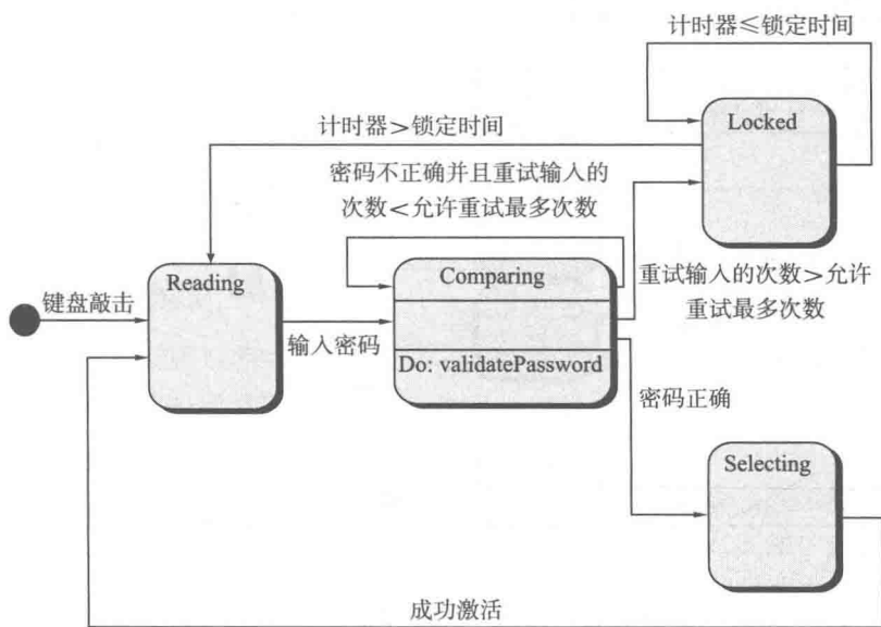
图 10-1 ControlPanel 类的状态图
