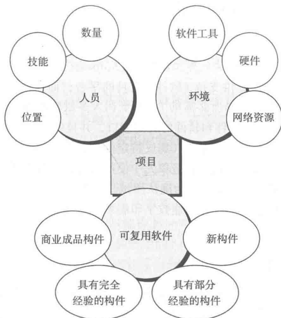
图 24-1 项目资源
