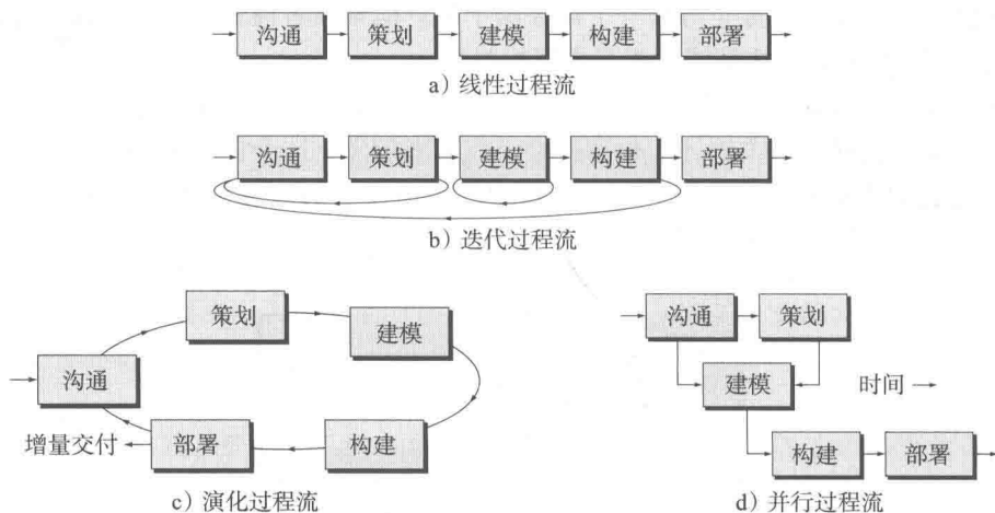
图 3-2 过程流
