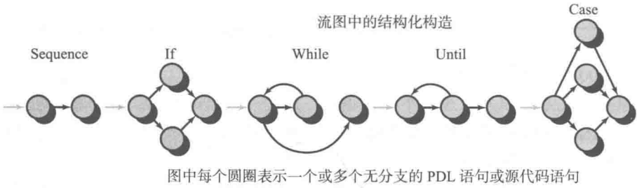
图 18-1 流图表示
