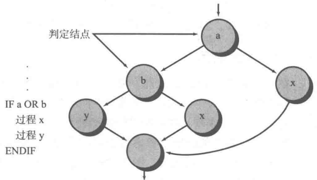
图 18-3 复合逻辑
