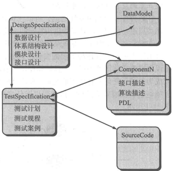
图 21-2 配置对象
