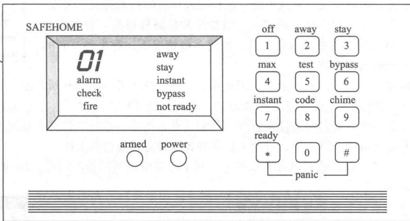
图 7-1 SafeHome 控制面板
