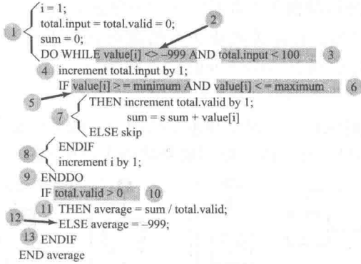
图 18-4 已标识结点的 PDL
