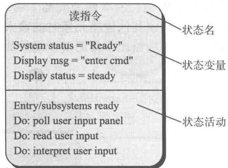
图 7-5 UML 状态图表示
