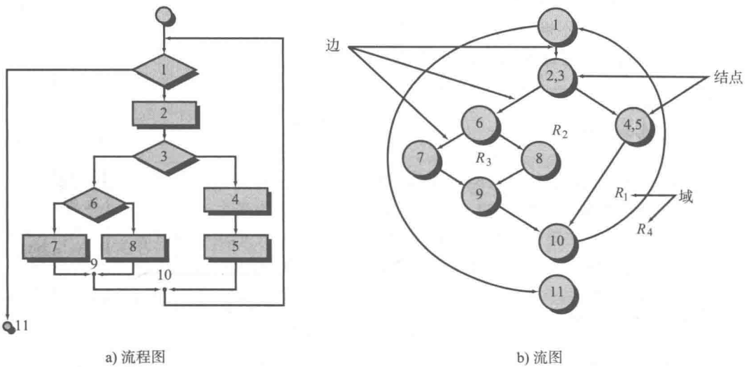
图 18-2 流程图和流图
