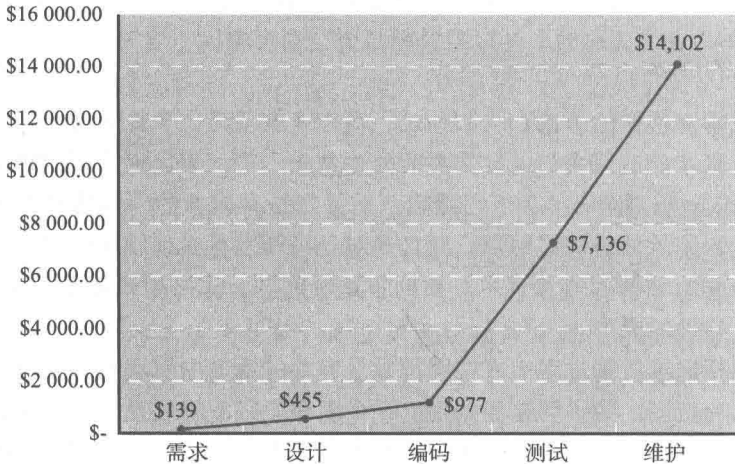
图 15-2 改正错误和缺陷的相对成本 [Boe01b]
