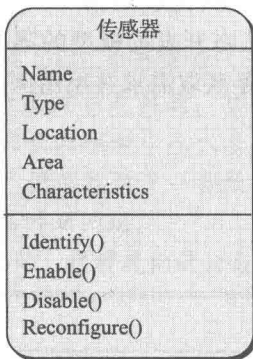
图 7-4 Sensor 类图
