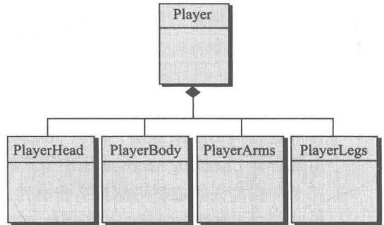
图 9-4 复合聚合类
