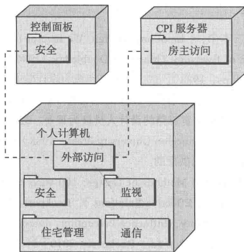
图 11-7 UML 部署图
