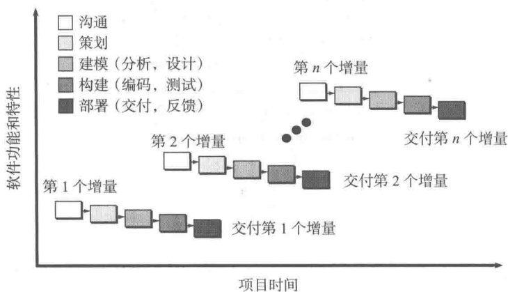
图 4-3 增量模型
