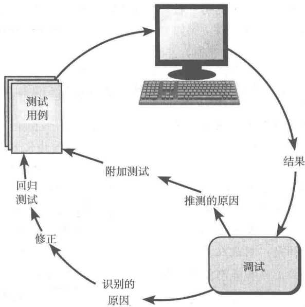
图 17-7 调试过程
